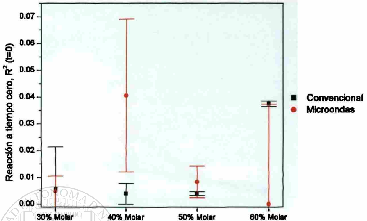
Figura 33. Contenido inicial de alúmina en la mezcla. Cantidad de espinel reaccionado a tiempo cero para cada curva cinética. Espinel reaccionado al momento en que se alcanzan los 1200°C.
