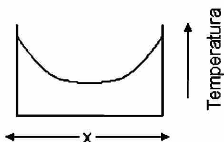
Figura 10. Comparación de perfiles térmicos en el calentamiento volumétrico y el calentamiento por conducción térmica.
