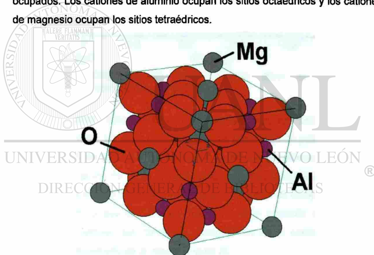
Figura 3. Celda unitaria del espinel alúmina-magnesia.
