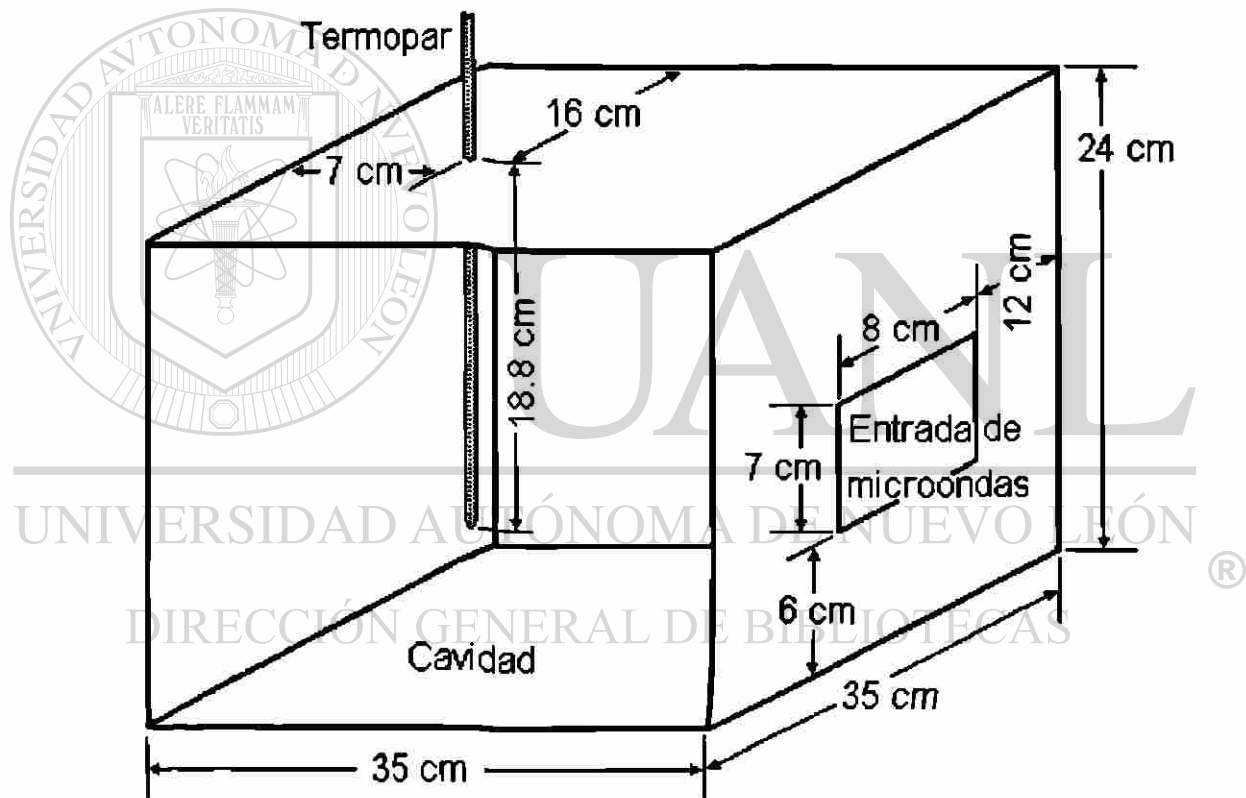
Figura 18. Esquema del horno de microondas y posición del termopar en la cavidad.
