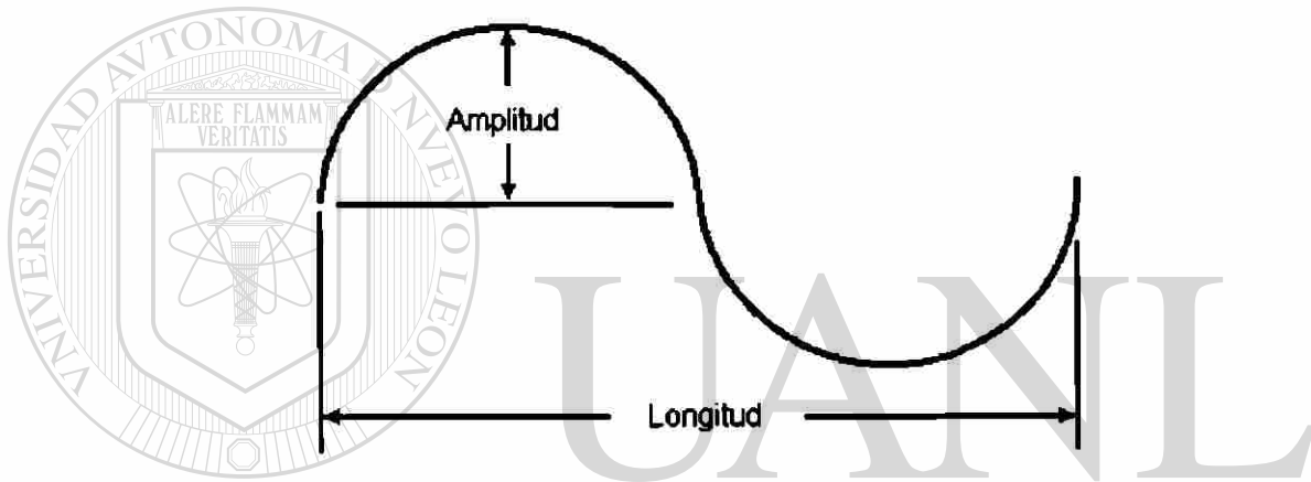
Figura 7. Representación de una onda cambiante en el tiempo.
