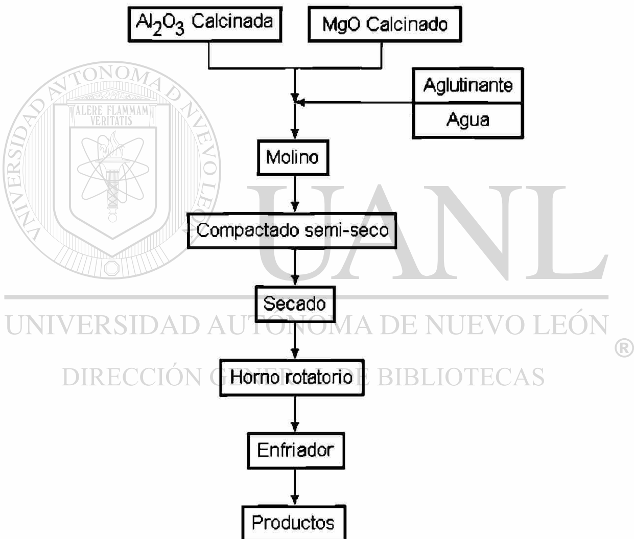
Figura 5. Producción del espinel con el uso de hornos rotatorios [27].
