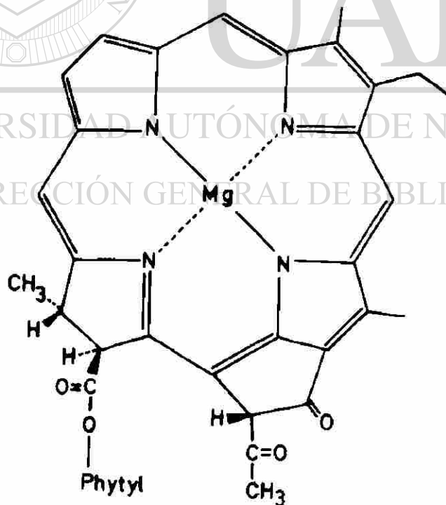
Fig. 1.- \alpha -Clorofila
