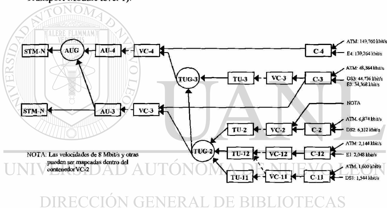
Figura 4.8 Estructura de multiplexión SDH
