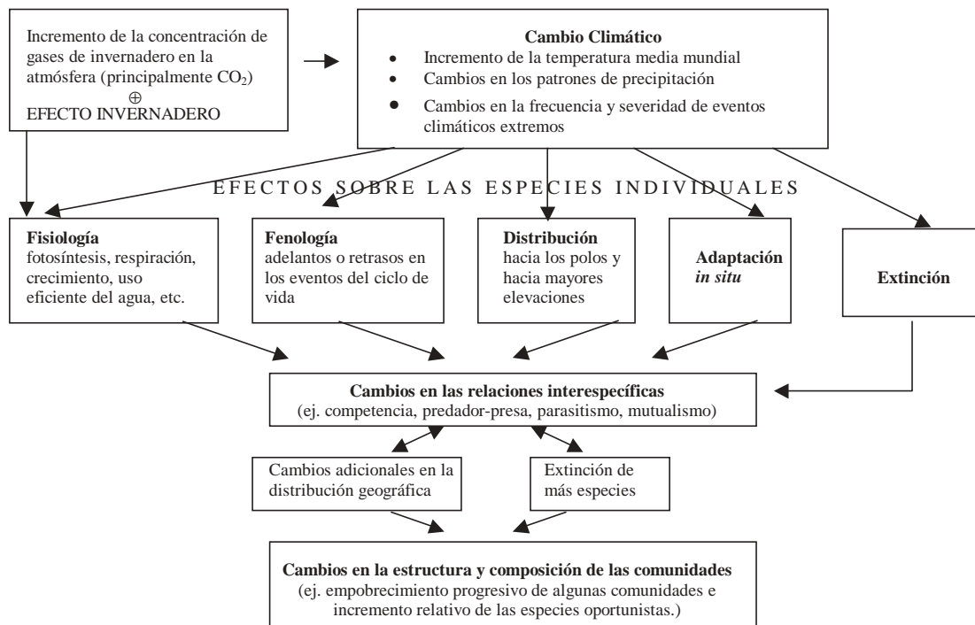
Fig.3. Vías potenciales del cambio en las comunidades y de la extinción de especies por efecto del incremento de gases de invernadero en la atmósfera. El aumento en la concentración de \text{CO}_2 en la atmósfera afecta algunos procesos fisiológicos de manera directa, y de manera indirecta a través de los efectos del cambio climático. La extinción de especies también puede presentarse como resultado directo del cambio climático o como consecuencia secundaria por los efectos del cambio climático sobre las relaciones inter- específicas. (Fuente: Adaptación de Hughes, 2000 1 ).
