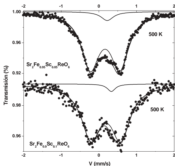
Fig. 4. Espectros Mössbauer experimental y ajuste de \text{Sr}_2\text{Fe}_{0.95}\text{Sc}_{0.05}\text{ReO}_6 y \text{Sr}_2\text{Fe}_{0.9}\text{Sc}_{0.1}\text{ReO}_6 obtenidos en la región paramagnética.
