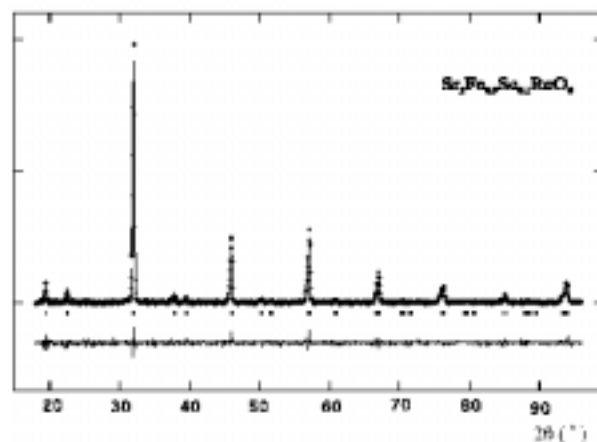
Fig. 1. Difractogramas de rayos X y ajuste para \text{Sr}_2\text{Fe}_{0.9}\text{Sc}_{0.1}\text{ReO}_6 rómbico Immm.
