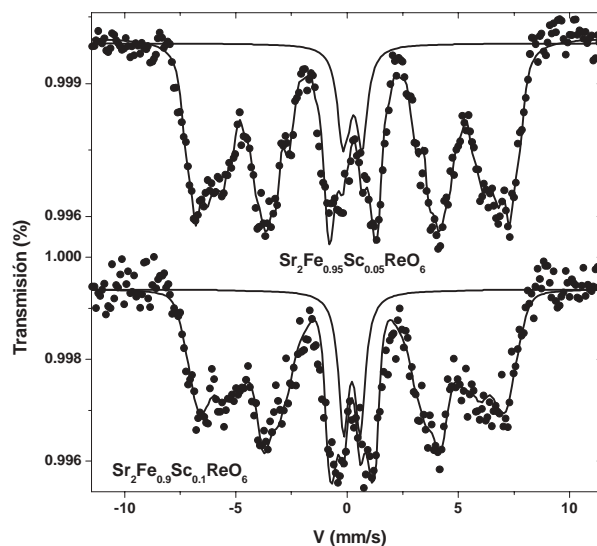
Fig. 5. Espectros Mössbauer para los compuestos \text{Sr}_2\text{Fe}_{0.95}\text{Sc}_{0.05}\text{ReO}_6 y \text{Sr}_2\text{Fe}_{0.9}\text{Sc}_{0.1}\text{ReO}_6 a temperatura ambiente.
