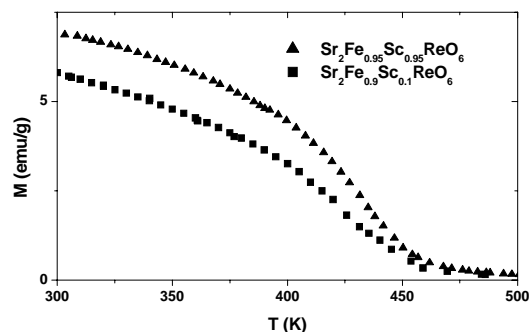
Fig. 2. Medidas de imanación para los compuestos estudiados bajo un campo aplicado de 0.5 Teslas.
