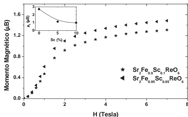
Fig. 3. Dependencia del momento magnético por fórmula unidad en función del campo aplicado a 10 K para el sistema \text{Sr}_2\text{Fe}_{1-x}\text{Sc}_x\text{ReO}_6
