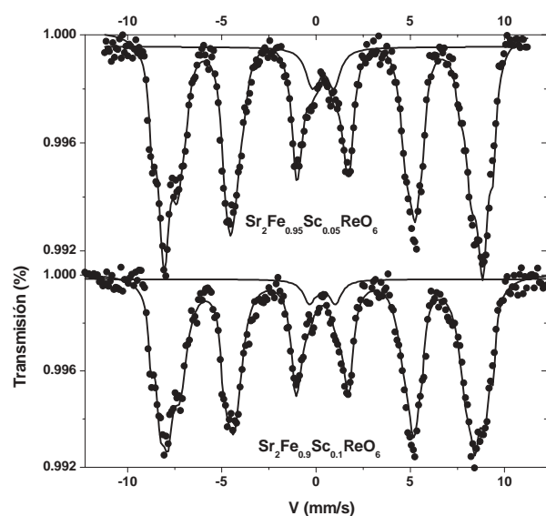
Fig. 6. Espectros Mössbauer para los compuestos \text{Sr}_2\text{Fe}_{0.95}\text{Sc}_{0.05}\text{ReO}_6 y \text{Sr}_2\text{Fe}_{0.9}\text{Sc}_{0.1}\text{ReO}_6 magnéticamente ordenados a 77 K.
