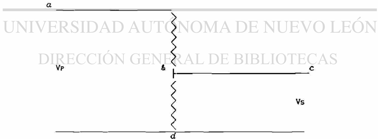
Fig. 5.2 Conexión como autotransformador.
