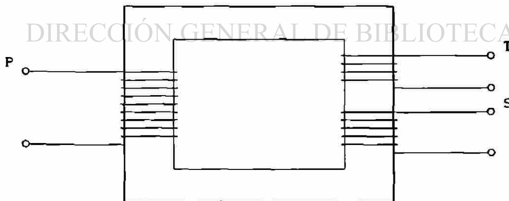
Fig. 3.14 Transformador monofásico de tres devanados.
