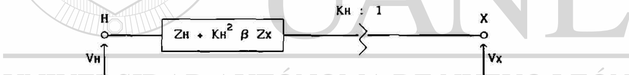
Fig. 3.5 Transformador con impedancias reflejadas al lado de alta.
