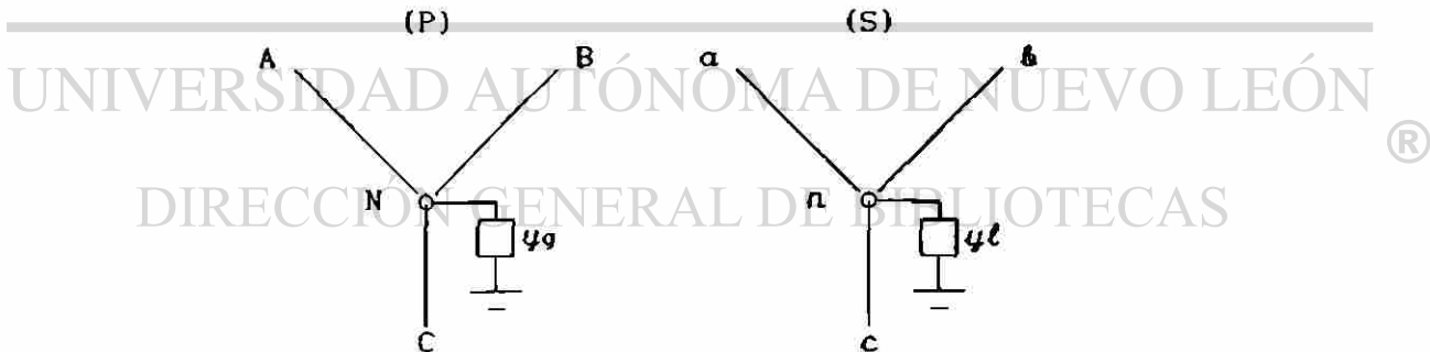
Fig. 4.26 Representación de la conexión trifásica.
