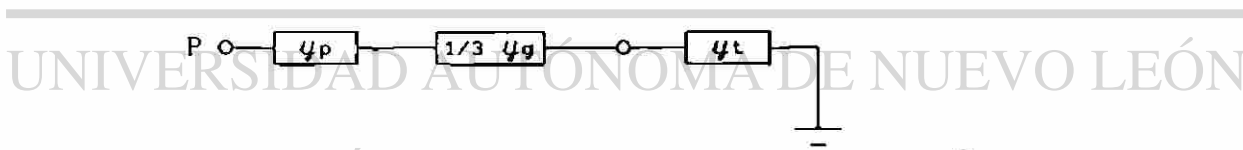
Fig. 4.59 Circuito de secuencia cero.
