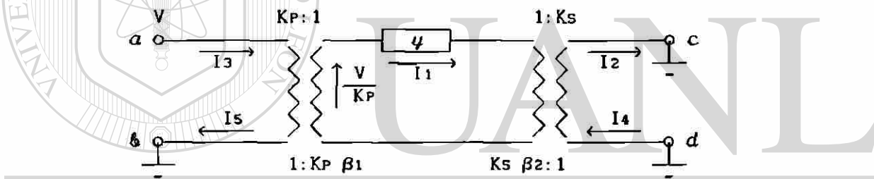
Fig. 3.12 Circuito generalizado de un transformador monofásico de dos devanados.
