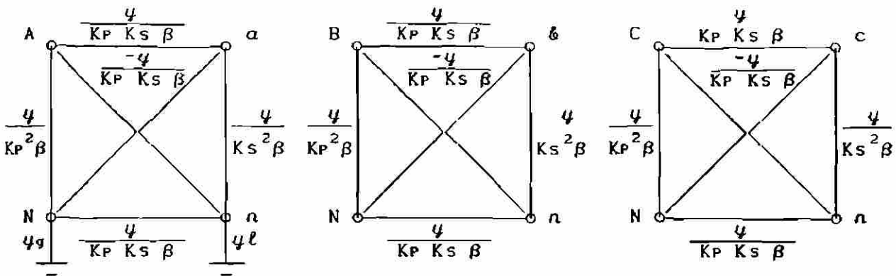
Fig. 4.27 Circuito equivalente de la conexión trifásica.
