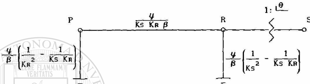
Fig. 4.90 Circuito generalizado de secuencia positiva.
