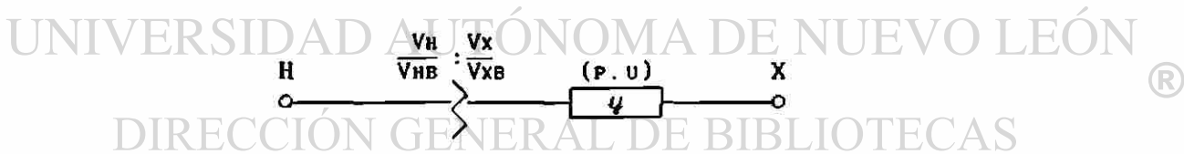
Fig. 3.2 Transformador con magnitudes y parámetro en por unidad.
