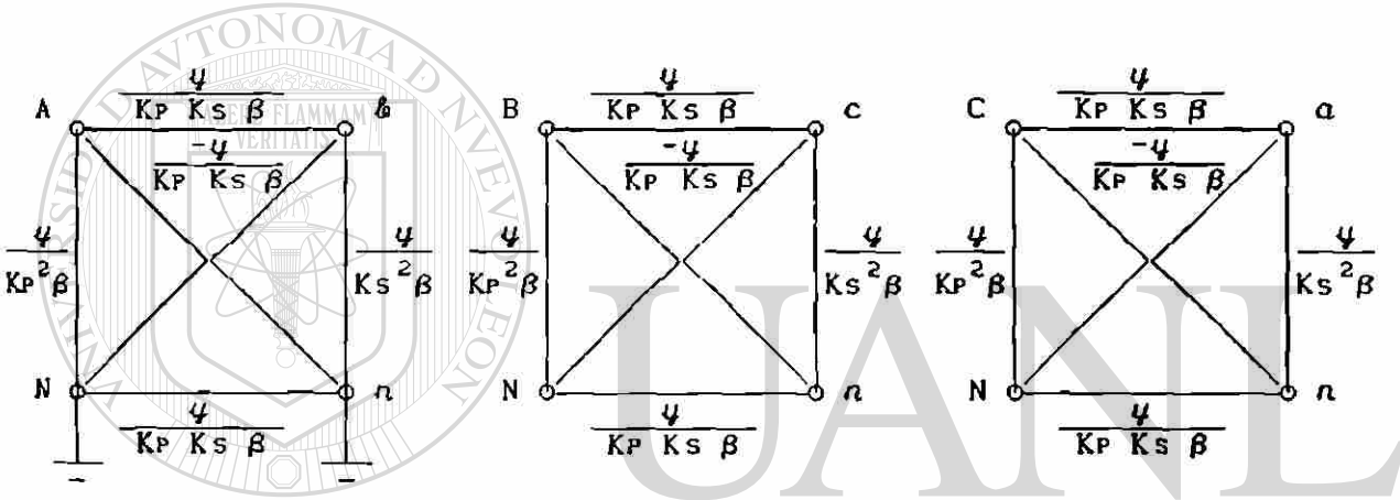
Fig. 4.38 Circuito equivalente de la conexión trifásica.
