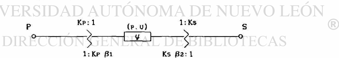
Fig. 3.11 Transformador monofásico con relación de transformación en por unidad.
