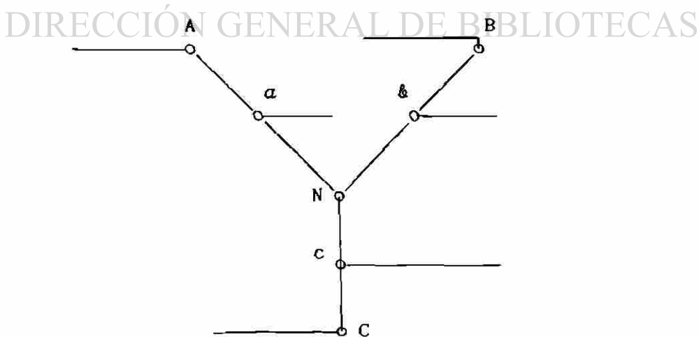
Fig. 6.2 Representación de un banco trifásico de autotransformadores monofásicos.
