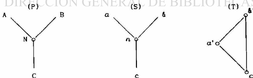
Fig. 4.55 Representación de un arreglo trifásico.
