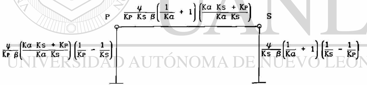
Fig. 6.7 Circuito generalizado de secuencia positiva.
