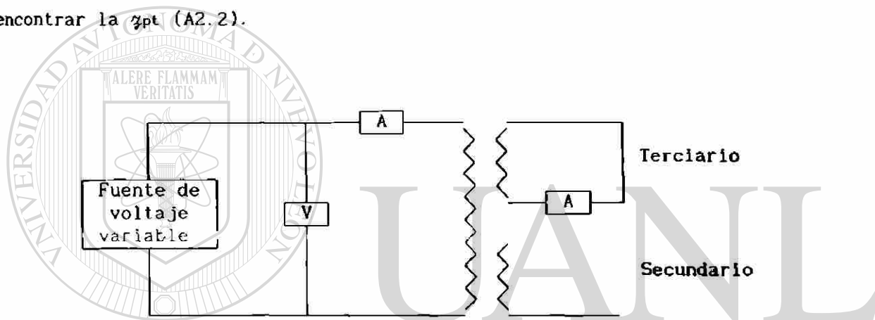
Fig. A2.2 Conexión para obtener z_{pt} .
