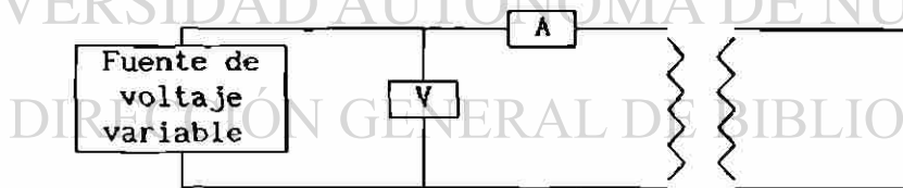
Fig. A1.1 Conexión para prueba de cortocircuito.
