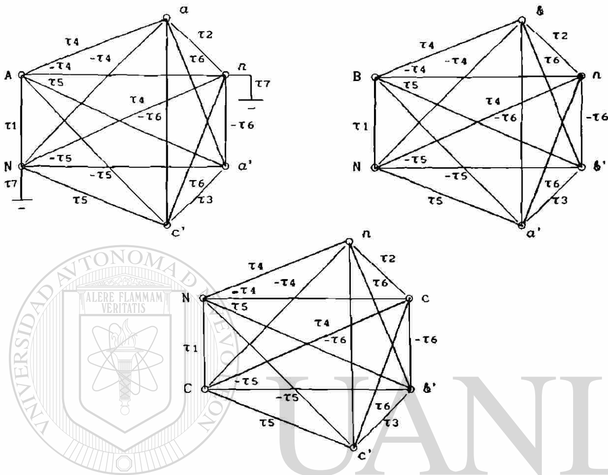
Fig. 4.66 Circuito equivalente de la conexión trifásica.
