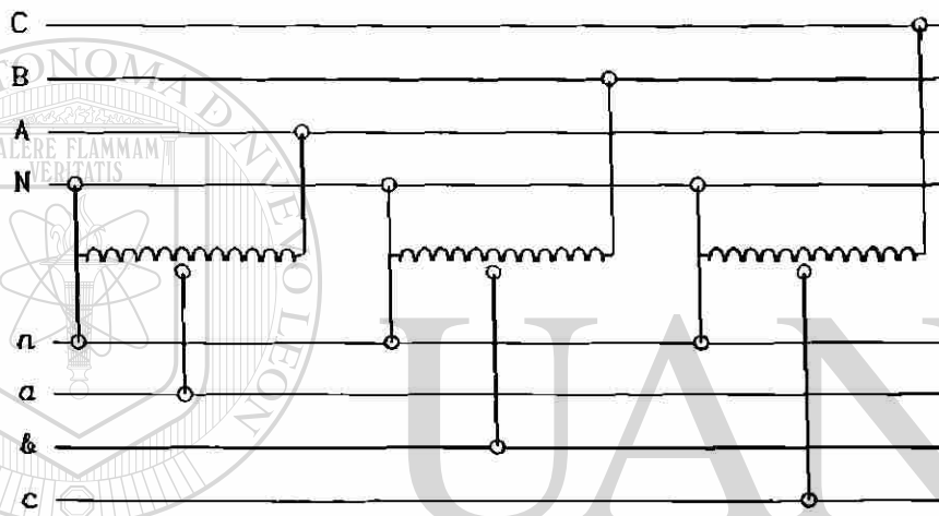
Fig. 6.1 Banco trifásico de autotransformadores monofásicos.
