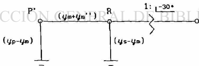
Fig. 4.81 Circuito reducido de secuencia negativa.
