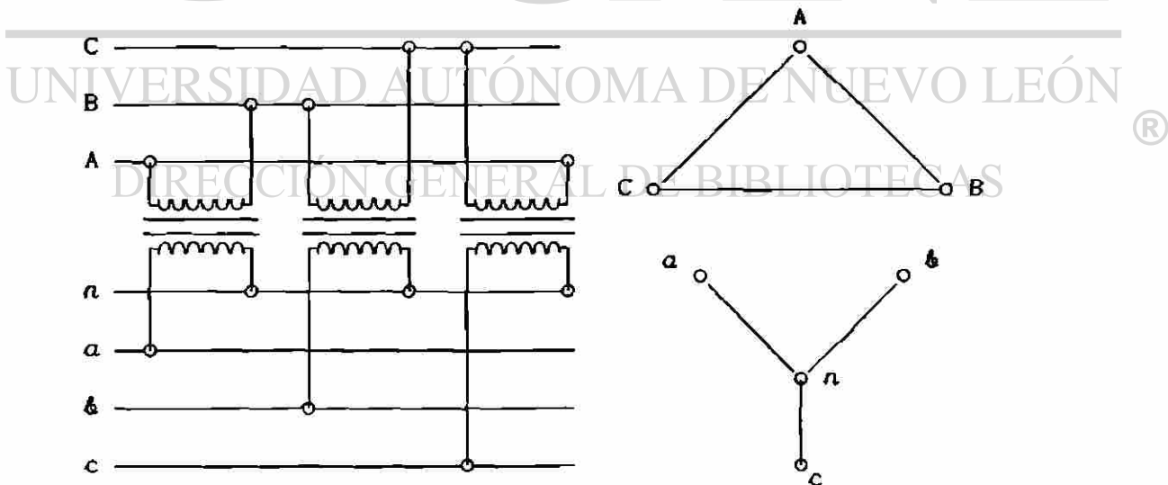
Fig. 4.1 Conexión trifásica de tres unidades monofásicas en \Delta -Y.
