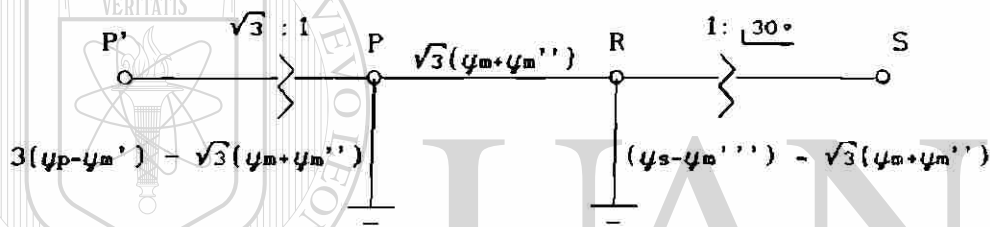
Fig. 4.78 Circuito de secuencia positiva con corrección en transformador ficticio.
