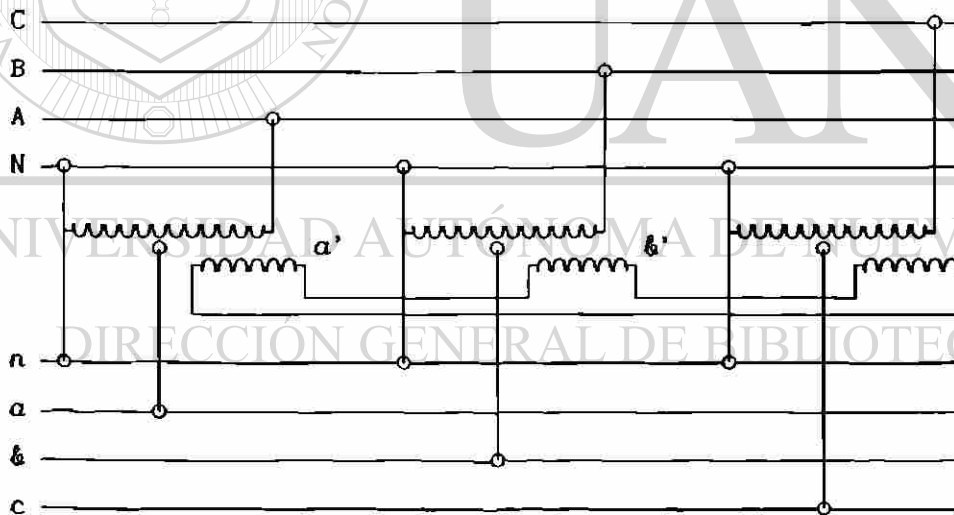
Fig. 6.9 Banco trifásico de autotransformadores monofásicos de tres devanados.
