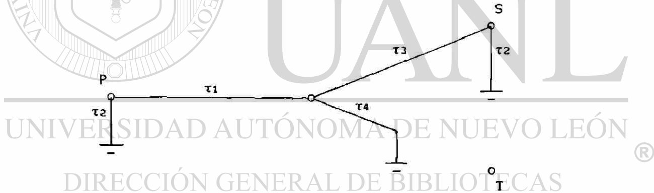
Fig. 4.68 Circuito generalizado en estrella de secuencia cero.
