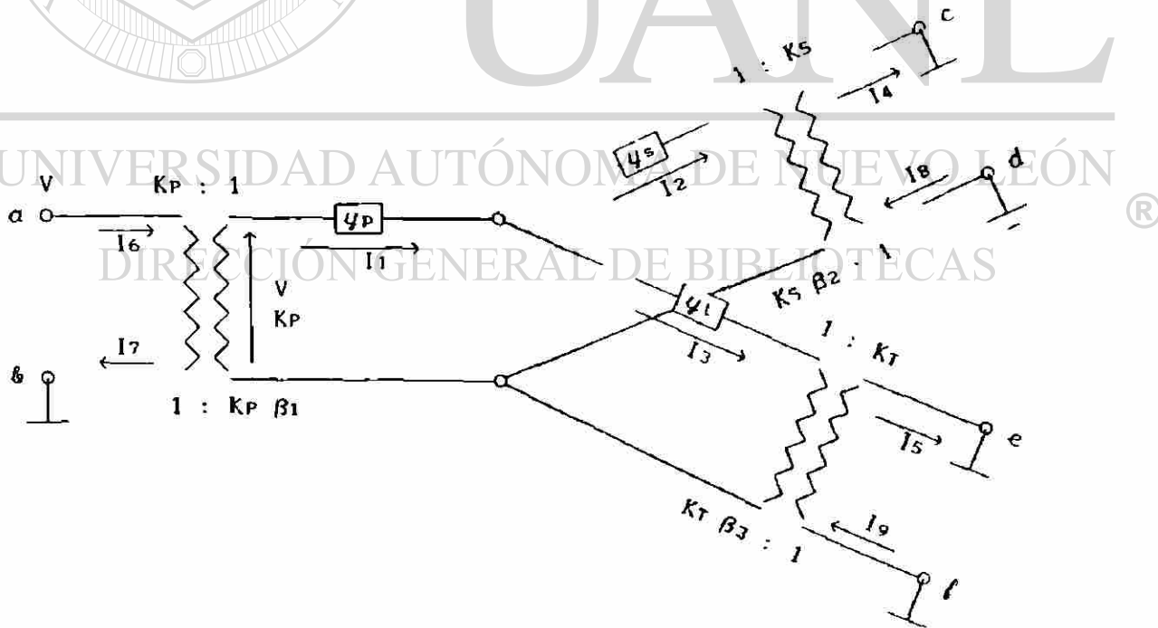
Fig. 3.17 Circuito generalizado de un transformador monofásico de tres devanados.
