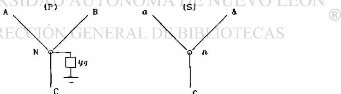
Fig. 4.32 Representación de la conexión trifásica.
