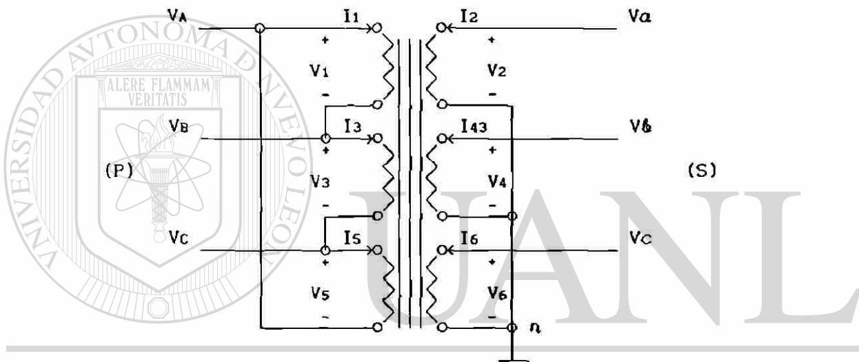
Fig. 4.75 Circuito de conexión trifásica.
