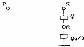
Fig. 4.19 Circuito de secuencia cero.
