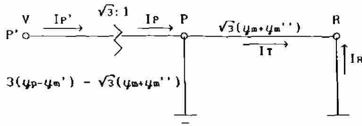
Fig. 4.78a Corrección parcial del circuito de secuencia positiva.
