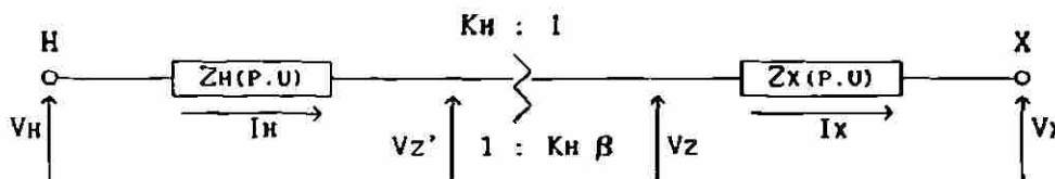
Fig. 3.4 Transformador con magnitudes y parámetros en por unidad.
