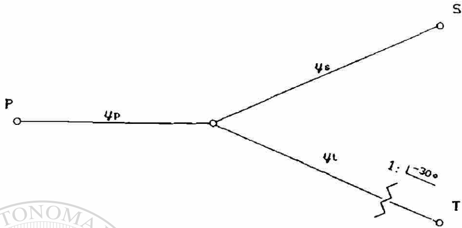
Fig. 4.64 Circuito de secuencia negativa simplificado.
