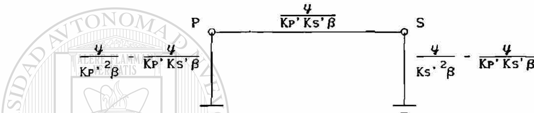
Fig. 4.47 Circuito generalizado de secuencia positiva.
