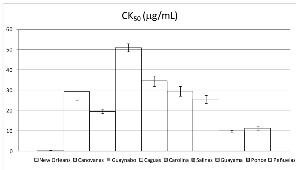
Fig.6. CK 50 e intervalos de confianza de adultos expuestos a permetrina.
