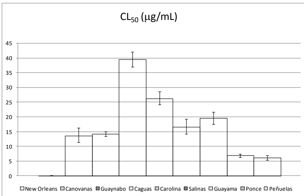
Fig.7. CL 50 e intervalos de confianza de adultos expuestos a permetrina.
