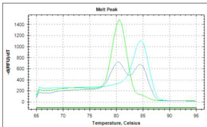
Fig. 4. Gráfica de Meltcurve, que muestra las curvas con sus temperaturas correspondientes: un pico a 80 °C, (Phe1534) (susceptibles), un pico a 85 °C (Cys1534) (resistentes) y ambos picos, 80°C y 85°C, heterocigotos
