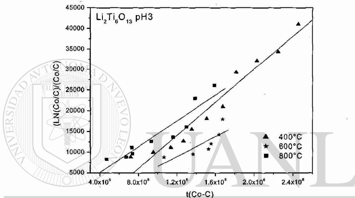
Fig. 4.7 Gráfico del modelo de Langmuir-Hiselwood en la degradación de 2,4 DNA con Li_2Ti_6O_{13} preparado a pH 3 y tratado a diferentes temps.
