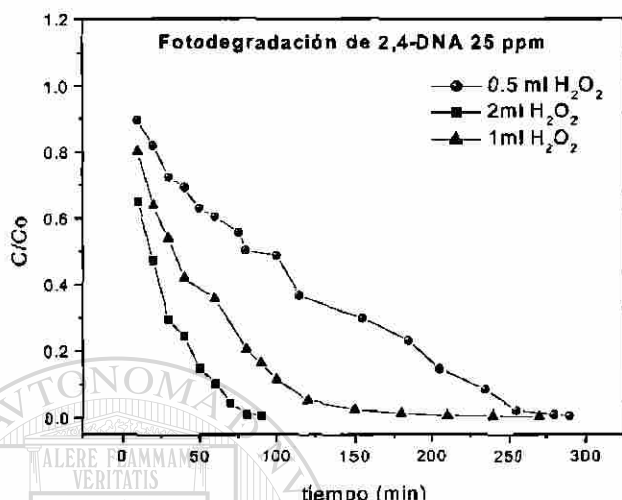
Fig. A-4 Comportamiento de la fotoactividad del sistema, a diferentes conc. de H 2 O 2 , \lambda = 254 nm
