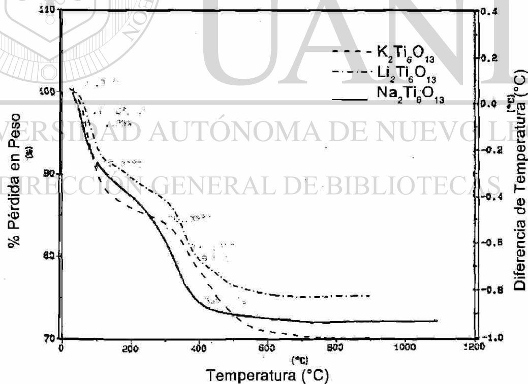
Fig. 4.67. Termograma de muestra fresca de hexatitanatos sintetizados a pH 9, atm N_2 .
