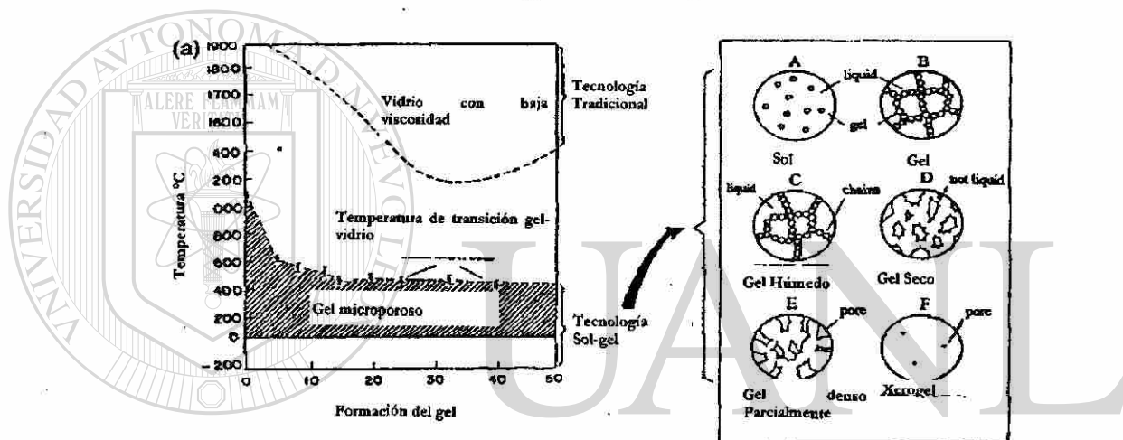
Fig. 2.3 Formación del gel con respecto de la temperatura
