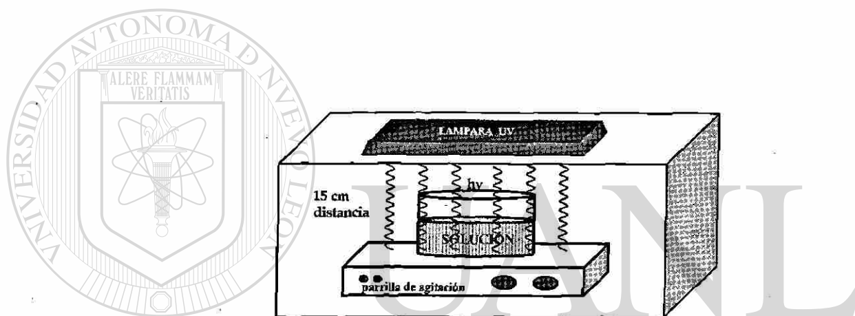
Figura 3.2 Sistema utilizado para la degradación fotocatalítica de la 2,4 DNA
