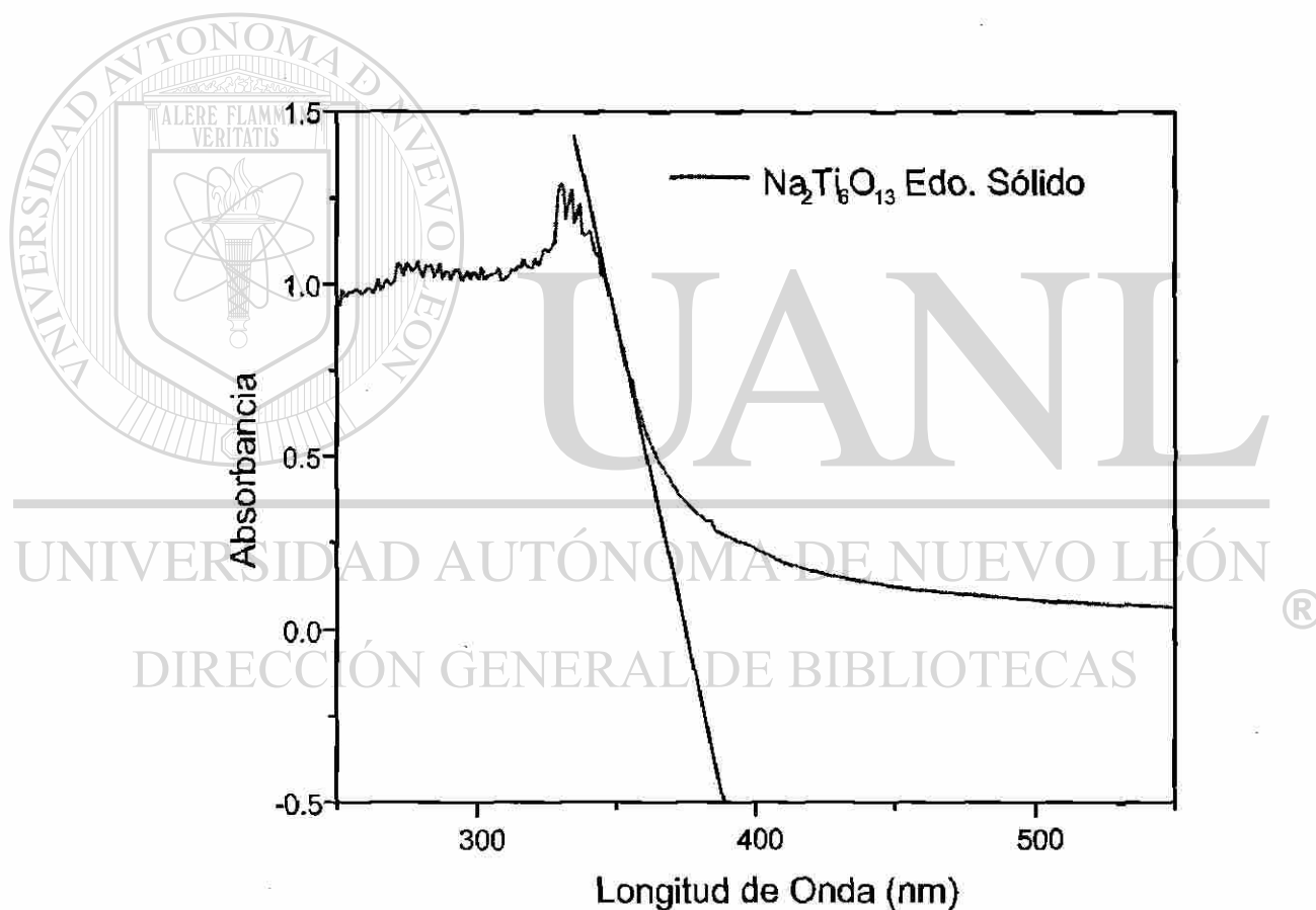
Fig. 4.16 Espectros UV-Vis de \text{Na}_2\text{Ti}_6\text{O}_{13} para el cálculo de la E_g , sintetizados por Estado Sólido.
