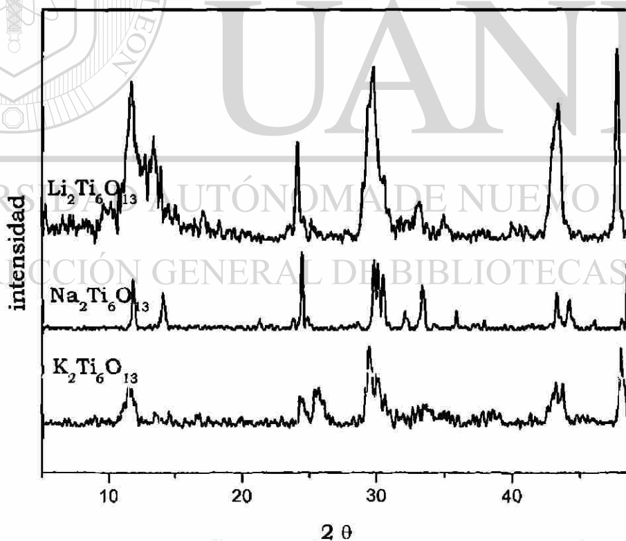
Fig. 4.66 Difractograma de hexatitanatos sintetizados via Sol-gel pH 9
