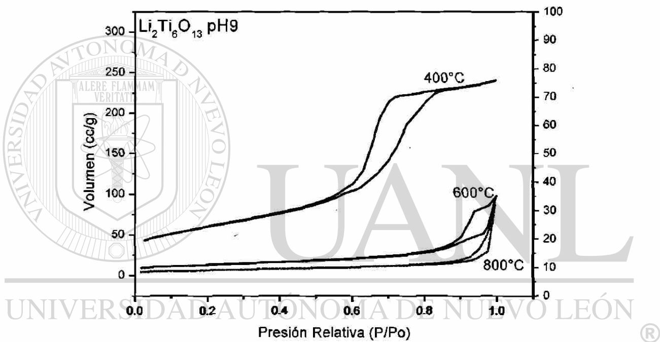
Fig. 4.12 Isothermas de adsorción y desorción de \text{Li}_2\text{Ti}_6\text{O}_{13} . Sol-gel pH 9 a diferentes temperaturas.
