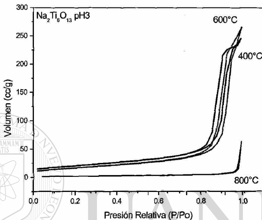
Fig. 4.24 Isothermas de adsorción y desorción de \text{Na}_{12}\text{Ti}_6\text{O}_{13} Sol-gel pH 3 a diferentes temperaturas.
