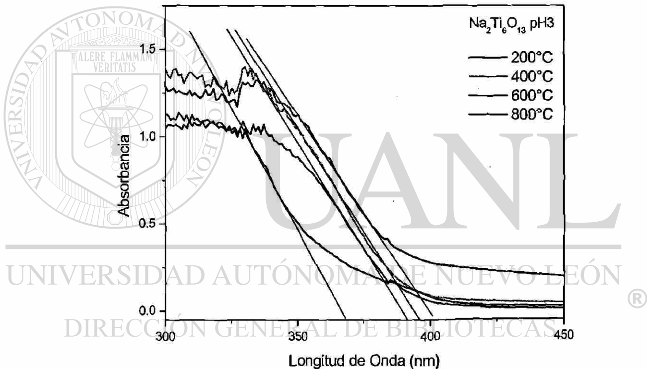
Fig. 4.23 Espectro UV-Vis de \text{Na}_2\text{Ti}_6\text{O}_{13} sintetizados por Sol-gel pH 3, para el cálculo de valores de E_g .
