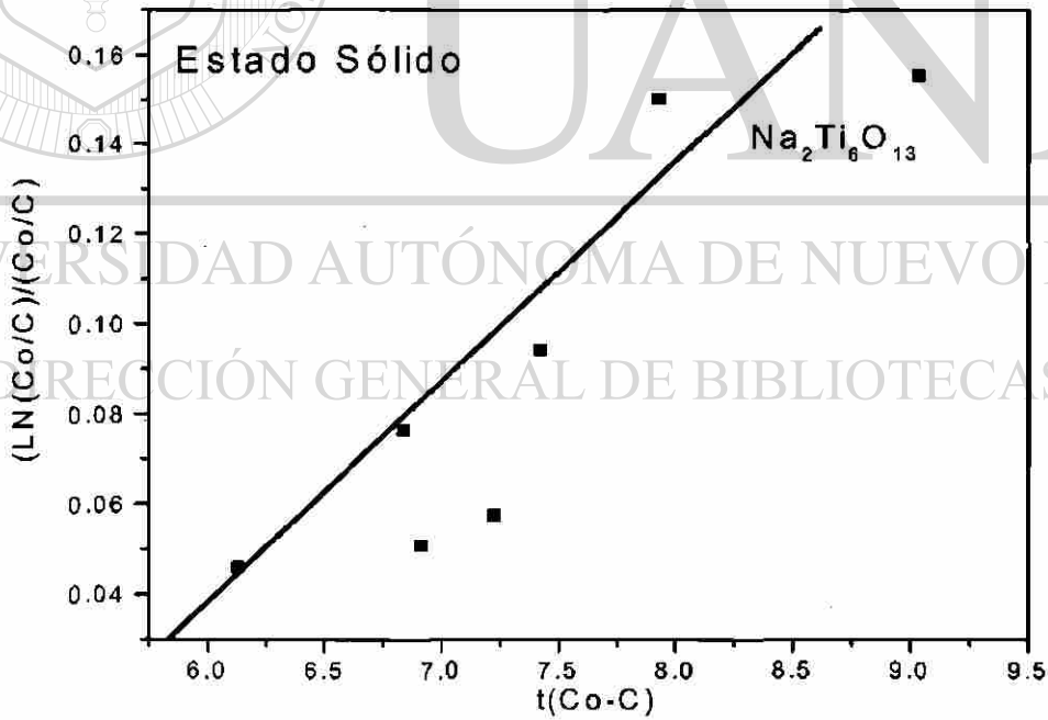
Fig. 4.19 Gráfico del modelo de Langmuir-Hiselow en la degradación de 2,4 DNA con \text{Na}_2\text{Ti}_6\text{O}_{13} por Estado Sólido.
