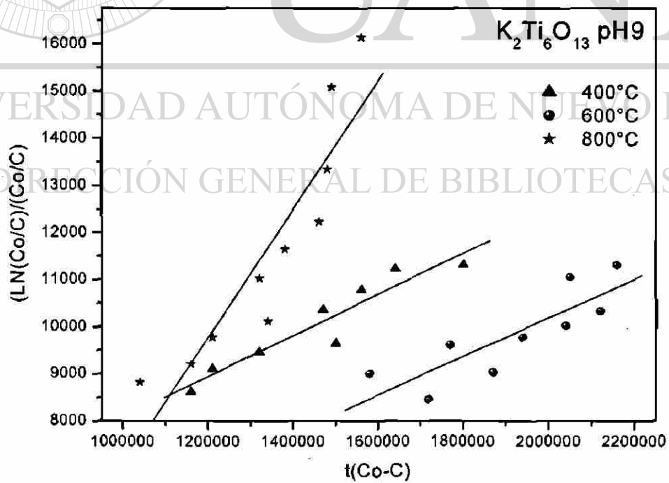
Fig. 4.52 Gráfico del modelo de Langmuir-Hiselwood en la degradación de 2,4 DNA con K_2Ti_6O_{13} preparado a pH 9 y tratado a diferentes temps.
