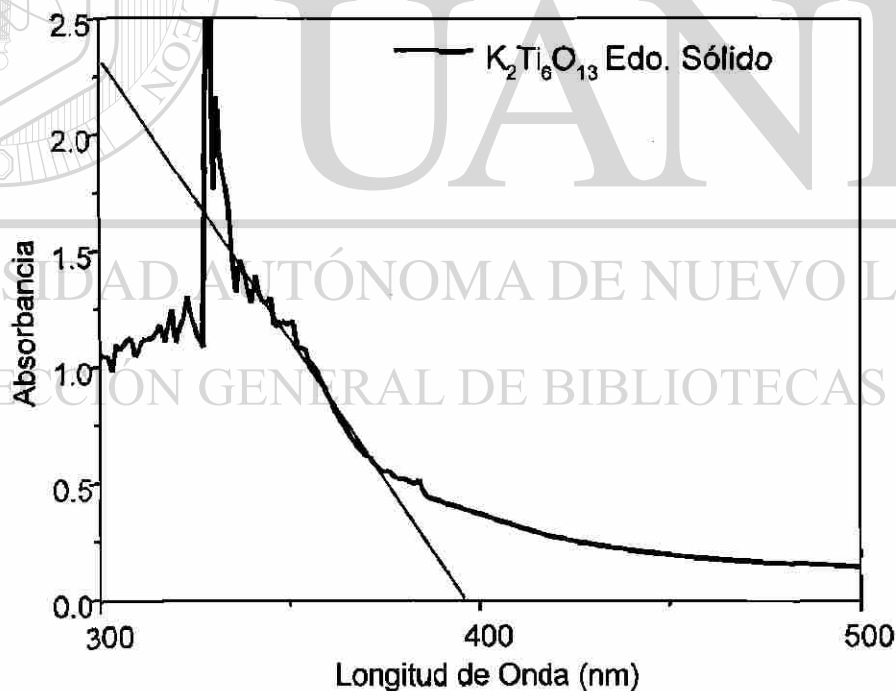
Fig. 4.35 Espectros UV-Vis de K_2Ti_6O_{13} para el cálculo de la E_g sintetizados por Estado Sólido.
