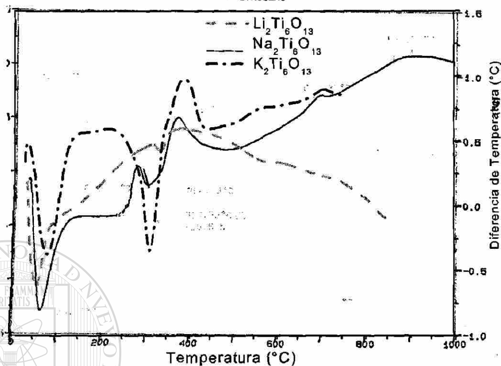
Fig. 4.60 Termograma de muestra fresca de los hexatitanatos sintetizado a \text{pH } 3.5^\circ\text{C}/\text{min. atm } \text{N}_2 .
