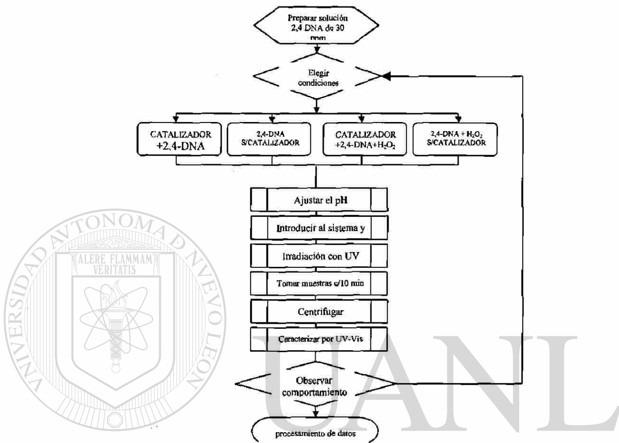
Fig. 3.3 Diagrama para el estudio de la degradación fotocatalítica de 2,4-DNA
