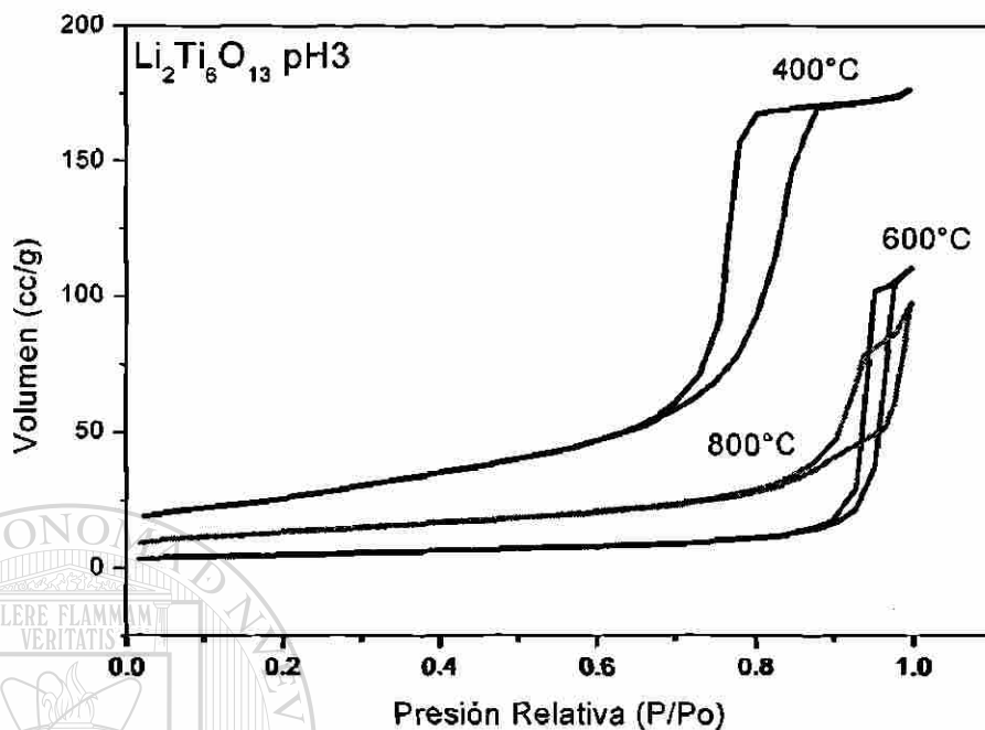
Fig. 4.5 Isothermas de adsorción y desorción de \text{Li}_2\text{Ti}_6\text{O}_{13} vía Sol-gel a pH 3, a diferentes temperaturas.
