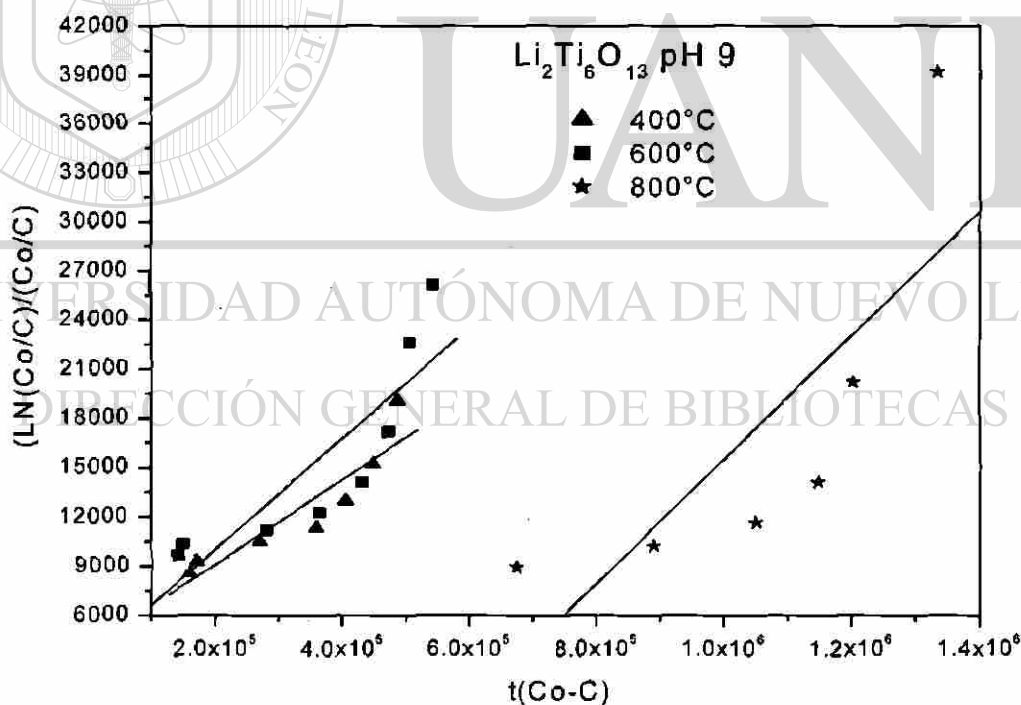
Fig. 4.14 Gráfico del modelo de Langmuir-Hinshelwood en la degradación de 2,4-DNA con \text{Li}_2\text{Ti}_6\text{O}_{13} preparado a pH 9 y tratado a diferentes temps.
