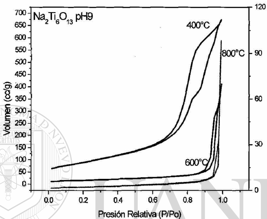
Fig. 4.31 Gráfico de isotermas de muestras calcinadas a diferentes temperaturas del compuesto \text{Na}_2\text{Ti}_6\text{O}_{13} pH 9.
