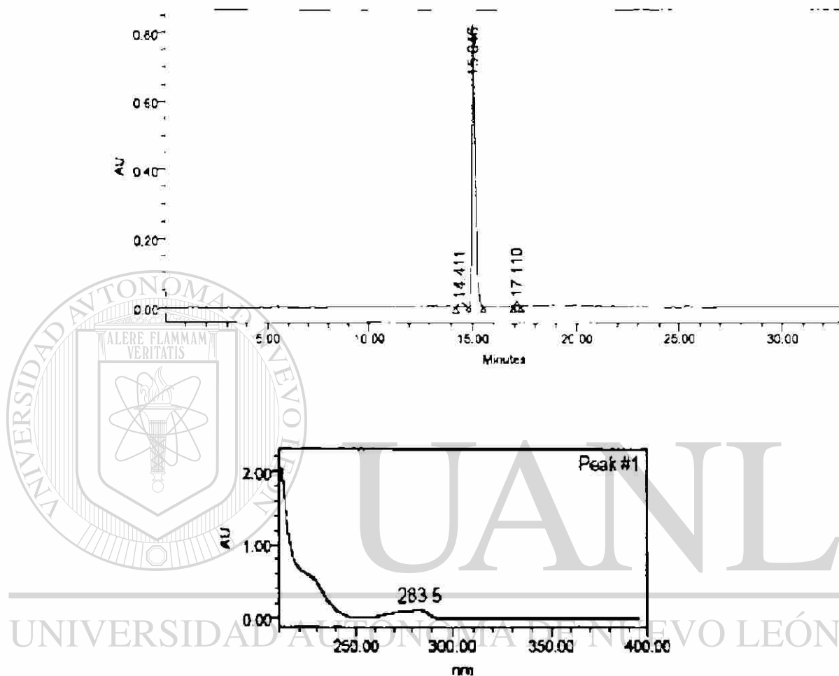
Figura 12. Cromatograma y Espectro UV-Vis del compuesto 3 (contenido en el tubo 73) obtenidos usando como Fase Estacionaria una columna Symmetry C18 5 \mu m, 3.9 X 150 mm No. Serie WAT 046980 y como Fase Móvil: MeOH:agua 70:30, con las condiciones descritas en 3.2.5.1.
