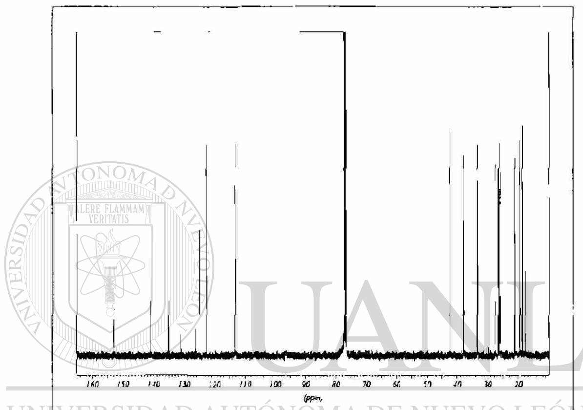
Figura 23. Espectro de ^{13}\text{C} RMN del compuesto 4 aislado de raíz de L.® frutescens DIRECCIÓN GENERAL DE BIBLIOTECAS
