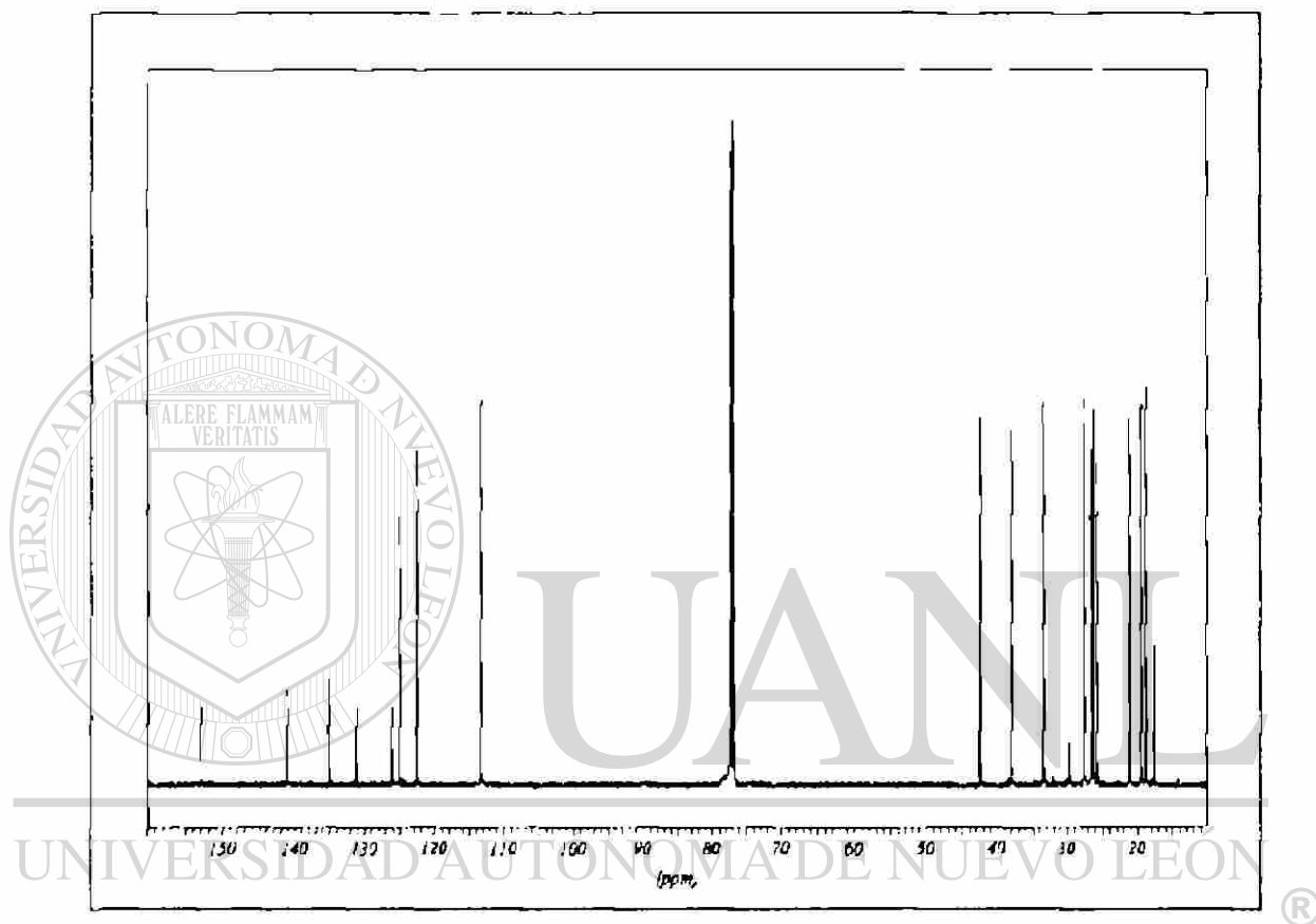
Figura 22. Espectro de ^{13}\text{C} RMN del compuesto 3 aislado de raíz de L. frutescens .
