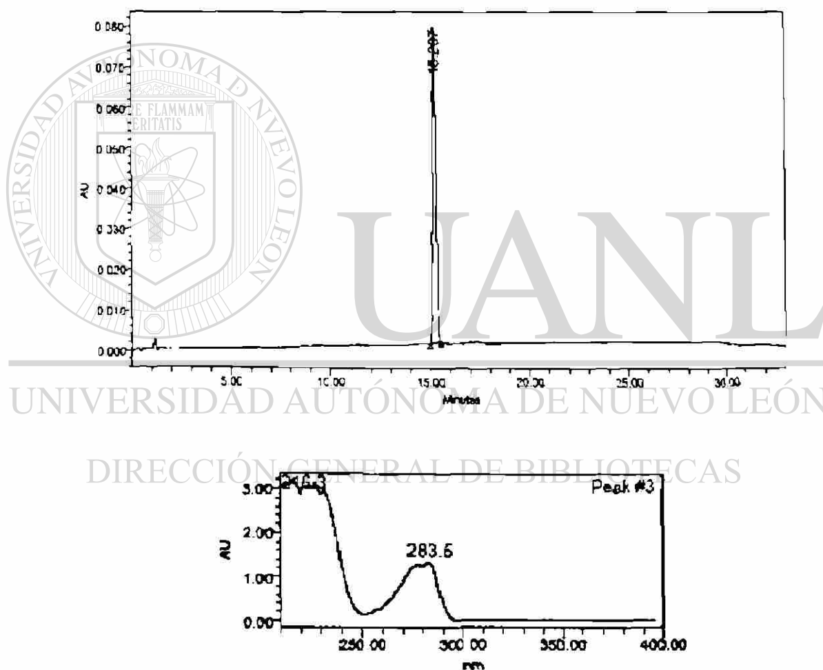
Figura 13. Cromatograma y Espectro UV-Vis del compuesto 4 usando como Fase Estacionaria una columna Symmetry C18 5 \mu m, 3.9 X 150 mm No. Serie WAT 046980 y como Fase Móvil: MeOH:agua 70:30, con las condiciones descritas en 3.2.5.1.
