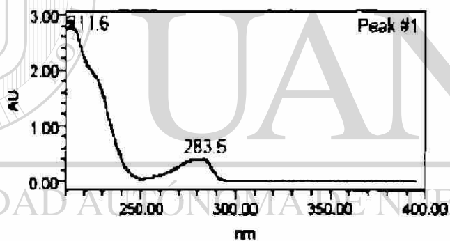
Figura 11. Cromatograma y Espectro UV-Vis del compuesto 3 (contenido en el tubo 70) obtenidos usando como Fase Estacionaria una columna Symmetry C18 5 \mu m, 3.9 X 150 mm No. Serie WAT 046980 y como Fase Móvil: MeOH:agua 70:30, con las condiciones descritas en 3.2.5.1.
