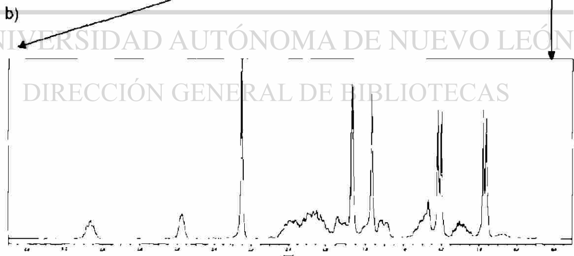
Figura 20. a) Espectro de ^1\text{H} RMN del compuesto 3 aislado de raíz de L. frutescens , b) Ampliación de la zona del Espectro ^1\text{H} RMN del compuesto 3 entre 0.5 y 3.5 ppm.
