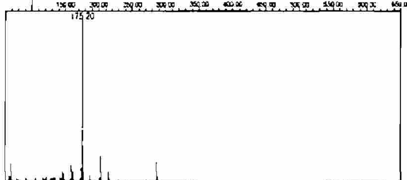
Figura 6. Cromatograma de la fracción VLC 20:1 obtenido con Columna Polarity dC18 3 \mu m 2.1 X 50 cm como Fase Estacionaria y ácido fórmico 0.1% en agua y ácido fórmico 0.1% en ACN como Fase Móvil, con las condiciones descritas en 3.2.4.4 y detector a) DAD y b) EM.
