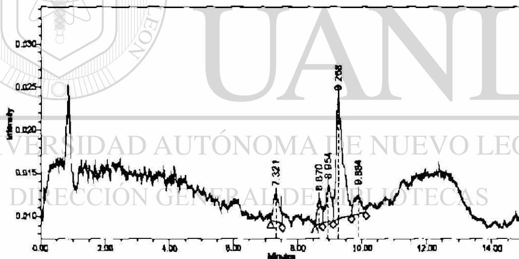
Figura 8. Cromatograma de la Fracción VLC 10:1 obtenido con Columna Polarity \mu\text{C18 } 3 \mu\text{m } 2.1 \times 50 \text{ cm} como Fase Estacionaria y ácido fórmico 0.1% en agua y ácido fórmico 0.1% en ACN como Fase Móvil, con las condiciones descritas en 3.2.4.4 y detector a) DAD y b) EM.
