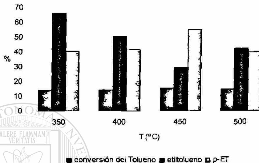
Figura 15. Dependencia de la conversión del tolueno, la producción del grupo de etiltolueno y la selectividad del isómero del p -ET, con respecto a la temperatura sobre la zeolita natural clinoptilolita (ZCM).
