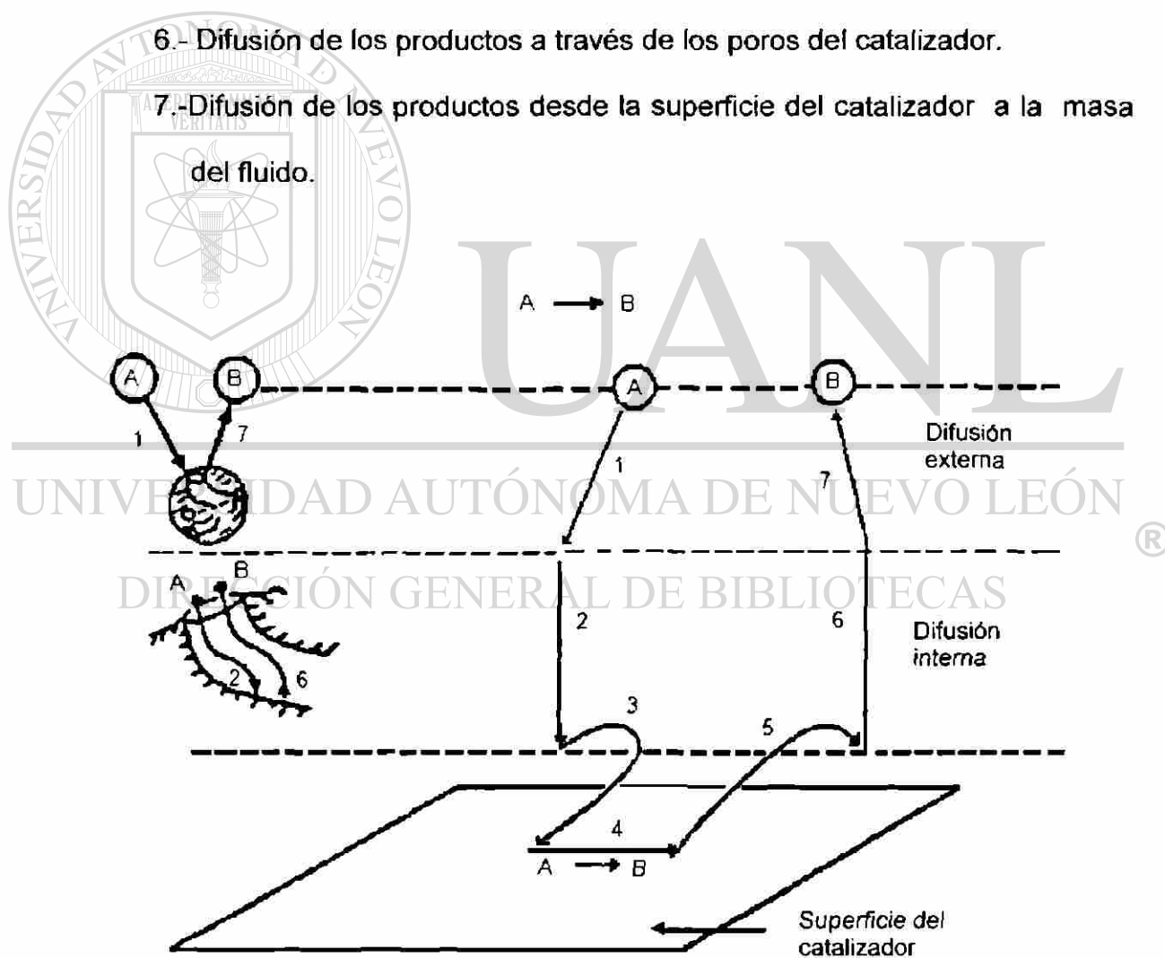
Figura 1. Representación de las reacciones catalíticas en la superficie del catalizador.
