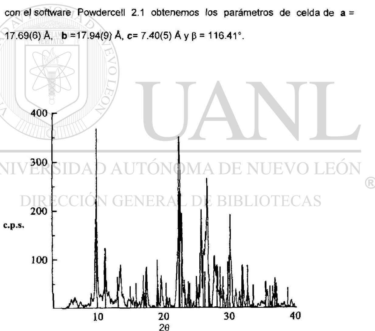
Figura 9. Patrón de difracción de rayos x de la clinoptilofita natural.
