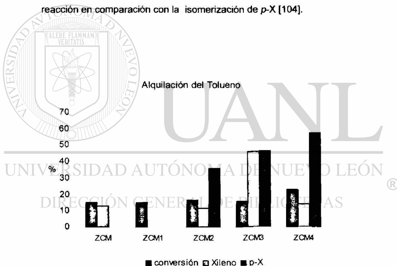
Figura 22. Relación de la conversión del tolueno, la producción del grupo xileno X y la selectividad del isómero para-xileno p -X, con respecto a los catalizadores.
