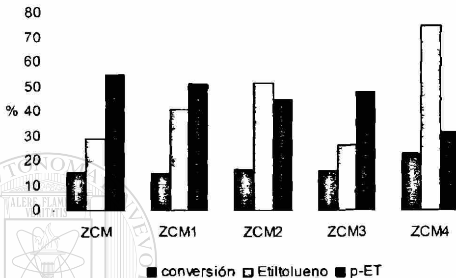
Figura 23. Comportamiento de la selectividad del grupo de ET, la selectividad del isómero p -ET con respecto a los diferentes catalizadores
