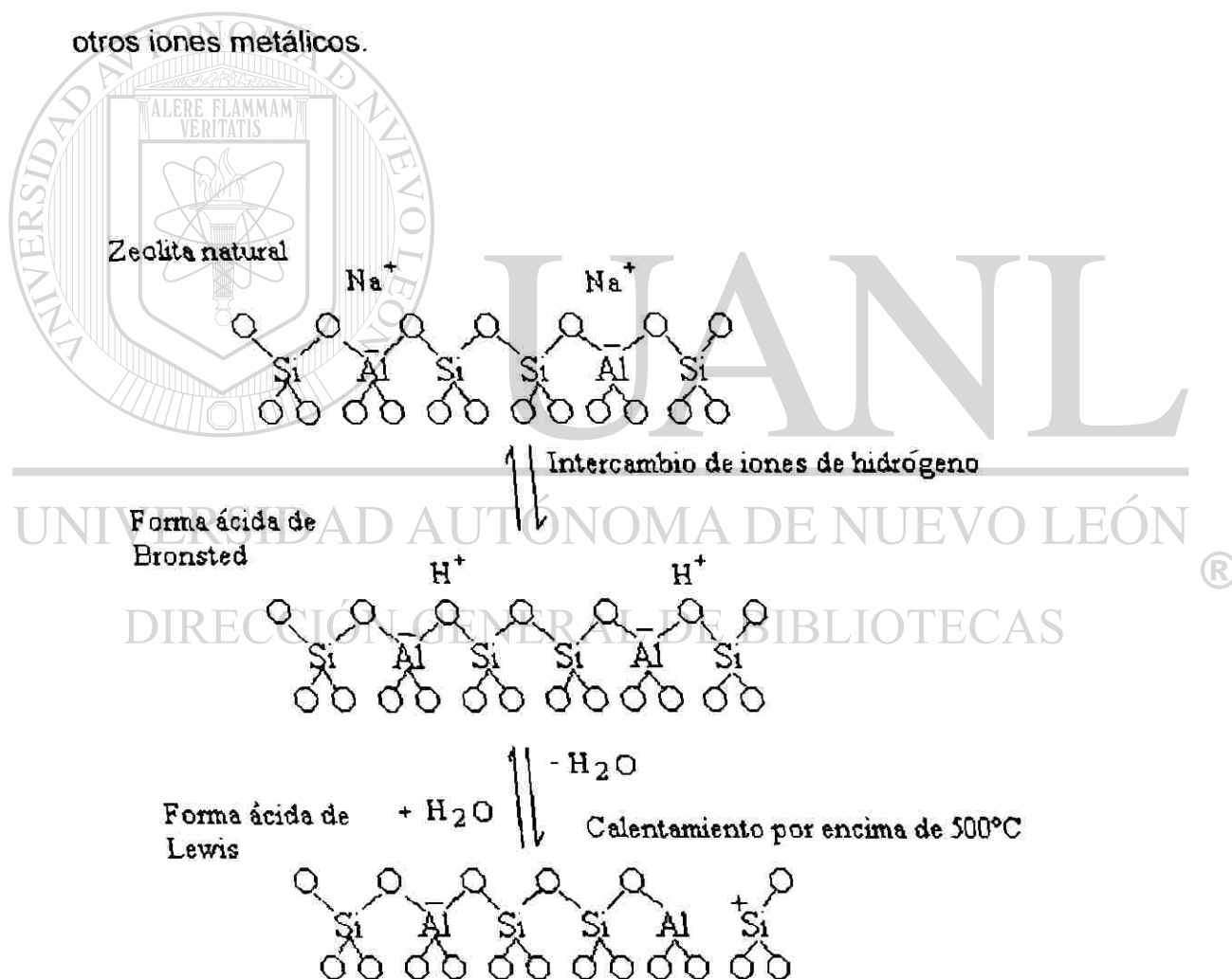
Figura 4. Esquema para la generación de centros ácidos de Bronsted y Lewis en la zeolita.
