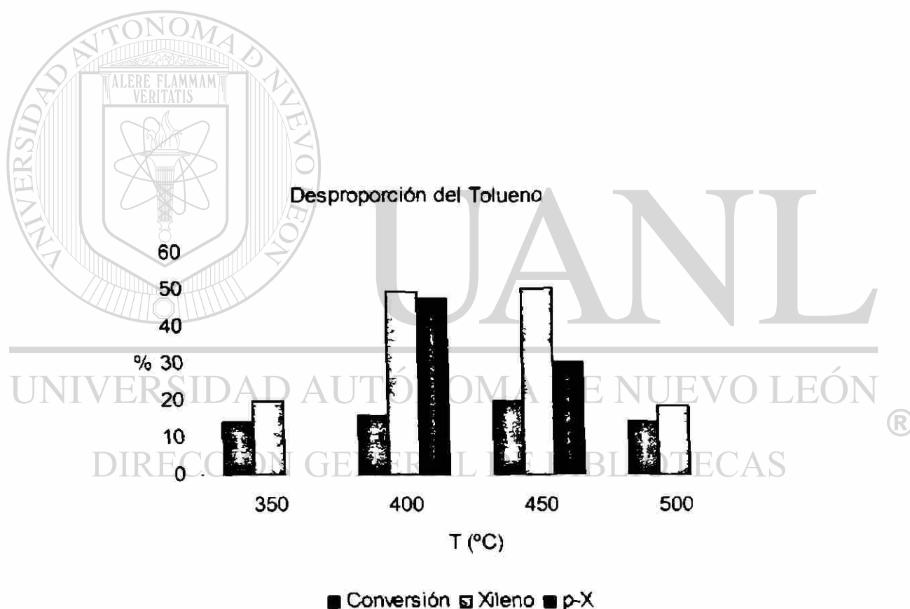
Figura 12. Se presenta la conversión del tolueno, el contenido del grupo xileno y la selectividad del para-xileno en función de la temperatura sobre la zeolita natural clinoptilolita (ZCM).
