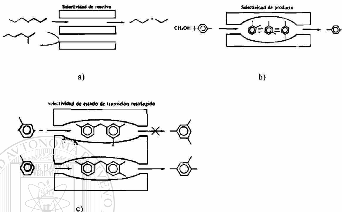
Figura 3. Catálisis selectiva de forma, a) catálisis selectiva de reactivo, b) catálisis selectiva de producto, c) catálisis selectiva de estado de transición.
