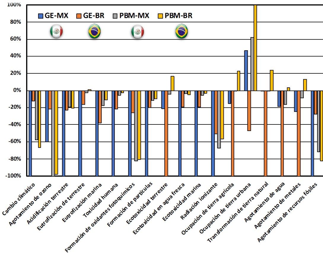
Figura 6.3. Resultados de impactos ambientales del ACV para los tres escenarios de estudio según el método ReCiPe Midpoint (H).
