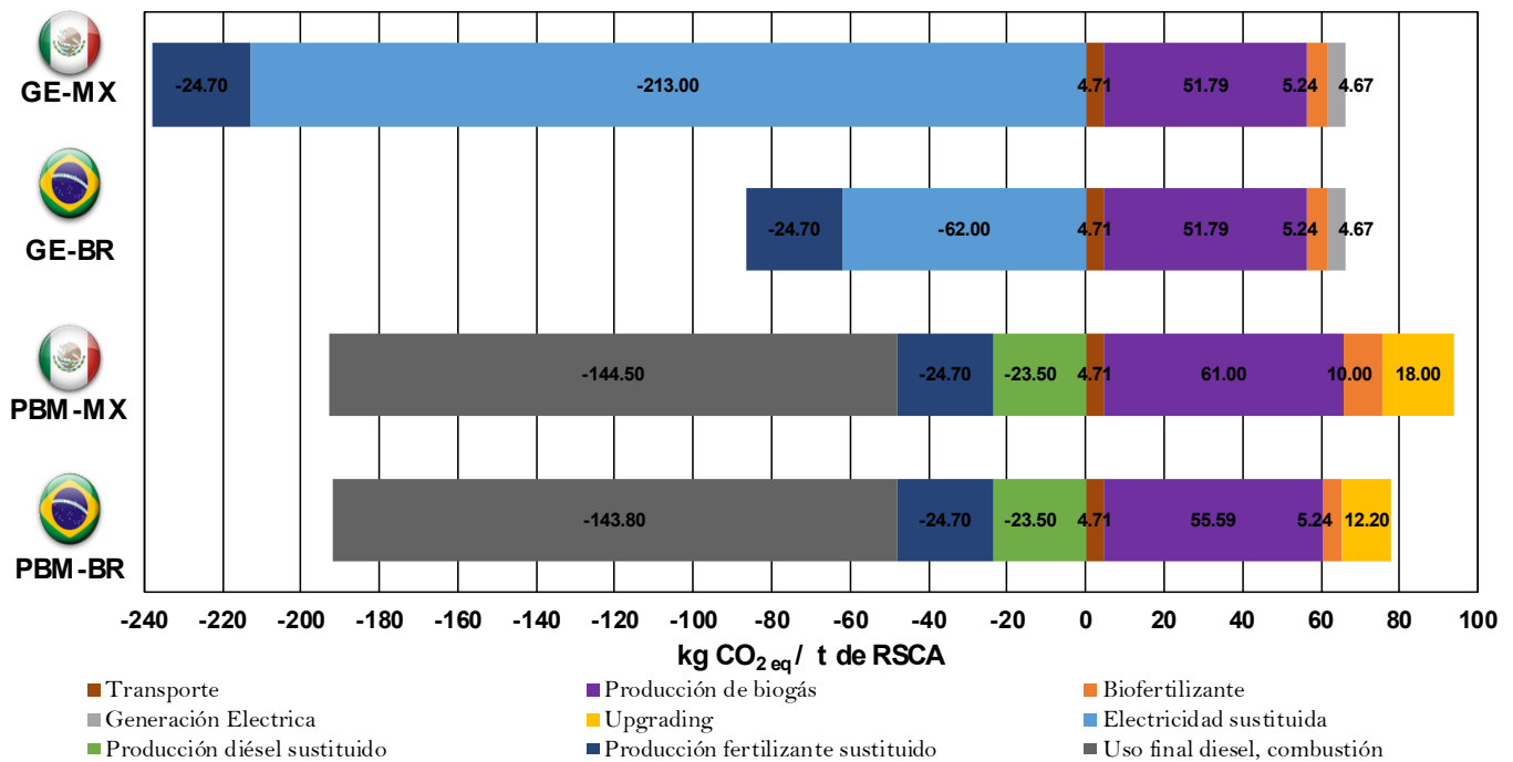
Figura 6.5. Análisis de puntos críticos en la categoría de impacto de cambio climático por los principales procesos de los cuatro escenarios. GE= Generación eléctrica; PBM= Producción de biometano; MX= México; BR= Brasil.
