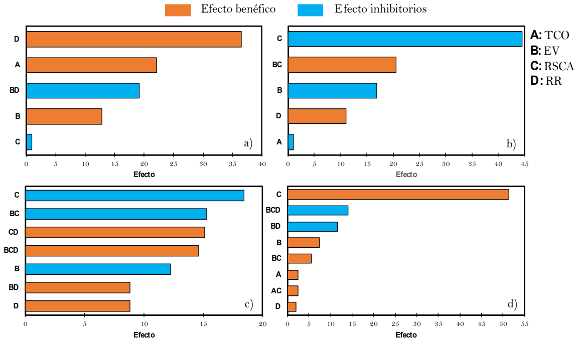
Figura 6.1. Diagrama de Pareto del diseño central compuesto con punto medio. a) Productividad de CH 4 , b) CH 4 /CO 2 , c) AGV/AB, d) ICoD.
