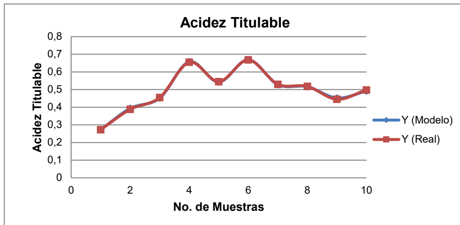
Figura 116. Modelo de predicción vs. valor real de la acidez titulable de la variedad Cabernet Sauvignon.
