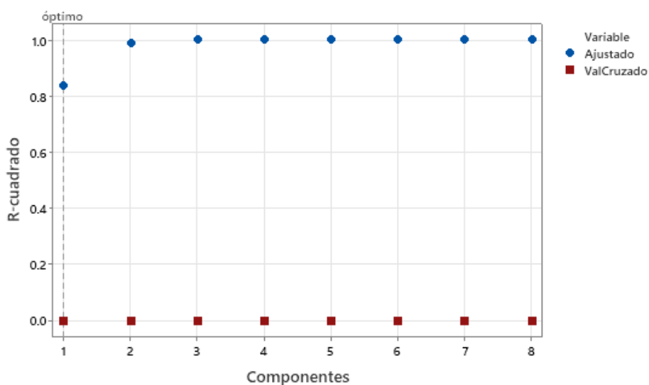
Figura 135. Selección de modelos de PLS para el pH de la variedad Cabernet Sauvignon.
