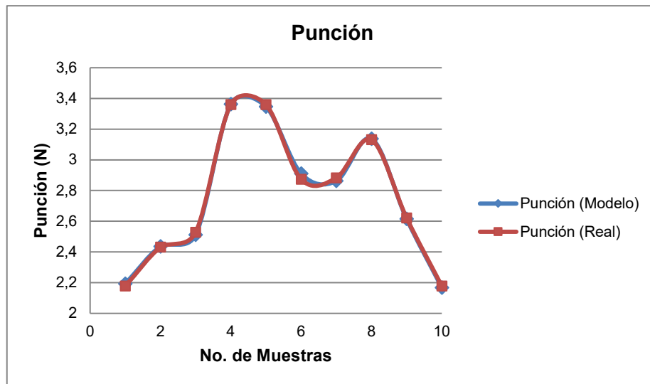
Figura 108. Modelos de predicción vs. valor real para la textura de la variedad de uva Shiraz.
