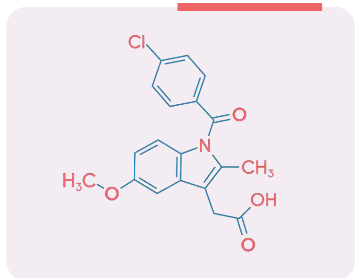
Figura 5 | Fórmula estructural de la Indometacina.
