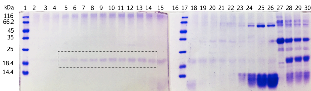
Figura 57. Análisis de fracciones de elución de la separación de SmbP (9.8 kDa) + Brazzein3xNG (19.58 kDa) por IA mediante SDS-PAGE 15%. Carriles 1 y 17: marcador de peso molecular, carriles 2-15: fracciones de elución de Brazzein3xNG, carriles 18-26: fracciones de elución de Brazzein3xNG + SmbP + quimera, carril 27: SmbP_Brazzein3xNG sin digerir, carriles 28, 29 y 30: digestión de SmbP_Brazzein3xNG con enteroquinasa a las 16, 20 y 22 horas de reacción respectivamente.
