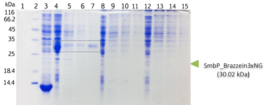
Figura 52. Análisis de expresión de los tándems SmbP_Brazzein3xNG (30.02 kDa), SmbP_Rattusin2xNG (18.05 kDa) y SmbP_Rattusin3xNG (21.86 kDa) en E. coli Origami2(DE3) por SDS-PAGE 15%. Carril 2: marcador de peso molecular, carril 3: control positivo SmbP_STOP (9.8 kDa), carriles 4, 5, 6 y 7: SmbP_Brazzein3xNG, carriles: 8, 9, 10 y 11: SmbP_Rattusin2xNG, carriles 12, 13, 14 y 15: SmbP_Rattusin3xNG.
