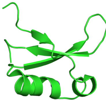
Figura 4. Estructura secundaria de Brazzein. PDBE (2018).
