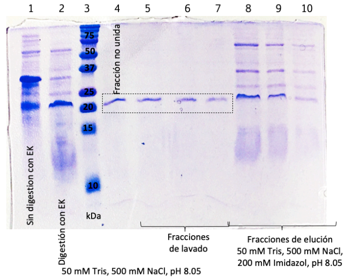
Figura 69. Reacción con enteroquinasa (EK) para la remoción del tag de SmbP_Brazzein FLEX (31.4 kDa). Carril 1: SmbP_Brazzein FLEX (31.4 kDa) sin digerir, carril 2: SmbP (9.8 kDa) + Brazzein FLEX (20.96 kDa) después de la digestión con enteroquinasa, carril 3: marcador de peso molecular, carril 4: percolado/fracción no unida, carriles 5 – 7: fracciones de lavado, carriles 8 – 10: fracciones de elución.
