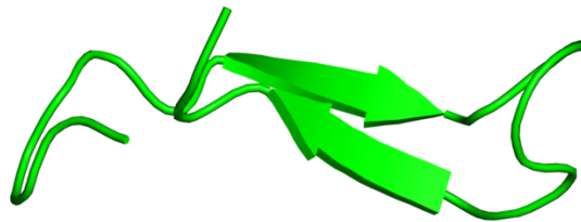
Figura 7. Estructura secundaria de Hepcidin. PDBE (2018)
