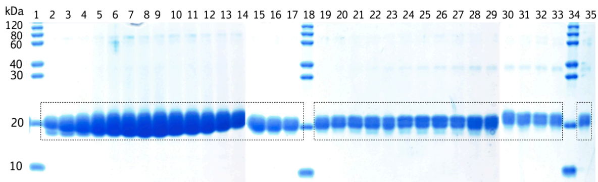
Figura 19. Análisis de fracciones de elución de CusF3H+_Brazzein (17.09 kDa) mediante SDS-PAGE 15%. Carriles 1, 18 y 34: marcador de peso molecular, carriles: 2-17, 19-33 y 35 fracciones de elución.
