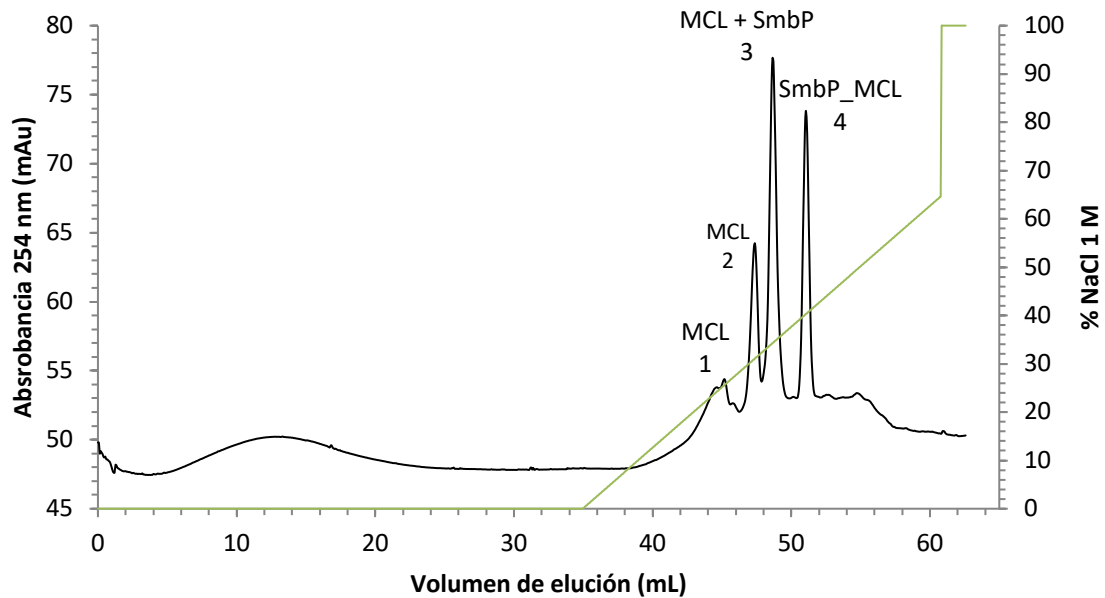
Figura 38. Cromatograma de purificación por intercambio aniónico para SmbP + MCL después de digerir con enteroquinasa. Buffer de equilibrio: 50 mM Tris, pH 8, y buffer de elución: 50 mM Tris, 1M NaCl, pH 8. El pico 1 se obtuvo a los 45.18 mL de elución con una absorbancia de 54.38 mAu y una concentración de 256 mM de NaCl (25.6%). El pico 2 se obtuvo a los 47.38 mL de elución con una absorbancia de 64.22 mAu y una concentración de 311 mM de NaCl (31.1%). El pico 3 se obtuvo a los 48.64 mL de elución con una absorbancia de 77.64 mAu y una concentración de 343 mM de NaCl (34.3%). El pico 4 se obtuvo a los 51.04 mL de elución con una absorbancia de 73.81 mAu y una concentración de 403 mM de NaCl (40.3%).
