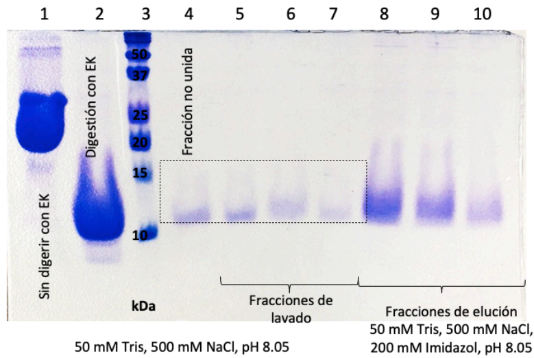
Figura 46. Reacción con enteroquinasa (EK) para la remoción del tag de SmbP_Scygonadin (21.1 kDa). Carril 1: SmbP_Scygonadin (21.1 kDa) sin digerir, carril 2: SmbP (9.8 kDa) + Scygonadin (11.27 kDa) después de la digestión con enteroquinasa, carril 3: marcador de peso molecular, carril 4: percolado/fracción no unida, carriles 5 – 7: fracciones de lavado, carriles 8 – 10: fracciones de elución.
