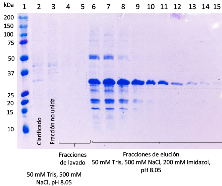
Figura 61. Análisis de fracciones de purificación IMAC de CusF3H+_Brazzein FLEX (31.68 kDa) por SDS-PAGE 12%. Carril 1: marcador de peso molecular, carril 2: lisado/clarificado, carril 3: percolado/fracción no unida, carriles 4 – 5: fracciones de lavado con 50 mM Tris, 500 mM NaCl, pH 8.05, carriles 6 – 15: fracciones de elución de CusF3H+_Brazzein FLEX.
