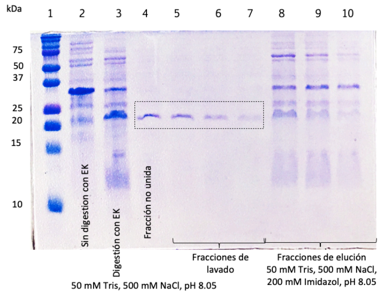
Figura 68. Reacción con enteroquinasa (EK) para la remoción del tag de CusF3H+_Brazzein FLEX (31.68 kDa). Carril 1: marcador de peso molecular, carril 2: CusF3H+_Brazzein FLEX (31.68 kDa) sin digerir, carril 3: CusF3H+ (10.15 kDa) + Brazzein FLEX (20.96 kDa) después de la digestión con enteroquinasa, carril 4: percolado/fracción no unida, carriles 5 – 7: fracciones de lavado, carriles 8 – 10: fracciones de elución.
