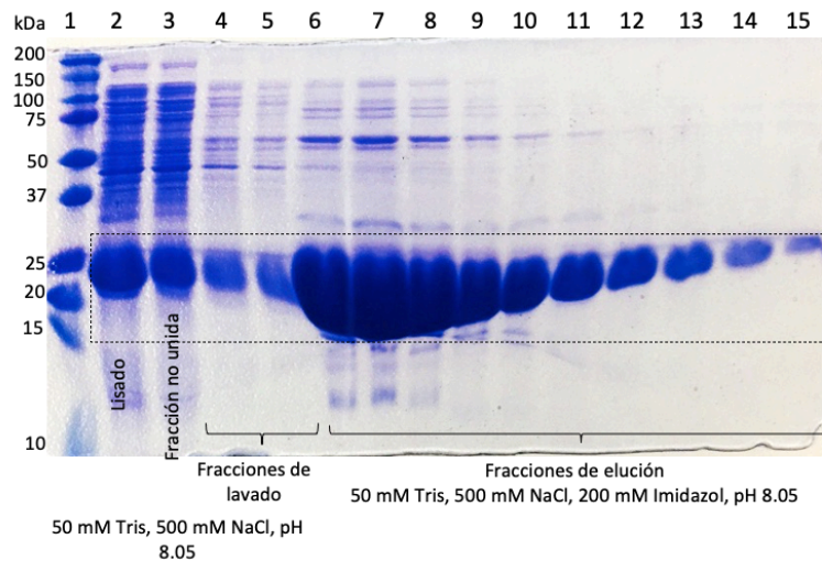
Figura 44. Análisis de fracciones de purificación IMAC de SmbP_Scygonadin (21.1 kDa) por SDS-PAGE 12%. Carril 1: marcador de peso molecular, carril 2: lisado/clarificado, carril 3: percolado/fracción no unida, carriles 4 y 5: fracciones de lavado con 50 mM Tris, 500 mM NaCl, pH 8.05, carriles 6 – 15: fracciones de elución de SmbP_Scygonadin.
