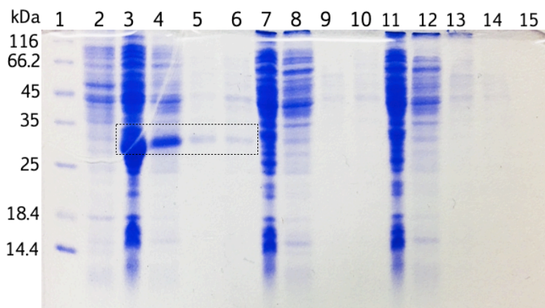
Figura 51. Análisis de expresión de los tándems SmbP_Brazzein3xNG (30.02 kDa), SmbP_Rattusin 2xNG (18.05 kDa) y SmbP_Rattusin3xNG (21.86 kDa) en E. coli SHuffle por SDS-PAGE 15%. Carril 1: marcador de peso molecular, carril 2: control negativo E. coli SHuffle, carriles 3, 4, 5 y 6: SmbP_Brazzein3xNG, carriles: 7, 8 9 y 10: SmbP_Rattusin2xNG, carriles 11, 12, 13 y 14: SmbP_Rattusin3xNG.
