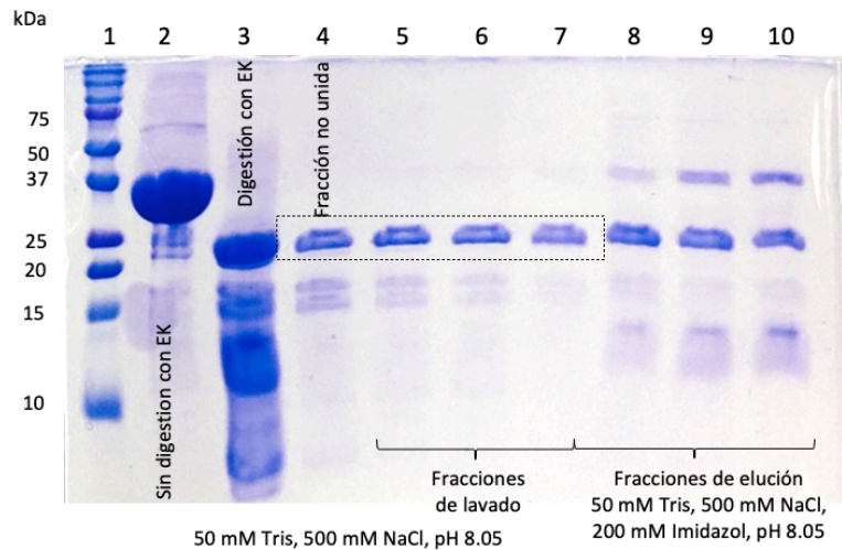
Figura 71. Reacción con enteroquinasa (EK) para la remoción del tag de CusF3H+_Scygonadin FLEX (34.19). Carril 1: marcador de peso molecular, carril 2: CusF3H+_Scygonadin FLEX (34.19 kDa) sin digerir, carril 3: CusF3H+ (10.15 kDa) + Scygonadin FLEX (23.47 kDa) después de la digestión con enteroquinasa, carril 4: percolado/fracción no unida, carriles 5 – 7: fracciones de lavado, carriles 8 – 10: fracciones de elución.
