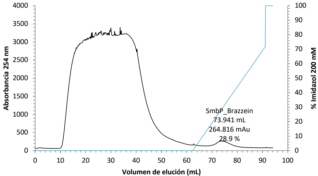
Figura 23. Cromatograma de purificación por afinidad a Ni(II) para SmbP_Brazzein con gradiente de elución. Solución amortiguadora de lisis: 50 mM Tris, 500 mM NaCl, 5 mM imidazol, solución amortiguadora de lavado: 50mM Tris, 500mM NaCl, 10mM imidazol y solución amortiguadora de elución: 50 mM Tris, 500 mM NaCl, 200 mM imidazol pH 8. El pico de elución más alto se obtuvo a los 73.9 mL de elución con una absorbancia de 264.81.621 mAu
