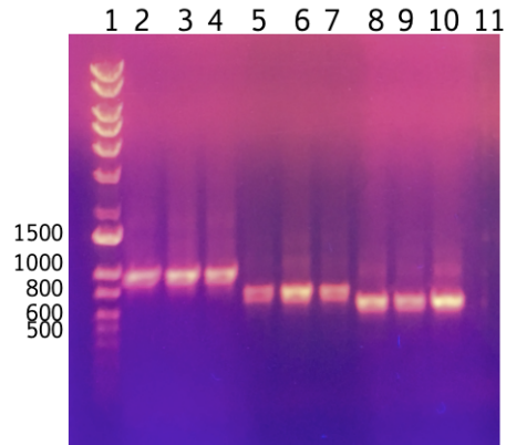
Figura 49. Productos de PCR para la confirmación de las construcciones en tándem con SmbP en gel de agarosa al 0.7%. Carril 1: marcador de peso molecular, carriles 2, 3 y 4: SmbP_Brazzein3xNG (989 pb), carriles 5, 6 y 7: SmbP_Rattusin3xNG (791 pb), carriles 8,9 y 10: SmbP_Rattusin2xNG (692 pb).
