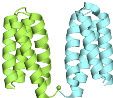
Figura 3. Estructura secundaria de SmbP. PDBE (2020)
