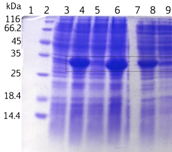
Figura 35. Análisis de microexpresión de SmbP_MCL(31.72 kDa) y CusF3H+_MCL (32.07 kDa) en medio Native Folder mediante SDS-PAGE 15%. Carril 2: marcador de peso molecular, carril 3: SmbP_MCL antes de la inducción con calentamiento a 95°C, carril 4: SmbP_MCL después de la inducción con calentamiento a 95°C, carril 5: CusF3H+_MCL antes de la inducción con calentamiento a 95°C, carril 6: CusF3H+_MCL después de la inducción con calentamiento a 95°C, carril 8: SmbP_MCL después de la inducción por lisis con perlas de vidrio, carril 9: CusF3H+_MCL después de la inducción por lisis con perlas de vidrio.
