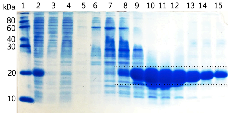
Figura 15. Análisis de fracciones de elución de CusF3H+_Brazzein (17.09 kDa) mediante SDS-PAGE 15%. Carril 1: marcador de peso molecular, carril 2: lisado, carril 3: percolado, carril 4: lavado, carriles 5-15: fracciones de elución.
