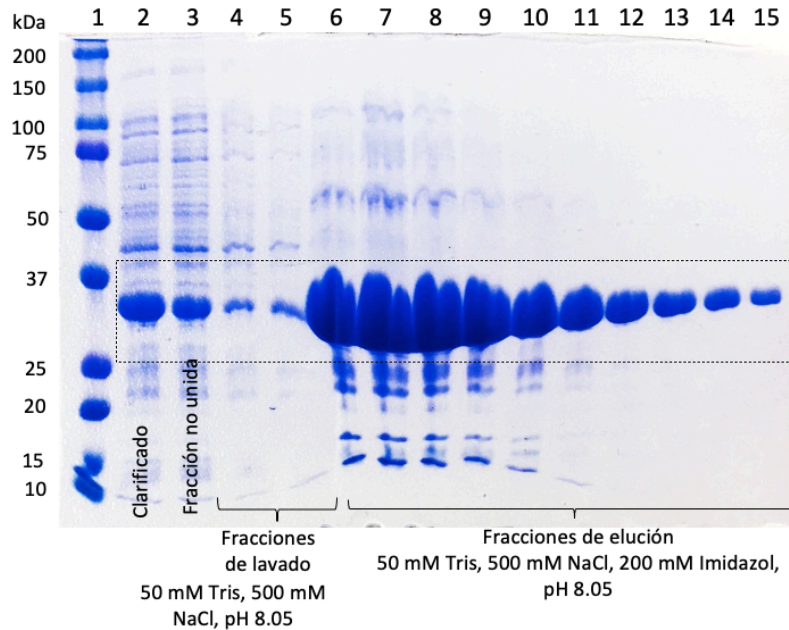
Figura 65. Análisis de fracciones de purificación IMAC de CusF3H+_Scygonadin FLEX (34.19 kDa) por SDS-PAGE 12%. Carril 1: marcador de peso molecular, carril 2: lisado/clarificado, carril 3: percolado/fracción no unida, carriles 4–7: fracciones de lavado con 50 mM Tris, 500 mM NaCl, pH 8.05, carriles 8–15: fracciones de elución de CusF3H+_Scygonadin FLEX.
