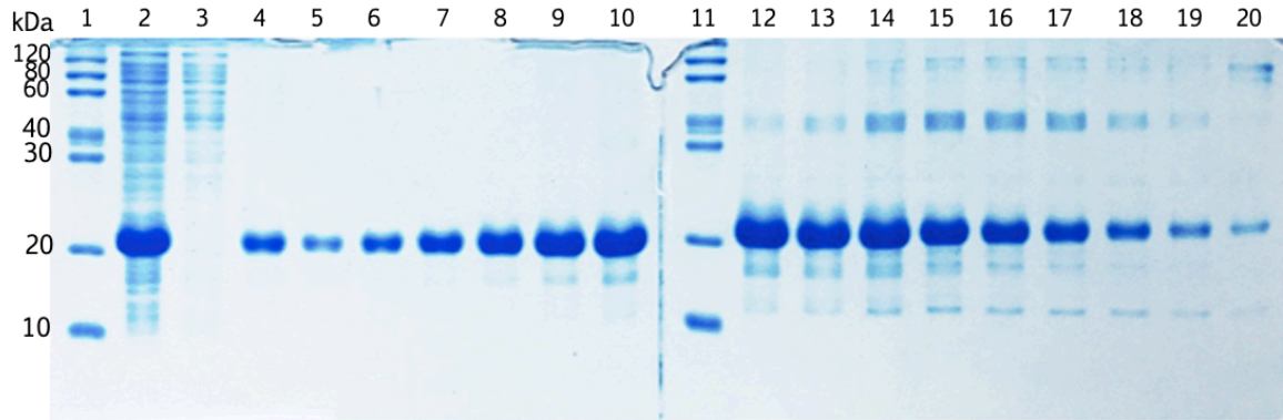
Figura 24. Análisis de fracciones de elución de SmbP_Brazzein (16.8 kDa) mediante SDS-PAGE 15%. Carriles 1 y 11: marcador de peso molecular, carril 2: lisado, carril 3: percolado, carriles 4: lavado 5-10 y 12-20: fracciones de elución
