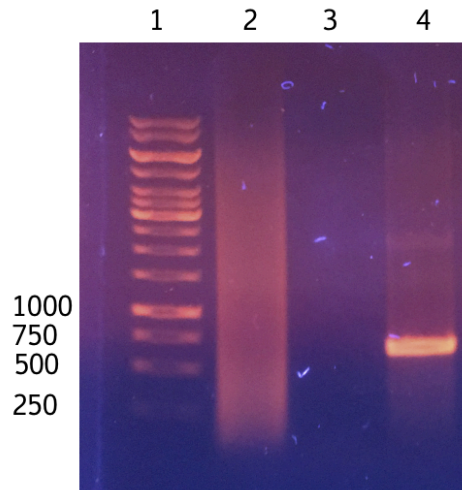
Figura 10. Amplificación de miraculin en gel de agarosa al 0.7%. El carril 1 muestra el marcador de peso molecular, en el carril 2 se muestra un control negativo con enzima sin ADN molde, en el carril 3 el control negativo sin enzima con ADN molde y en el carril 4 se encuentra la amplificación de Miraculin (573 pb).
