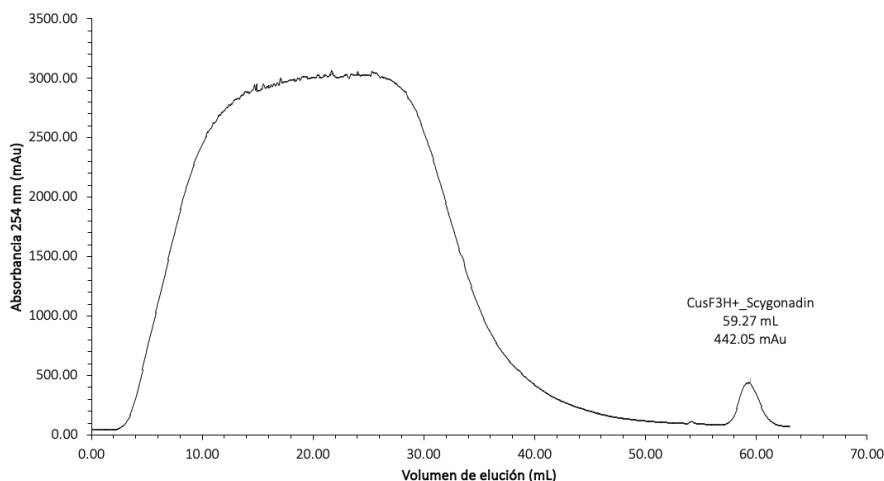
Figura 41. Cromatograma de purificación por afinidad a Ni(II) para CusF3H+_Scygonadin. Solución amortiguadora de lisis y lavado: 50 mM Tris, 500 mM NaCl, 5 mM imidazol, pH 8 y solución amortiguadora de elución: 50 mM Tris, 500 mM NaCl, 200 mM imidazol, pH 8.
