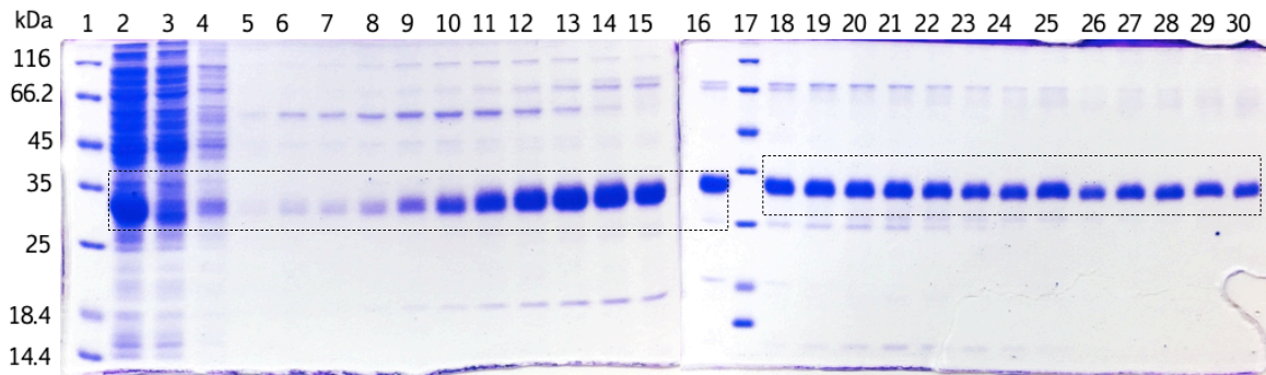
Figura 54. Análisis de fracciones de elución de SmbP_Brazzein3xNG (30.02 kDa) mediante SDS-PAGE 15%. Carriles 1 y 17: marcador de peso molecular, carril 2: clarificado, carril 3: percolado, carril 4: lavado, carriles 5-16 y 18-30: fracciones de elución.
