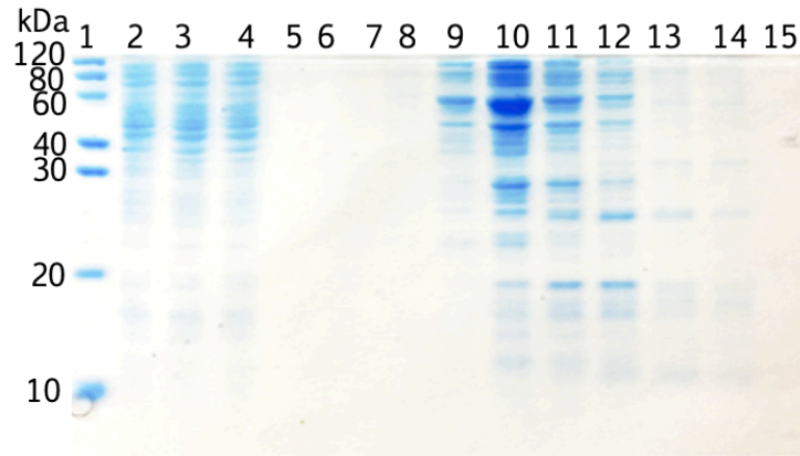
Figura 30. Análisis de fracciones de elución de CusF3H+_MCL (32.07 kDa) mediante SDS-PAGE 15%. Carril 1: marcador de peso molecular, carril 2: lisado, carril 3: percolado, carril 4: lavado, carriles 5-15: fracciones de elución.
