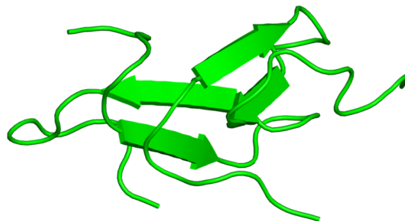
Figura 6. Estructura secundaria de Rattusin. PDBE (2018)
