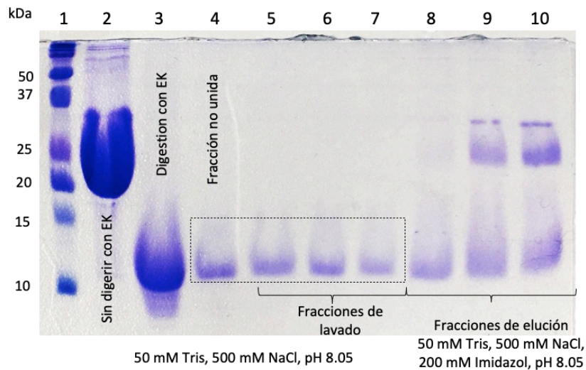
Figura 45. Reacción con enteroquinasa (EK) para la remoción del tag de CusF3H+_Scygonadin (21.4). Carril 1: marcador de peso molecular, carril 2: CusF3H+_Scygonadin (21.4 kDa) sin digerir, carril 3: CusF3H+ (10.15 kDa) + Scygonadin (11.27 kDa) después de la digestión con enteroquinasa, carril 4: percolado/fracción no unida, carriles 5 – 7: fracciones de lavado, carriles 8 – 10: fracciones de elución.
