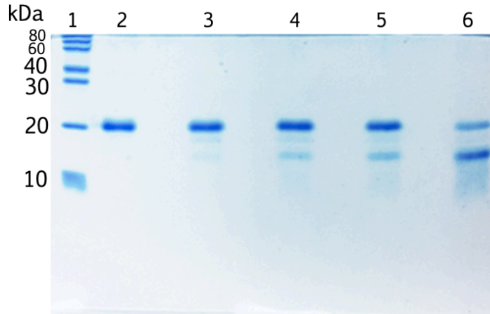
Figura 21. Análisis de digestión a 25°C con la enzima enteroquinasa para CusF3H+_Brazzein mediante SDS-PAGE 18%. Carril 1: marcador de peso molecular, carril 2: CusF3H+_Brazzein sin digerir, carril 3: 2 horas de digestión, carril 4: 4 horas de digestión, carril 5: 6 horas de digestión y carril 6: 24 horas de digestión.
