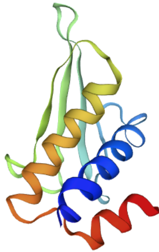
Figura 8. Estructura secundaria de Scygonadin. Biozentrum (2020)
