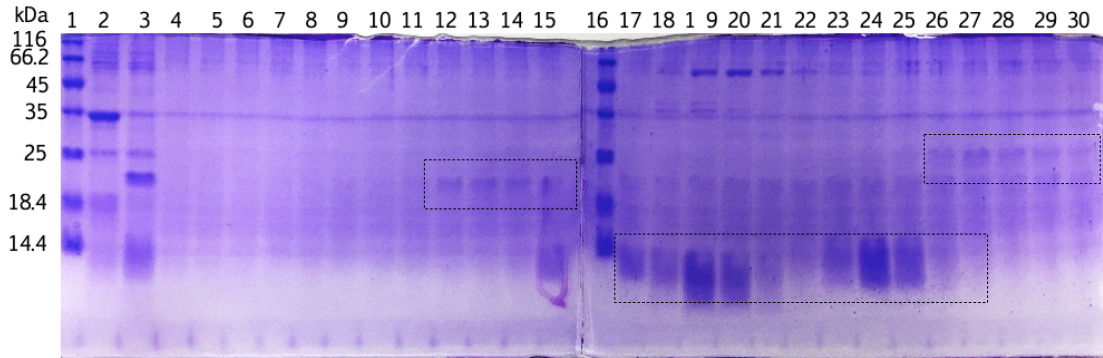
Figura 39. Análisis de fracciones de elución de la separación de SmbP (9.8 kDa) + MCL (21.35 kDa) por IA mediante SDS-PAGE 15%. Carriles 1 y 16: marcador de peso molecular, carril 2: SmbP_MCL sin digerir, carril 3: Digestión de SmbP_MCL con enteroquinasa, carriles 12-15: fracciones de elución de MCL, carriles 17-25: fracciones de elución de MCL + SmbP y carriles 26-30: fracciones de elución de SmbP_MCL.
