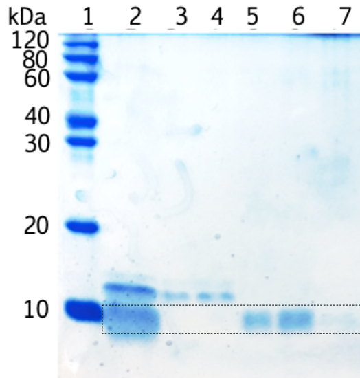
Figura 26. Análisis de fracciones de elución por exclusión por tamaño de SmbP (9.8 kDa) y Brazzein (6.37 kDa) mediante SDS-PAGE 16%. Carril 1: marcador de peso molecular, carril 2: SmbP_Brazzein después de digestión con enteroquinasa, carriles 3 y 4: fracciones de elución de SmbP y carriles 5-7: fracciones de elución de Brazzein.
