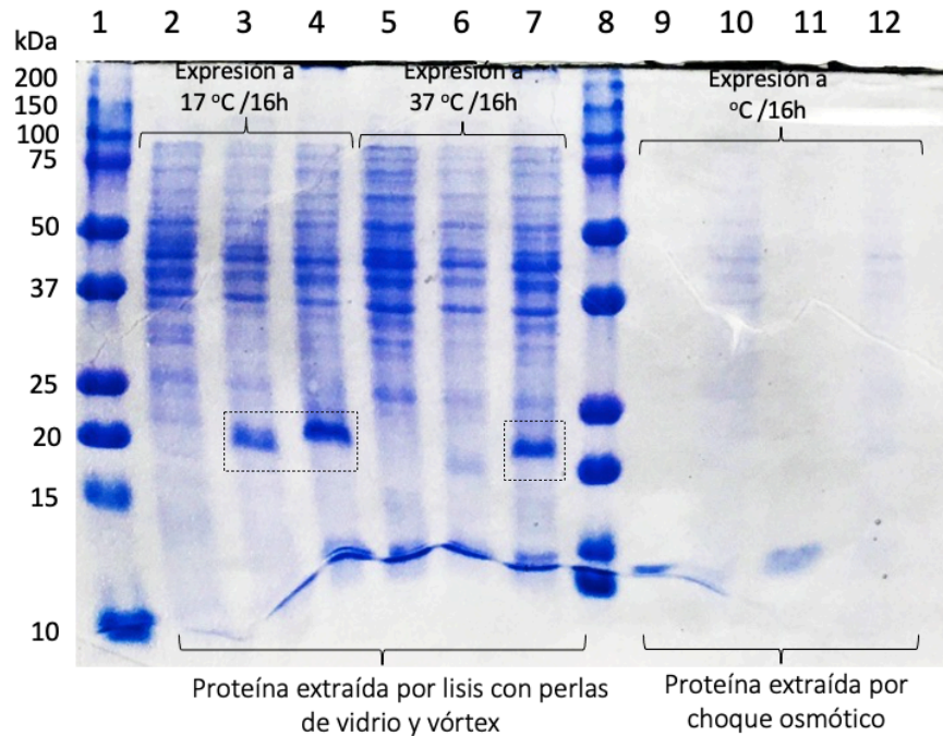
Figura 60. Microexpresión a diferentes condiciones de PelB_SmbP_Hepcidin FLEX (20.68 kDa), CusF3H+_Hepcidin FLEX (20.97 kDa) y SmbP_Hepcidin FLEX (20.68 kDa). Carril 1: marcador de peso molecular, carril 2: control negativo E. coli SHuffle a 17 °C /16 horas/0.1 mM IPTG, carril 3: CusF3H+_Hepcidin FLEX, carril 4: SmbP_Hepcidin FLEX, carril 5: control negativo E. coli SHuffle a 37 °C /16 horas/0.1 mM IPTG, carril 6: CusF3H+_Hepcidin FLEX, carril 7: SmbP_Hepcidin FLEX, carril 8: marcador de peso molecular, carril 9: F. Hiper. E. coli BL21(DE3), carril 10: F. Hipo E. coli BL21(DE3), carril 11: F. Hiper PelB_SmbP_Hepcidin FLEX, carril 12: F. Hipo PelB_SmbP_Hepcidin FLEX.
