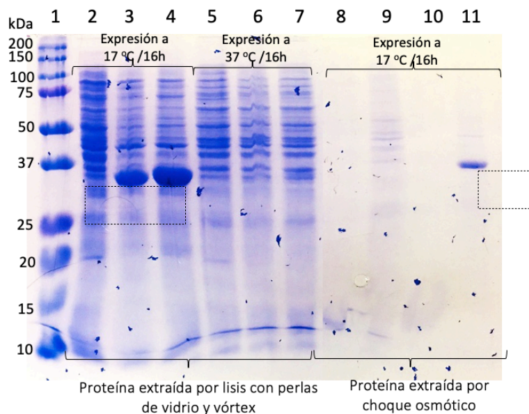
Figura 59. Microexpresión a diferentes condiciones de PelB_SmbP_Scygonadin FLEX (33.9 kDa), CusF3H+_Scygonadin FLEX (34.19 kDa) y SmbP_Scygonadin FLEX (33.9 kDa). Carril 1: marcador de peso molecular, carril 2: control negativo E. coli SHuffle a 17 °C /16 horas/0.1 mM IPTG, carril 3: CusF3H+_Scygonadin FLEX, carril 4: SmbP_Scygonadin FLEX, carril 5: control negativo E. coli SHuffle a 37 °C /16 horas/0.1 mM IPTG, carril 6: CusF3H+_Scygonadin FLEX, carril 7: SmbP_Scygonadin FLEX, carril 8: F. Hiper. E. coli BL21(DE3), carril 9: F. Hipo E. coli BL21(DE3), carril 10: F. Hiper PelB_SmbP_Scygonadin FLEX, carril 11: F. Hipo PelB_SmbP_Scygonadin FLEX.
