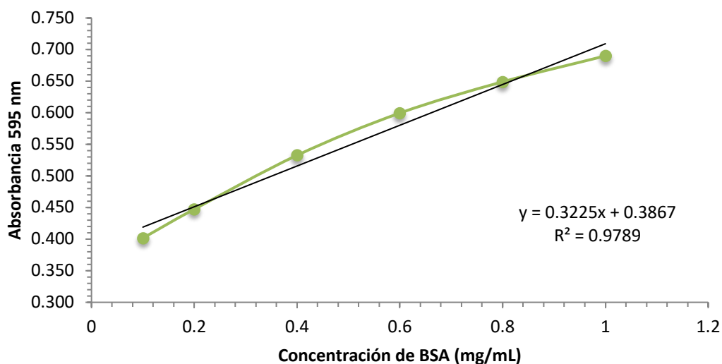
Figura 20. Curva de calibración de BSA para la cuantificación de CusF3H+_Brazzein
