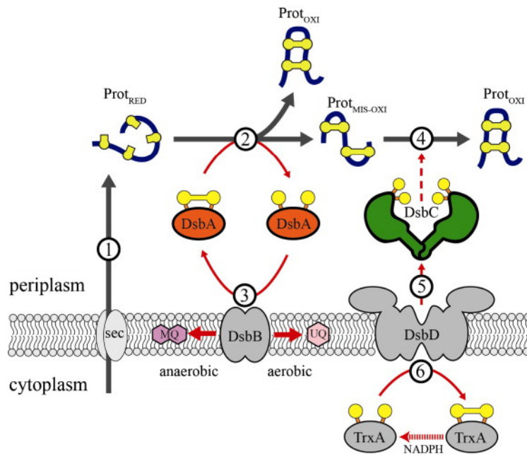
Figura 1. Formación de enlaces disulfuro en el periplasma de Escherichia coli . Berkmen (2012)
