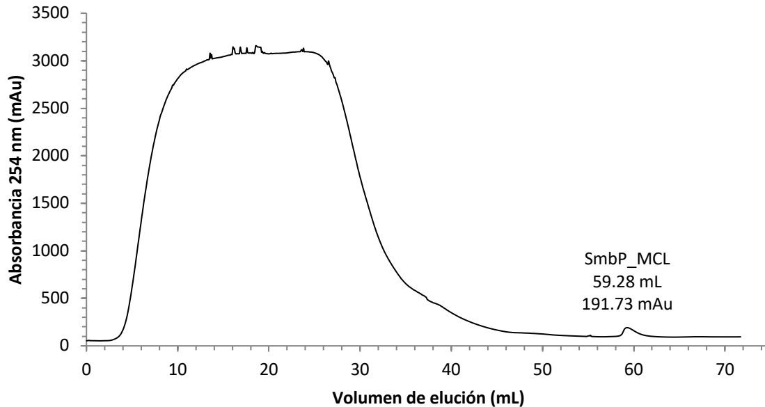
Figura 36. Cromatograma de purificación por afinidad a Ni(II) para SmbP_MCL expresada en Native Folder. Solución amortiguadora de lisis y lavado: 50 mM Tris, 500 mM NaCl, 5 mM imidazol, pH 8 y solución amortiguadora de elución: 50 mM Tris, 500 mM NaCl, 200 mM imidazol, pH 8. El pico de elución se obtuvo a los 59.28 mL de elución con una absorbancia de 191.73 mAu.
