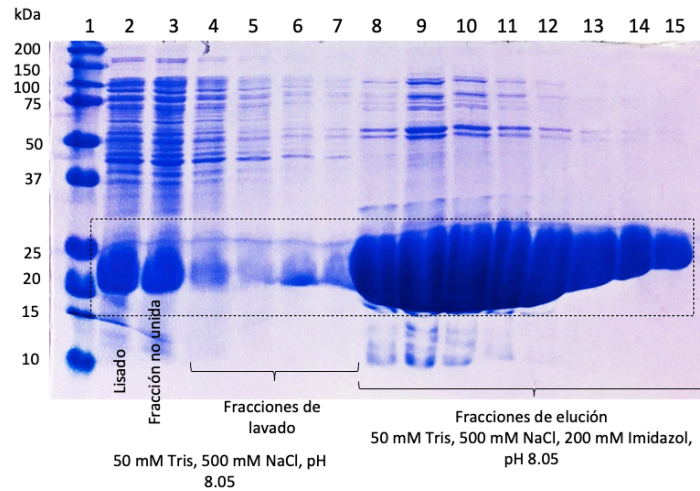
Figura 42. Análisis de fracciones de purificación IMAC de CusF3H+_Scygonadin (21.4 kDa) por SDS-PAGE 12%. Carril 1: marcador de peso molecular, carril 2: lisado/clarificado, carril 3: percolado/fracción no unida, carriles 4 – 7: fracciones de lavado con 50 mM Tris, 500 mM NaCl, pH 8.05, carriles 8 – 15: fracciones de elución de CusF3H+_Scygonadin.
