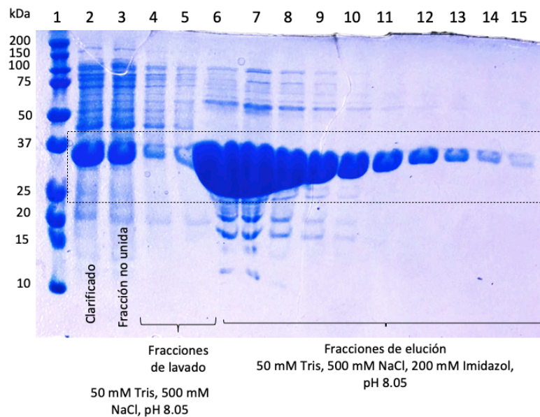
Figura 67. Análisis de fracciones de purificación IMAC de SmbP_Scygonadin FLEX (33.9 kDa) por SDS-PAGE 12%. Carril 1: marcador de peso molecular, carril 2: lisado/clarificado, carril 3: percolado/fracción no unida, carriles 4 y 5: fracciones de lavado con 50 mM Tris, 500 mM NaCl, pH 8.05, carriles 6 – 15: fracciones de elución de SmbP_Scygnadin FLEX
