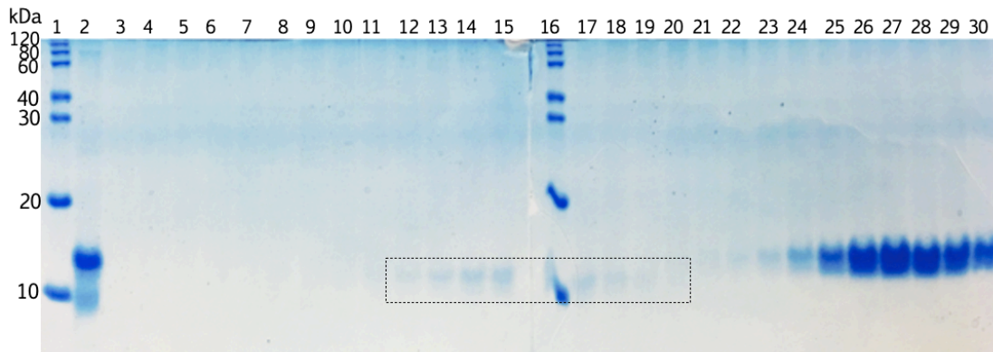
Figura 28. Análisis de fracciones de elución de la separación de SmbP (9.8 kDa) + Brazzein (6.37 kDa) por IA mediante SDS-PAGE 15%. Carriles 1 y 16: marcador de peso molecular, carril 2: Digestión de SmbP_Brazzein con enteroquinasa, carriles 12-20: fracciones de elución de Brazzein, carriles 23-30: fracciones de elución de SmbP.
