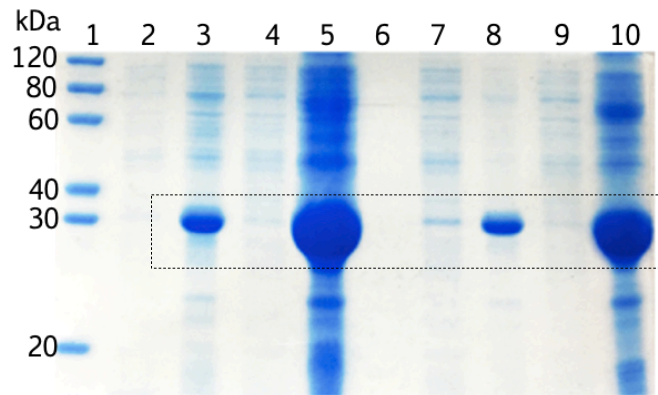
Figura 31. Análisis de fracciones del tratamiento con lisozima, lisozima/triton y lisis celular para CusF3H+_MCL (32.07 kDa) por SDS-PAGE 15%. Carril 1: marcador de peso molecular, carril 2: clarificado del tratamiento con lisozima, carril 3: residuo celular del tratamiento con lisozima, carril 4: clarificado del tratamiento con lisozima después de la lisis celular, carril 5: residuo celular del tratamiento con lisozima después de la lisis celular, carril 7: clarificado del tratamiento con lisozima y triton, carril 8: residuo celular del tratamiento con lisozima y triton, carril 9: clarificado del tratamiento con lisozima, lisis celular y triton, carril 10: residuo celular del tratamiento con lisozima, lisis celular y triton.
