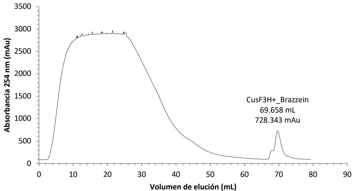
Figura 14. Cromatograma de purificación por afinidad a Ni(II) para CusF3H+_Brazzein. Solución amortiguadora de lisis y lavado: 50 mM Tris, 500 mM NaCl, solución amortiguadora de elución: 50 mM Tris, 500 mM NaCl, 200 mM imidazol pH 8. El pico de elución se obtuvo a los 69.658 mL de elución con una absorbancia de 728.343 mAu.
