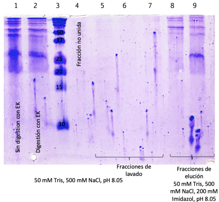
Figura 70. Reacción con enteroquinasa (EK) para la remoción del tag de SmbP_Hepcidin FLEX (20.68 kDa). Carril 1: SmbP_Hepcidin FLEX (20.68 kDa) sin digerir, carril 2: SmbP (9.8 kDa) + Hepcidin FLEX (10.24 kDa) después de la digestión con enteroquinasa, carril 3: marcador de peso molecular, carril 4: percolado/fracción no unida, carriles 5 – 7: fracciones de lavado, carriles 8 – 10: fracciones de elución.
