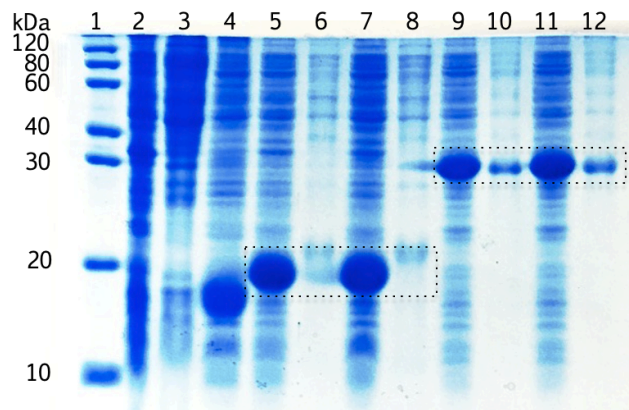
Figura 13. Expresiones en pequeña escala para CusF3H+_Brazzein (17.09 kDa) y CusF3H+_MCL (32.07 kDa) mediante SDS-PAGE al 15%. Carril 1: marcador de peso molecular, carril 2: fracción soluble E. coli SHuffle T7 express, carril 3: fracción insoluble E. coli SHuffle T7 express, carril 4: fracción soluble CusF3H+, carril 5 y 7: fracción soluble de CusF3H+_Brazzein, carril 6 y 8: fracción insoluble de CusF3H+_Brazzein, carril 9 y 11: fracción soluble CusF3H+_Miraculin y carril 10 y 12: fracción insoluble de CusF3H+_Miraculin.
