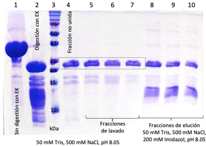
Figura 72. Reacción con enteroquinasa (EK) para la remoción del tag de SmbP_Scygonadin FLEX (33.9 kDa). Carril 1: SmbP_Scygonadin (33.9 kDa) sin digerir, carril 2: SmbP (9.8 kDa) + Scygonadin (23.47 kDa) después de la digestión con enteroquinasa, carril 3: marcador de peso molecular, carril 4: percolado/fracción no unida, carriles 5 – 7: fracciones de lavado, carriles 8 – 10: fracciones de elución.
