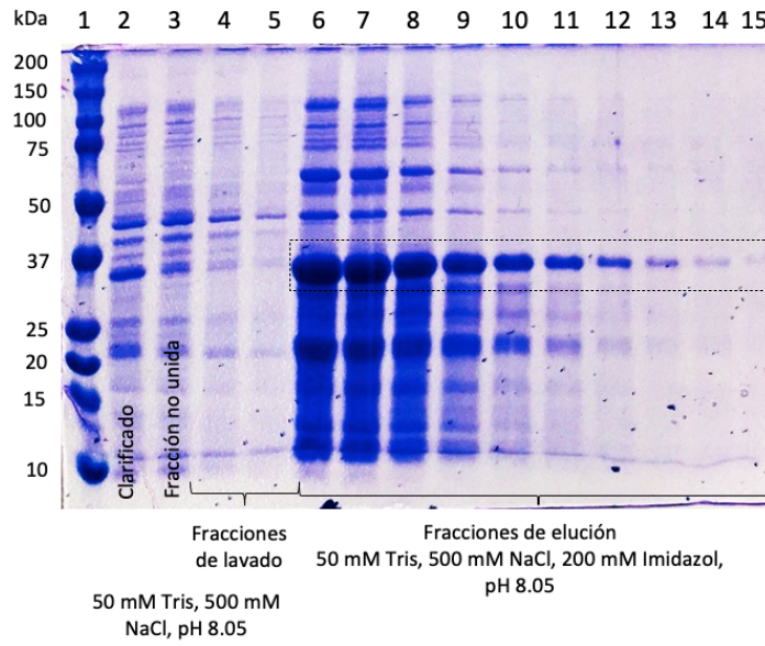
Figura 62. Análisis de fracciones de purificación IMAC de SmbP_Brazzein FLEX (31.4 kDa) por SDS-PAGE 12%. Carril 1: marcador de peso molecular, carril 2: lisado/clarificado, carril 3: percolado/fracción no unida, carriles 4 y 5: fracciones de lavado con 50 mM Tris, 500 mM NaCl, pH 8.05, carriles 6 – 15: fracciones de elución de SmbP_Brazzein FLEX
