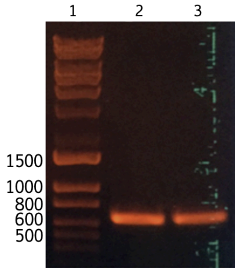
Figura 12. Productos de la PCR para la confirmación de la construcción SmbP_Brazzein (653 pb) en gel de agarosa al 0.7%. Carril 1: marcador de peso molecular, carriles 2 y 3: ADNs plasmídicos analizados.
