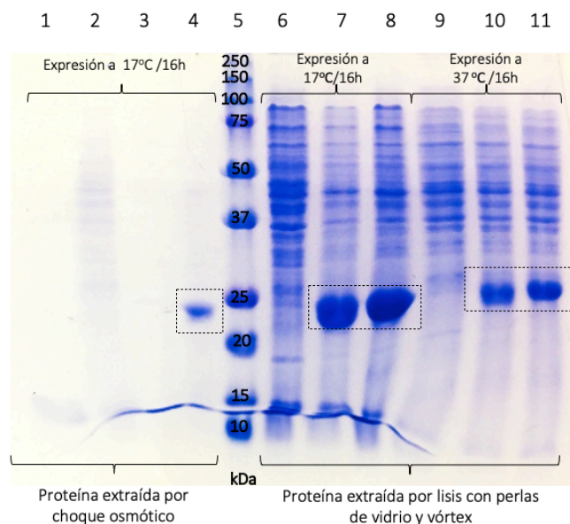
Figura 40. Microexpresión a diferentes condiciones de PelB_SmbP_Scygonadin (21.1 kDa), CusF3H+_Scygonadin (21.4 kDa) y SmbP_Scygonadin (21.1 kDa). Carril 1: F- Hiper. E. coli BL21(DE3), carril 2: F. hipo E. coli BL21(DE3), carril 3: F. Hiper PelB_SmbP_Scygonadin, carril 4: F. Hipo. PelB_SmbP_Scygonadin, carril 5: marcador de peso molecular, carril 6: control negativo E. coli Shuffle T7 express a 17 °C /16 horas/0.1 mM IPTG, carril 7: CusF3H+_Scygonadin, carril 8: SmbP_Scygonadin, carril 9: control negativo E. coli Shuffle T7 express a 37 °C /16 horas/0.1 mM IPTG, carril 10: CusF3H+_Scygonadin y carril 11: SmbP_Scygonadin.
