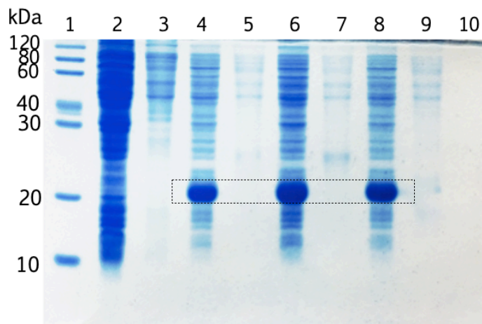
Figura 22. Expresiones en pequeña escala para SmbP_Brazzein (16.8 kDa) mediante SDS-PAGE al 15%. Carril 1: marcador de peso molecular, carril 2: fracción soluble E. coli SHuffle T7 express, carril 3: fracción insoluble E. coli SHuffle T7 express, carriles 4, 6 y 8: fracción soluble SmbP_Brazzein, carril 5, 7 y 9: fracción insoluble de SmbP_Brazzein.
