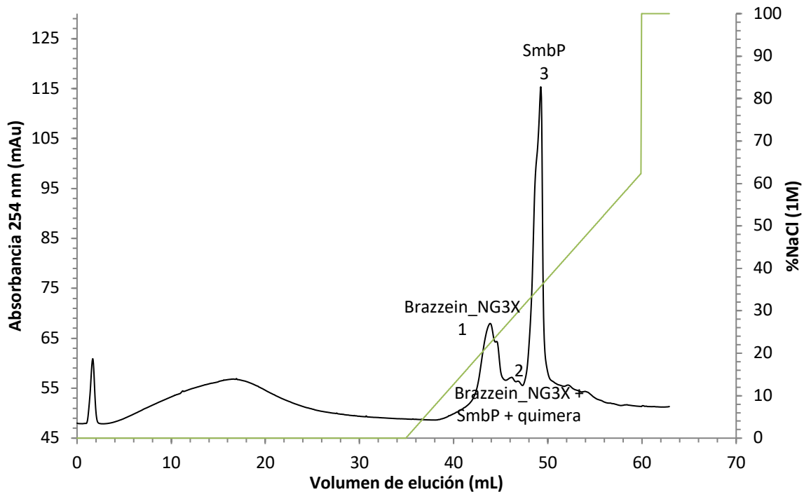
Figura 56. Cromatograma de purificación por intercambio aniónico para SmbP + Brazzein3xNG después de digerir con enteroquinasa. Buffer de equilibrio: 50 mM Tris, pH 8, y buffer de elución: 50 mM Tris, 1M NaCl, pH 8. El pico 1 se obtuvo a los 43.89 mL de elución con una absorbancia de 67.94 mAu y una concentración de 224 mM de NaCl (22.4%). El pico 2 se obtuvo a los 45.23 mL de elución con una absorbancia de 56.97 mAu y una concentración de 258 mM de NaCl (25.8%). El pico 3 se obtuvo a los 49.24 mL de elución con una absorbancia de 115.34 mAu y una concentración de 358 mM de NaCl (35.8%).
