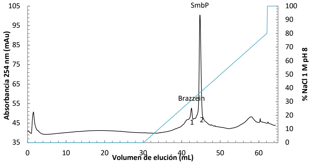
Figura 27. Cromatograma de purificación por intercambio aniónico para SmbP + Brazzein después de digerir con enteroquinasa. Buffer de equilibrio: 50 mM Tris, pH 8, y buffer de elución: 50 mM Tris, 1 M NaCl, pH 8. El pico de elución de Brazzein se obtuvo a los 42.54 mL de elución con una absorbancia de 52.67 mAu y una concentración de 312 mM de NaCl (31.2%).
