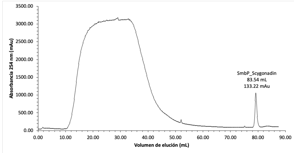
Figura 43. Cromatograma de purificación por afinidad a Ni(II) para SmbP_Scygonadin. Solución amortiguadora de lisis y lavado: 50 mM Tris, 500 mM NaCl, 5 mM imidazol, pH 8 y solución amortiguadora de elución: 50 mM Tris, 500 mM NaCl, 200 mM imidazol, pH 8.
