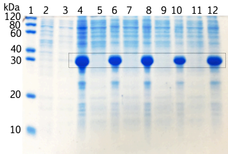
Figura 32. Análisis de fracciones del tratamiento con NaCl/Triton X-100 para CusF3H+_MCL (32.07 kDa) por SDS-PAGE 15%. Carril 1: marcador de peso molecular, carril 2: clarificado después de la lisis celular, carril 3: clarificado del tratamiento con 50 mM Tris, 1M NaCl, carril 4: residuo celular del tratamiento con 50 mM Tris, 1M NaCl, carril 5: clarificado del tratamiento con 50 mM Tris, 1M NaCl, 1% triton X-100, carril 6: residuo celular del tratamiento con 50 mM Tris, 1M NaCl, 1% triton X-100, carril 7: clarificado del tratamiento con 50 mM Tris, 1M NaCl, 1.8% triton X-100, carril 8: residuo celular del tratamiento con 50 mM Tris, 1M NaCl, 1.8% triton X-100, carril 9: clarificado del tratamiento con 50 mM Tris, 1M NaCl, 2.1% triton X-100, carril 10: residuo celular del tratamiento con 50 mM Tris, 1M NaCl, 2.1% triton X-100, carril 11: clarificado del tratamiento con 50 mM Tris, 1M NaCl, 2.1% triton X-100 por toda la noche, carril 12: residuo celular del tratamiento con 50 mM Tris, 1M NaCl, 2.1% triton X-100 por toda la noche.
