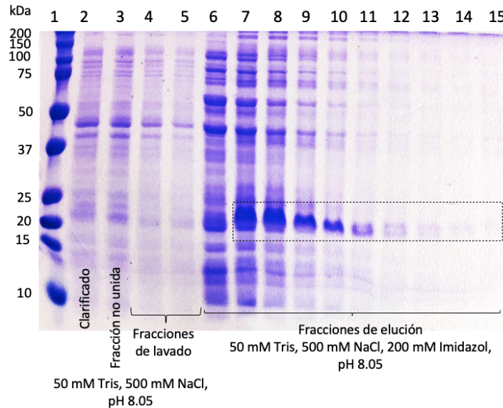
Figura 64. Análisis de fracciones de purificación IMAC de SmbP_Hepcidin FLEX (20.68 kDa) por SDS-PAGE 12%. Carril 1: marcador de peso molecular, carril 2: lisado/clarificado, carril 3: percolado/fracción no unida, carriles 4 y 5: fracciones de lavado con 50 mM Tris, 500 mM NaCl, pH 8.05, carriles 6 – 15: fracciones de elución de SmbP_Hepcidin FLEX.
