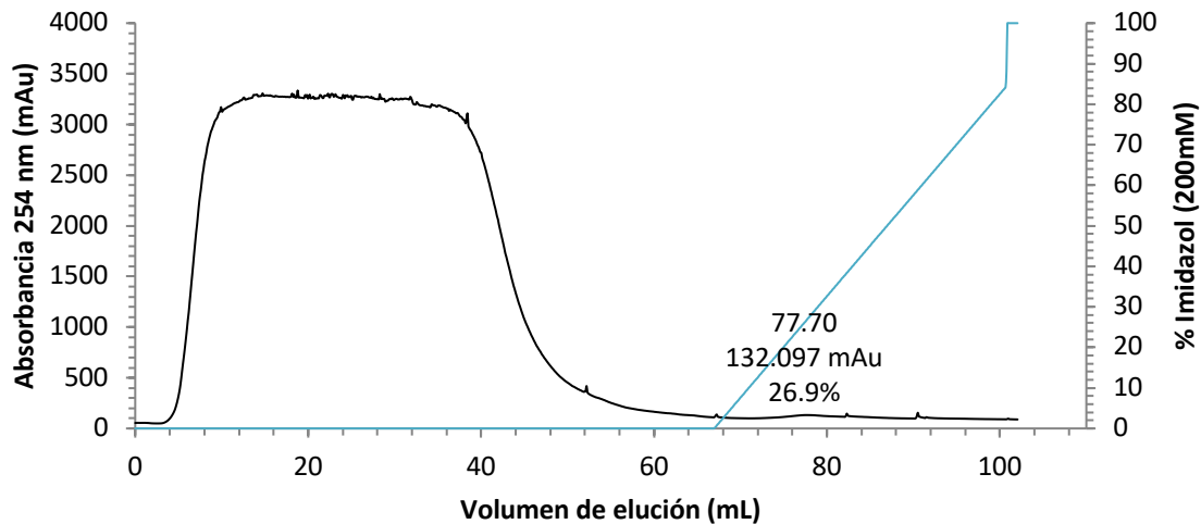
Figura 53. Cromatograma de purificación por afinidad a Ni(II) para SmbP_Brazzein_NG3X con gradiente de elución. Solución amortiguadora de lisis: 50 mM Tris, 500 mM NaCl, 5 mM imidazol, solución amortiguadora de lavado: 50 mM Tris, 500 mM NaCl, 10 mM imidazol y solución amortiguadora de elución: 50 mM Tris, 500 mM NaCl, 200 mM imidazol pH 8. El pico de elución más alto se obtuvo a los 77.7 mL de elución con una absorbancia de 132.09 mAu.
