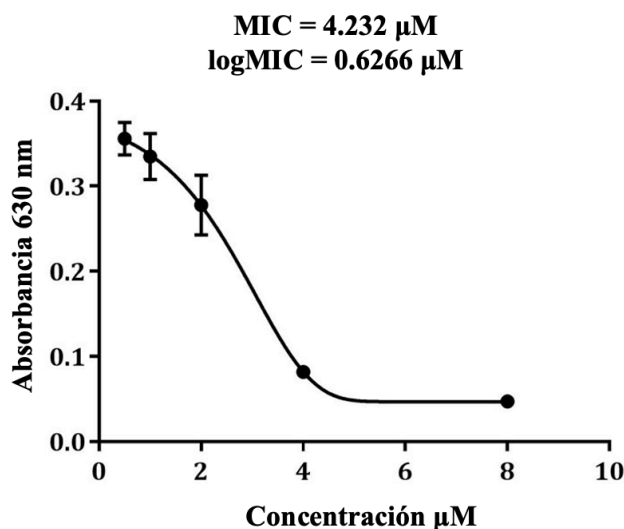
Figura 47. Actividad antimicrobiana de Scygonadin contra 1 \times 10^5 UFC/mL de Staphylococcus aureus . Los puntos en la gráfica representan cada concentración de Scygonadin evaluada a las 24 h de incubación. Las barras de error representan la desviación estándar entre las tres replicas. El resultado de la prueba T de Student reveló diferencias significativas contra el control negativo ( p < 0.05 ).
