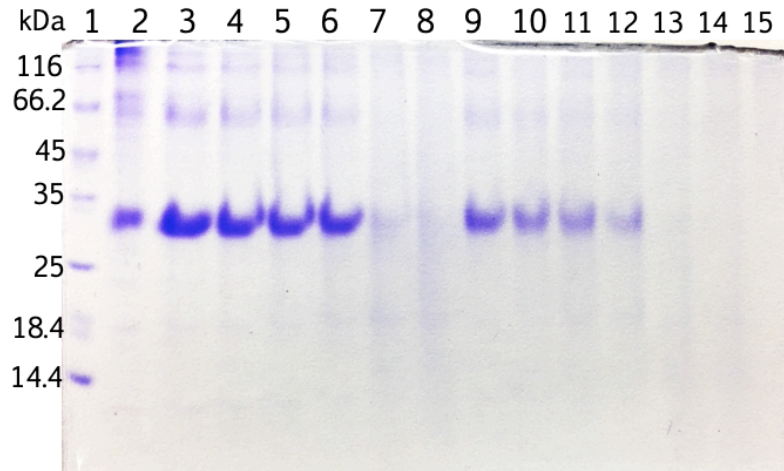
Figura 55. Análisis de digestión con hidroxilamina a 1M y 2M para SmbP_Brazzein3xNG (30.02 kDa) mediante Tricina-SDS-PAGE 15%. Carril 1: marcador de peso molecular, carril 2: SmbP_Brazzein3xNG sin digerir, carriles 3-8: digestión con 1 M \text{NH}_2\text{OH} a 1, 2, 3, 4, 17 y 20 horas de reacción, carriles 9-14: digestión con 2 M \text{NH}_2\text{OH} a 1, 2, 3, 4, 17 y 20 horas de reacción.
