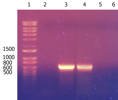
Figura 11. Productos de la PCR para la confirmación de la construcción CusF3H+_Miraculin en gel de agarosa al 0.7%. Carril 1: marcador de peso molecular, Carriles 2-4: ADNs plasmídicos analizados, carril 5: control negativo con enzima sin ADN molde y carril 6: control negativo sin enzima con ADN molde.
