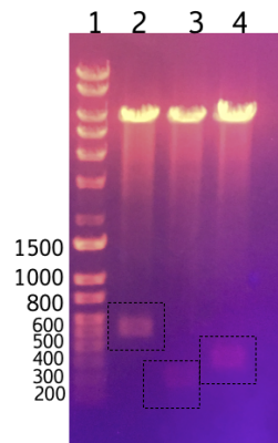
Figura 48. Análisis de restricción con NcoI y XhoI para la confirmación de las construcciones en tándem con CusF3H+ en gel de agarosa al 0.7%. Carril 1: marcador de peso molecular, carril 2: CusF3H+_Brazzein3xNG (495 pb), carril 3: CusF3H+_Rattusin2xNG (198 pb) y carril 4: CusF3H+_Rattusin3xNG (297 pb).
