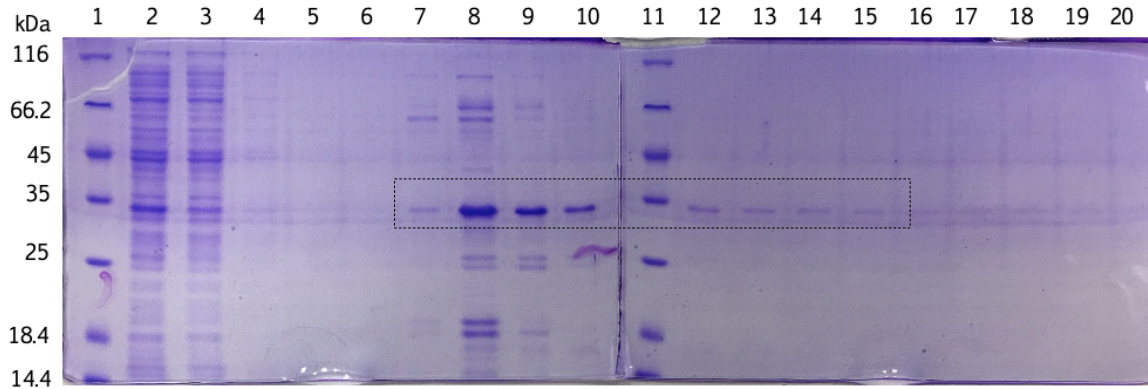
Figura 37. Análisis de fracciones de elución de SmbP_MCL (31.72 kDa) expresada en Native Folder mediante SDS-PAGE 15%. Carriles 1 y 11: marcador de peso molecular, carril 2: lisado, carril 3: percolado, carril 4: lavado, carriles 5-10 y 12-20: fracciones de elución.
