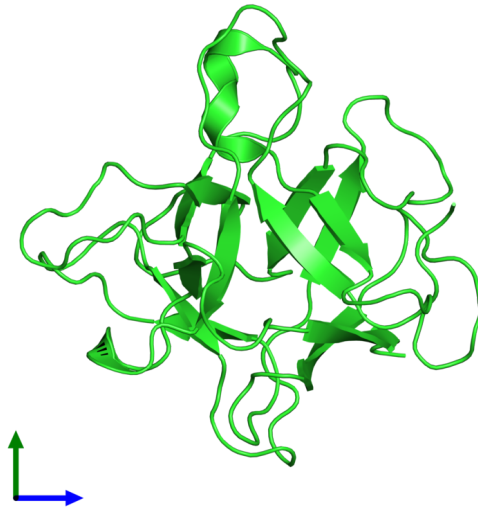
Figura 5. Estructura secundaria de Miraculin. PDBE (2018)
