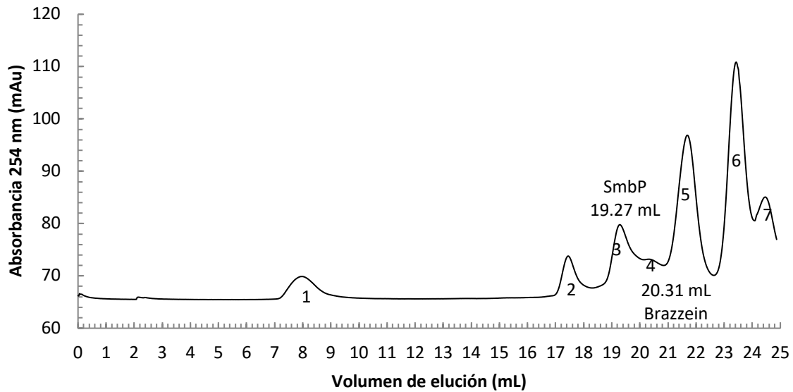
Figura 25. Cromatograma de purificación por exclusión por tamaño de SmbP y Brazzein después de digestión con enteroquinasa. El pico 3 eluyó a los 19.27 mL y el pico 4 a los 20.31 mL.
