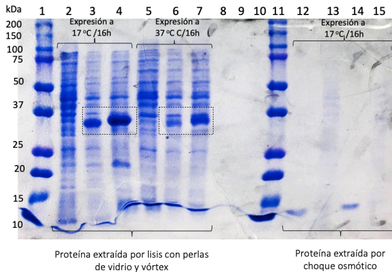
Figura 58. Microexpresión a diferentes condiciones de PelB_SmbP_Brazzein FLEX (31.4 kDa), CusF3H+_Brazzein FLEX (31.68 kDa) y SmbP_Brazzein FLEX (31.4 kDa). Carril 1: marcador de peso molecular, carril 2: control negativo E. coli SHuffle a 17 °C /16 horas/0.1 mM IPTG, carril 3: CusF3H+_Brazzein FLEX, carril 4: SmbP_Brazzein FLEX, carril 5: control negativo E. coli SHuffle a 37 °C /16 horas/0.1 mM IPTG, carril 6: CusF3H+_Brazzein FLEX, carril 7: SmbP_Brazzein FLEX, carril 11: marcador de peso molecular, carril 12: F. Hiper. E. coli BL21(DE3), carril 13: F. Hipo E. coli BL21(DE3), carril 14: F. Hiper PelB_SmbP_Scygonadin FLEX, carril 15: F. Hipo PelB_SmbP_Brazzein FLEX.
