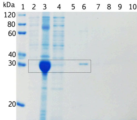
Figura 34. Purificación de CusF3H+_MCL (32.07 kDa) expresada en Origami2(DE3) mediante SDS-PAGE al 12%. Carril 1: Marcador de peso molecular, carril 2: Clarificado, carril 3: Restos celulares después de lisis con perlas de vidrio y lisozima, carril 4: percolado, carril 5: fracción de lavado, carril 6-10: fracciones de elución de CusF3H+_MCL.
