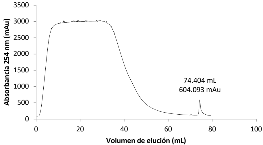
Figura 29. Cromatograma de purificación por afinidad a Ni (II) para CusF3H+_MCL. Solución amortiguadora de lisis y lavado: 50 mM Tris, 500 mM NaCl, solución amortiguadora de elución: 50 mM Tris, 500 mM NaCl, 200 mM imidazol pH 8. El pico de elución se obtuvo a los 74.40 mL de elución con una absorbancia de 604.09 mAu
