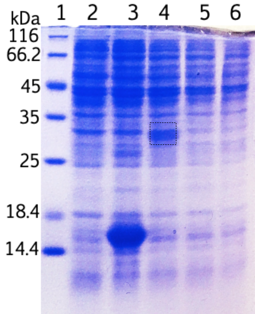
Figura 50. Microexpresión en E. coli SHuffle de tandems con CusF3H+ por SDS-PAGE 15%. Carril 1: marcador de peso molecular, carril 2: control negativo de E. coli SHuffle, carril 3: control positivo de CusF3H+_STOP (10.15), carril 4: CusF3H+_Brazzein3xNG (30.31 kDa), carril 5: CusF3H+_Rattusin2xNG (18.34 kDa), carril 5: CusF3H+_Rattusin3xNG (22.14 kDa).
