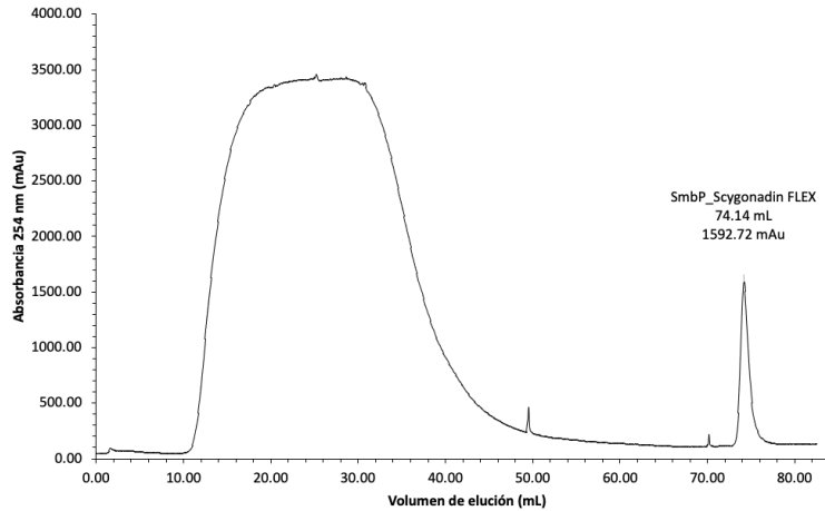
Figura 66. Cromatograma de purificación por afinidad a Ni(II) para SmbP_Scygonadin FLEX. Solución amortiguadora de lisis y lavado: 50 mM Tris, 500 mM NaCl, 5 mM imidazol, pH 8 y solución amortiguadora de elución: 50 mM Tris, 500 mM NaCl, 200 mM imidazol, pH 8.
