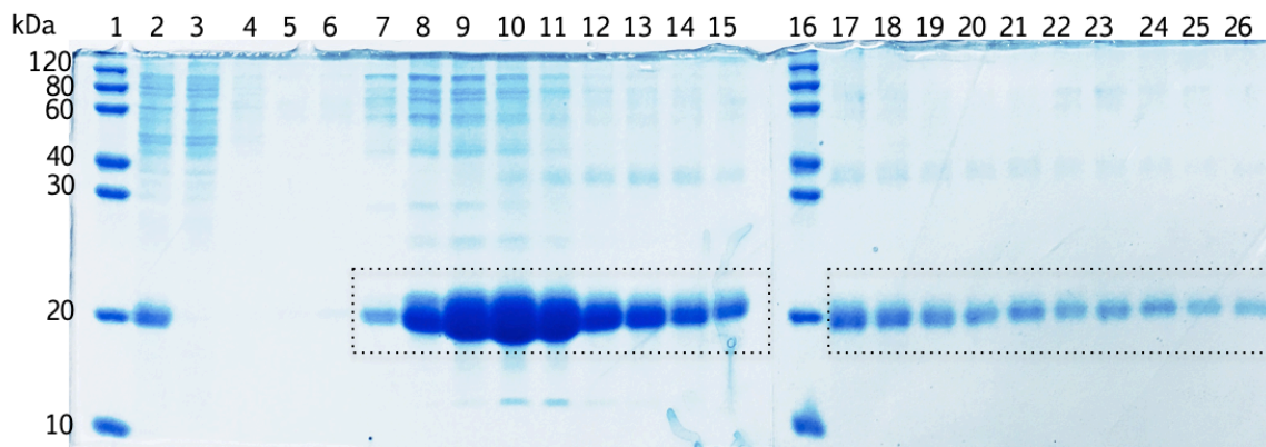
Figura 17. Análisis de fracciones de elución de CusF3H+_Brazzein (17.09 kDa) mediante SDS-PAGE 15%. Carriles 1 y 16: marcador de peso molecular, carril 2: lisado, carril 3: percolado, carriles 4 y 5: lavados, carriles 6-26: fracciones de elución.
