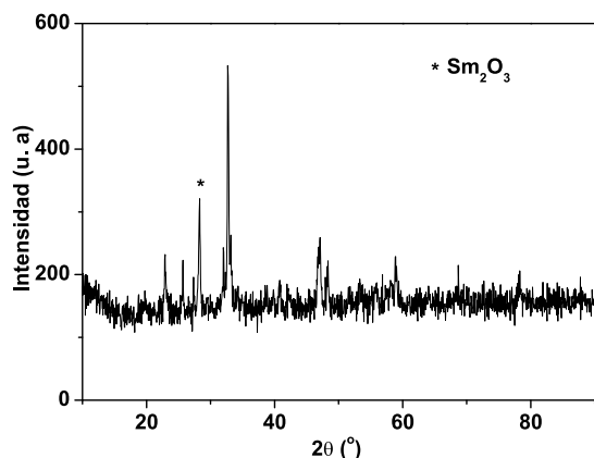
Figura 3. Difractograma del producto SmFeO_3
