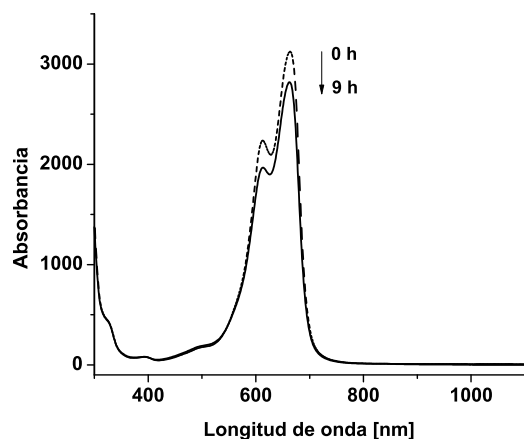
Figura 8. Barrido de máxima absorbancia para el blanco de H_2O_2 .
