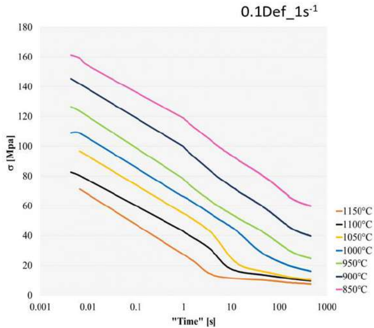
Figura 4. 33. Curvas de ablandamiento del acero experimental. Condiciones de deformación a 0.1\text{Def}_{1\text{s}^{-1}} a temperaturas entre 1150^{\circ}\text{C} y 850^{\circ}\text{C} .
