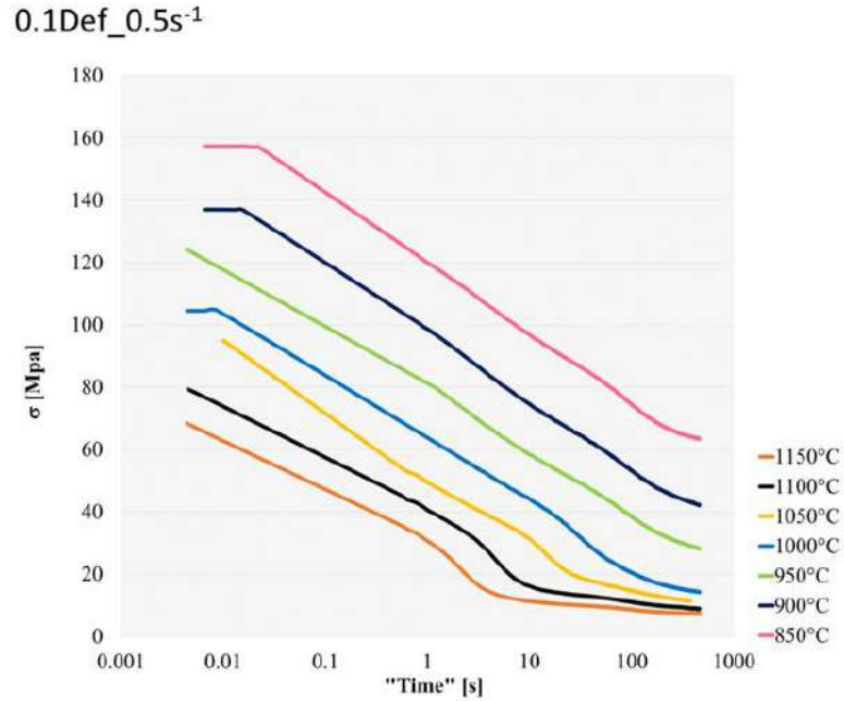
Figura 4. 32. Curvas de ablandamiento del acero experimental. Condiciones de deformación a 0.1\text{Def}_{0.5\text{s}^{-1}} a temperaturas entre 1150^{\circ}\text{C} y 850^{\circ}\text{C} .
