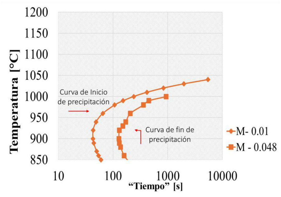
Figura 4. 15. Curva tiempo – temperatura – precipitación en matriz obtenida por simulación por software con JMatPro del acero experimental.
