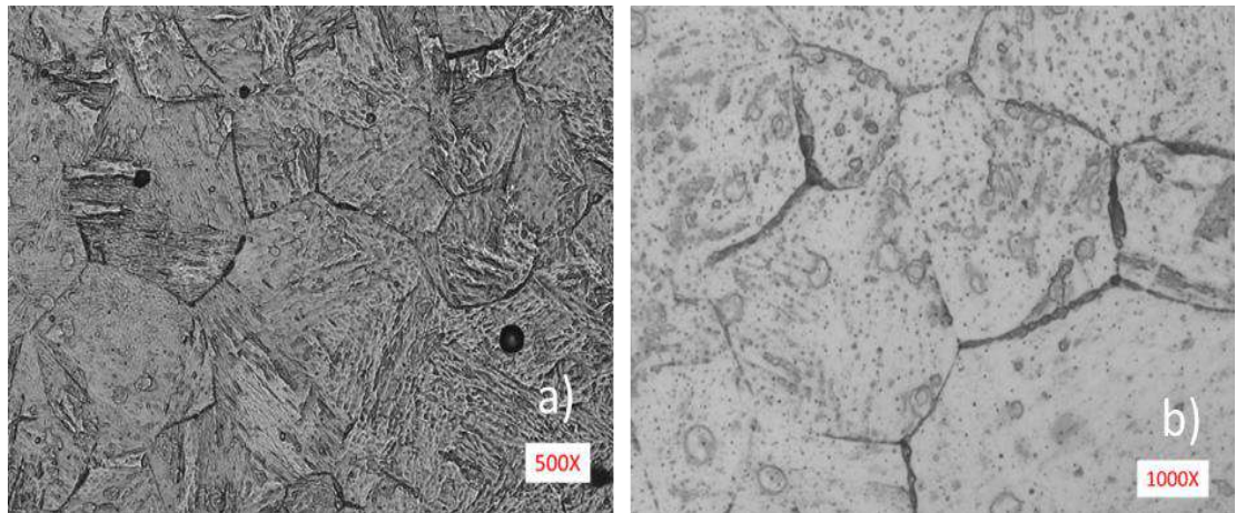
Figura 4. 6. Revelado de tamaño de grano previo a la deformación del Ciclo 2, a 500X y 1000X. Tiempo de ataque de 5 -15 minutos con solución de ácido pícrico sobresaturado y ácido clorhídrico.
