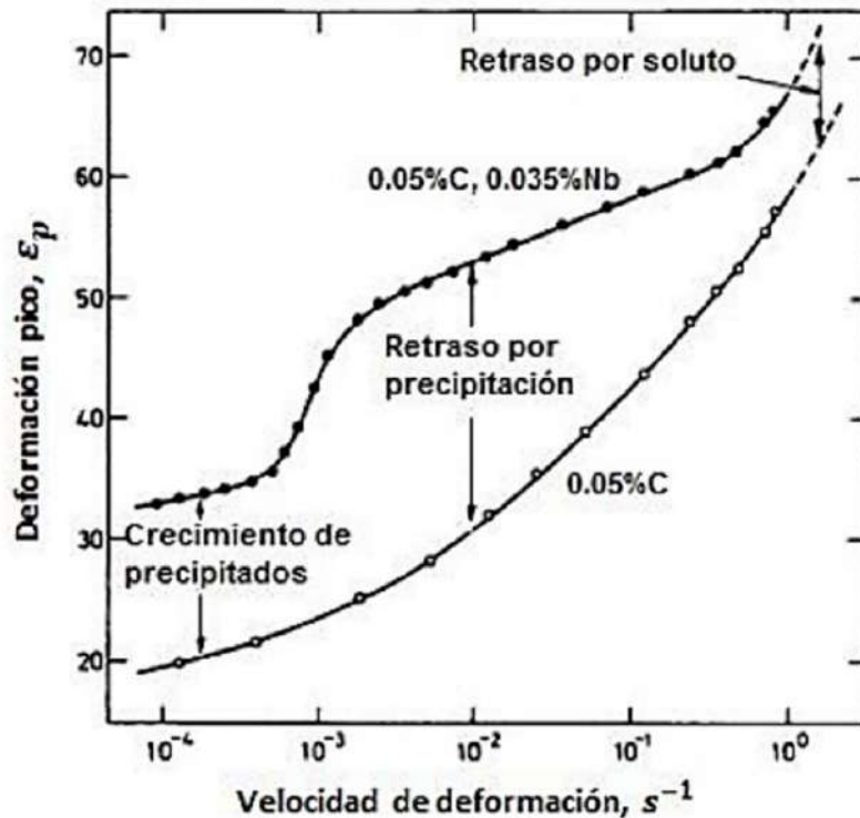
Figura 2. 21. Influencia de los elementos en solución sólida en el retraso de la recristalización dinámica.
