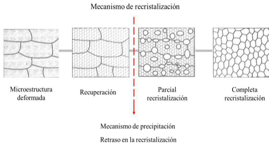
Figura 4. 44. Retraso de la recrystalización efectos de la precipitación inducida por deformación en el acero experimental [128,135,139].
