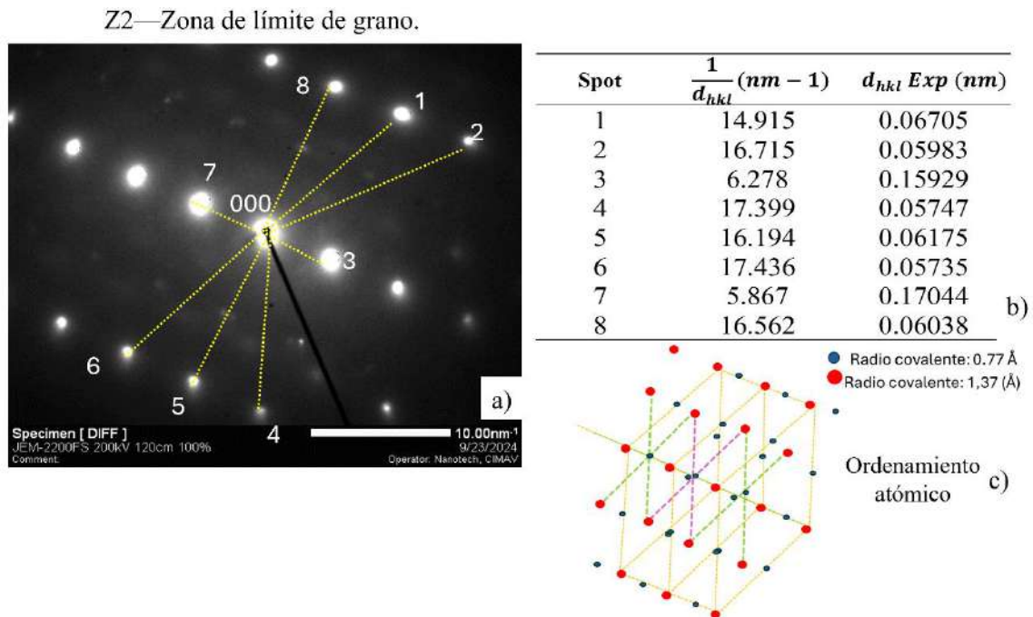
Figura 4. 74. Identificación de la constitución del precipitado inducido por deformación con interfaz coherente con la matriz.
