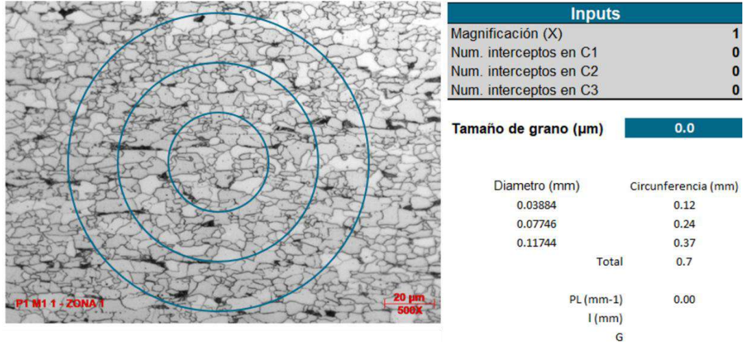
Figura 3. 8. Determinación del tamaño de grano por el método de rejilla patrón.
