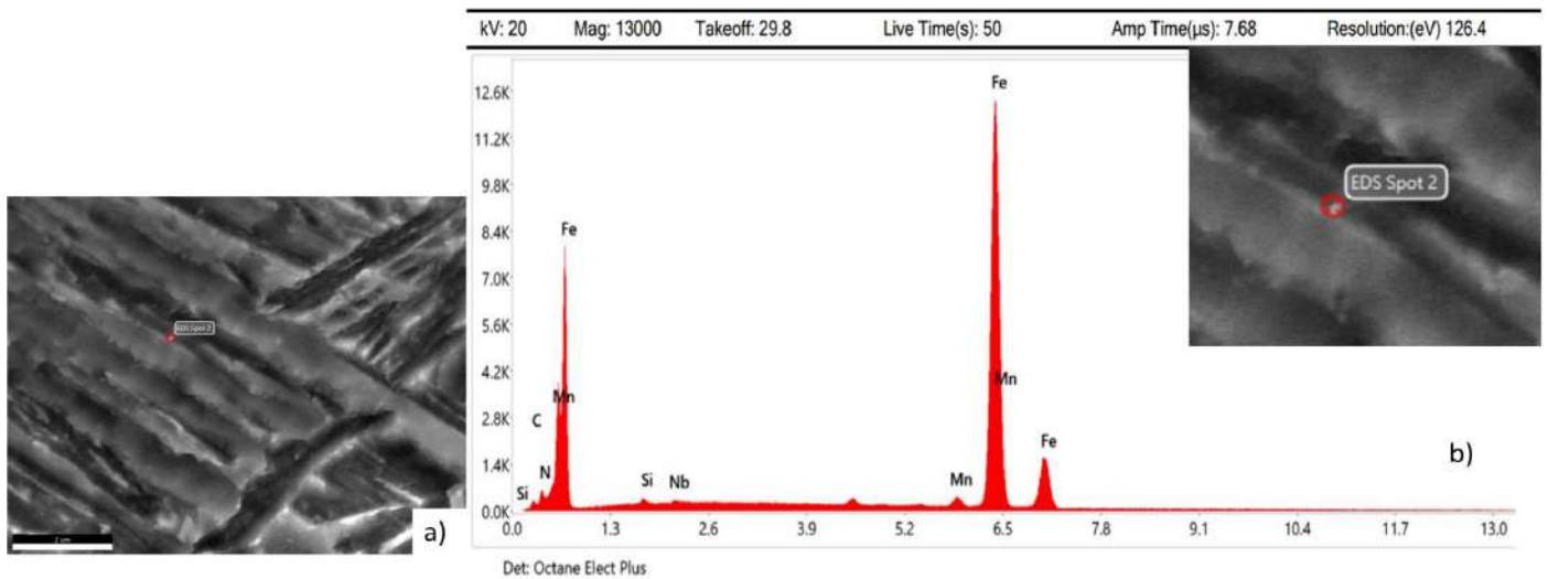
Figura 4. 29. Análisis de EDS a 20kV en zonas con indicios de precipitación. (a) Partícula nanométrica constituida por Nb, C, N. Imagen a 2μm. Nivel de energía L del niobio a 2.166ev, detección desde un voltaje de aceleración de 5kV.
