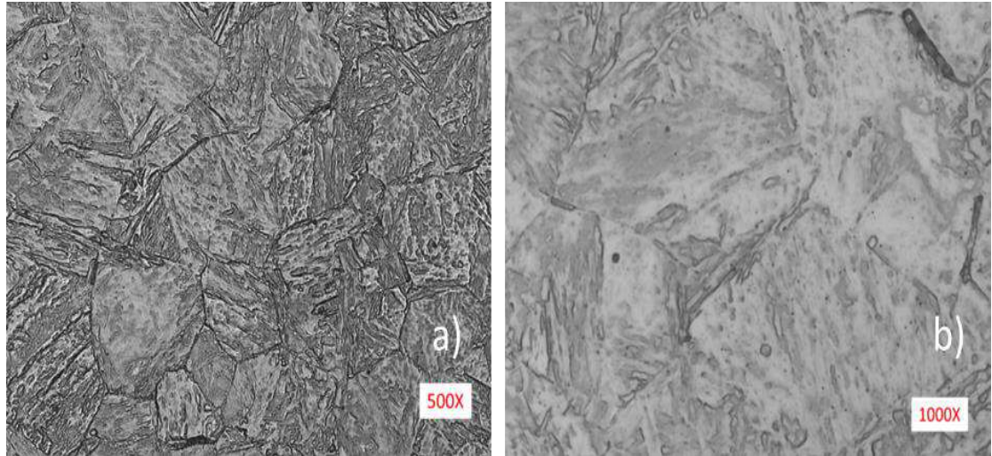
Figura 4. 5. Revelado de tamaño de grano previo a la deformación del Ciclo 1 a 500X y 1000X. Tiempo de ataque de 5-15 minutos con solución de ácido pícrico sobresaturados y ácido clorhídrico.
