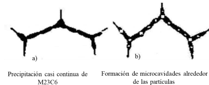
Figura 4. 43. Precipitación de Nb (C, N) o M23C6 (carburo enriquecido de Cr, Mo, V) [58,64,121,145,148].
