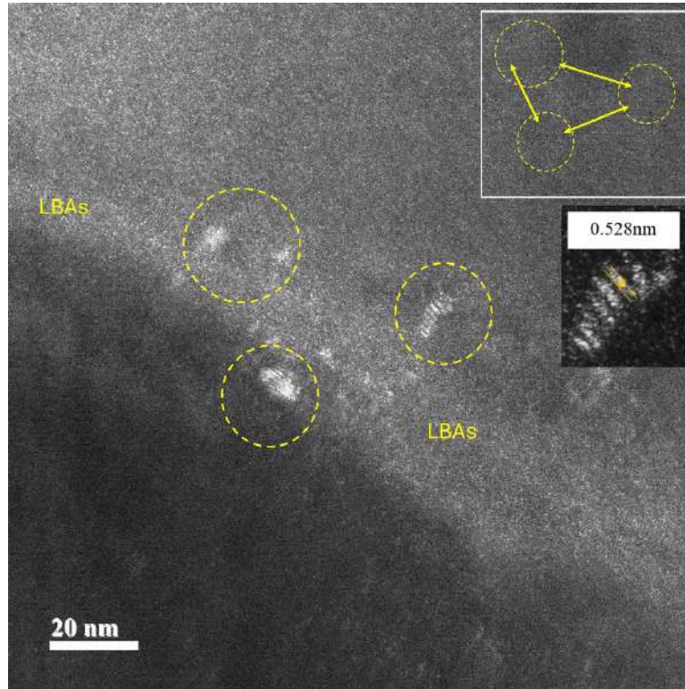
Figura 4. 71. Imágenes de campo obscuro (DF) de la condición 4. a) Nano precipitados de 3 a 5 nm en límite de subestructura. b) y c) Medición del radio atómico en precipitado de alta resolución.
