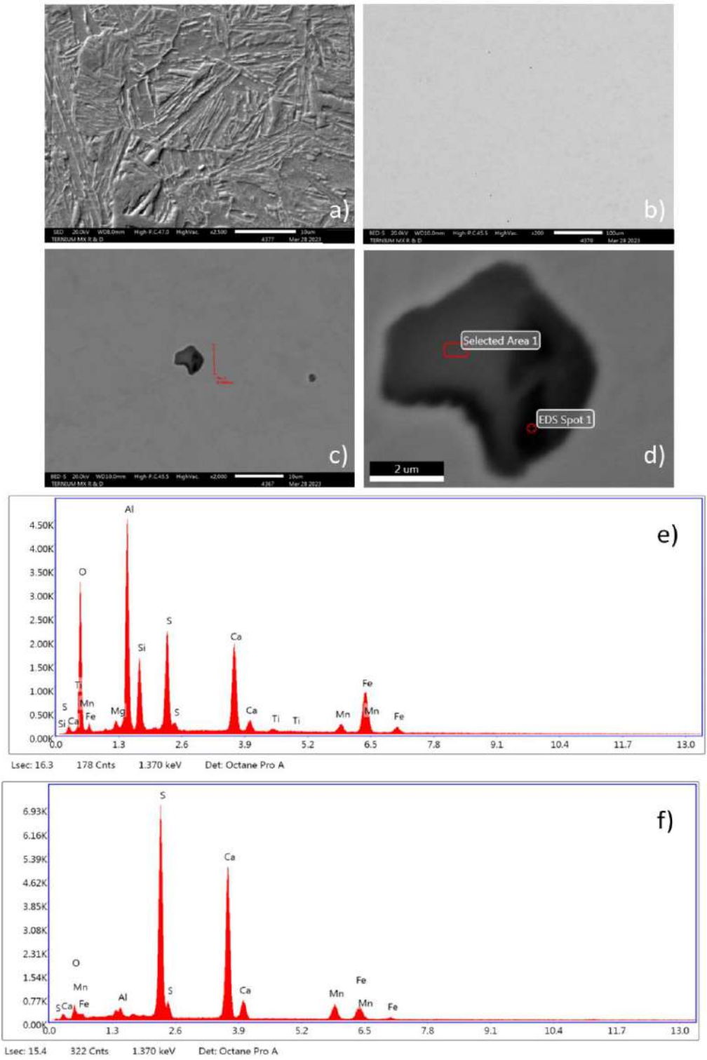
Figura 4. 27. Sulfuros e inclusiones. a) Microestructura revelada con Nital a un 3% a 10 \mu\text{m} . b) Muestra con vibro pulido a 100 \mu\text{m} . c) y d) Análisis de partícula en matriz. e) y f) Análisis por EDS de partícula y matriz.
