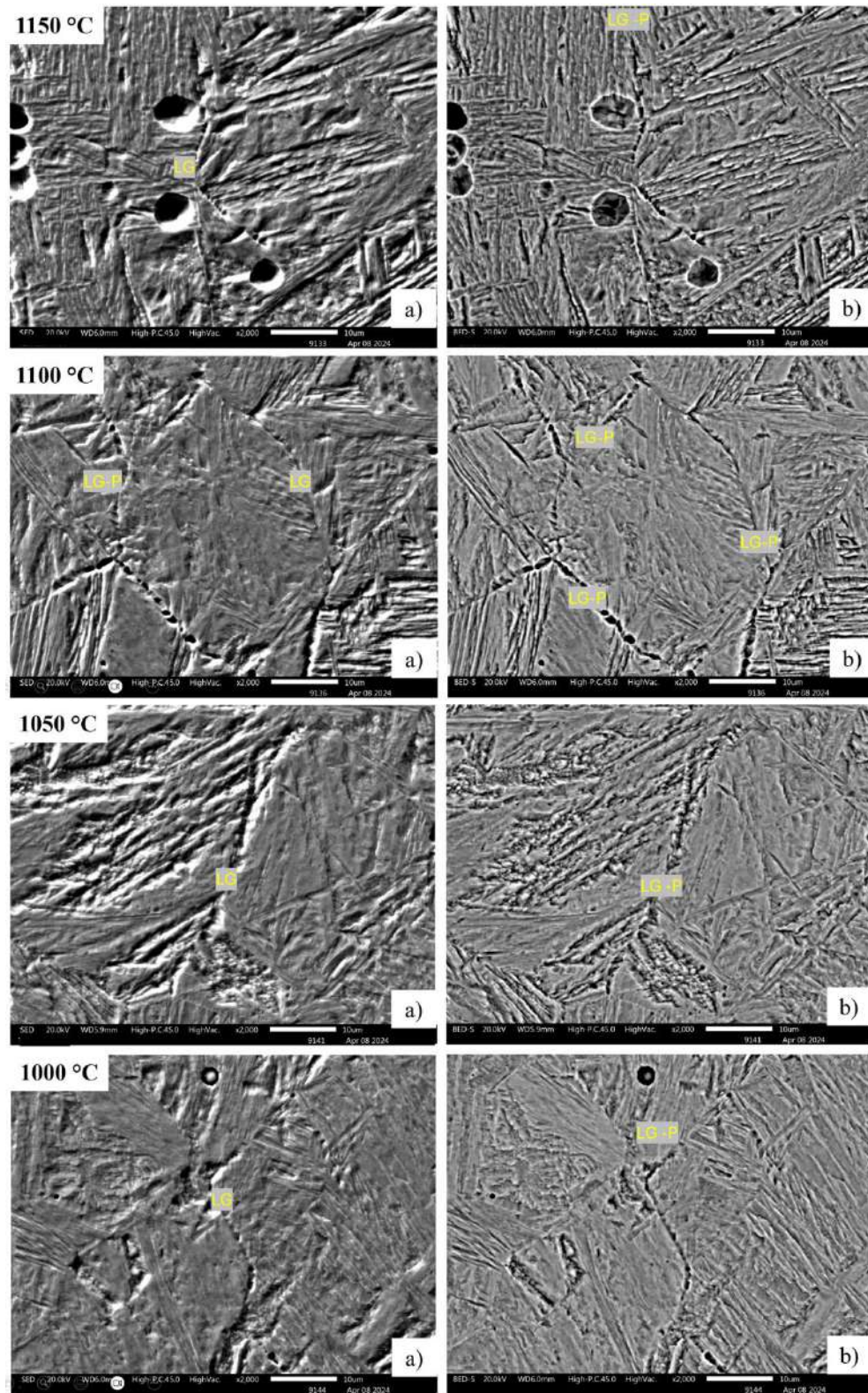
Figura 4. 50. Imágenes de los límites de grano austenítico deformado revelado con solución de ácido pícrico y clorhídrico. A) SED, B) BEDS a 2000x, 0.2 Def_0.5s -1 .
