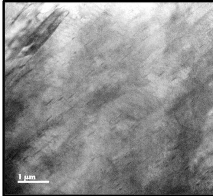
Figura 4. 70. Imagen de campo claro de la condición 4 a 1 μm que representa la interfaz de tipo planar extendida en la matriz del acero.
