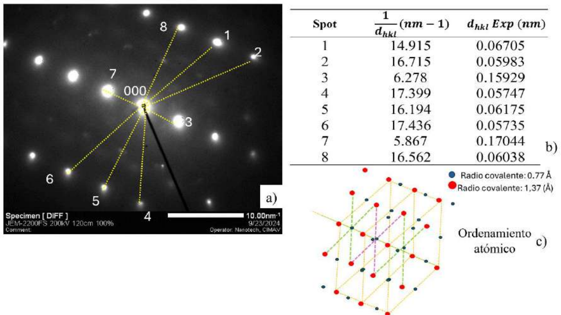
Figura 4. 74. Identificación de la constitución del precipitado inducido por deformación con interfaz coherente con la matriz.
