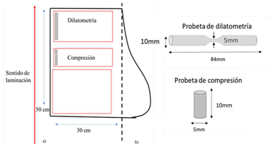
Figura 3. 5. Representación de, a) Barra de transferencia. b) Dimensiones de probetas de dilatometría y compresión.
