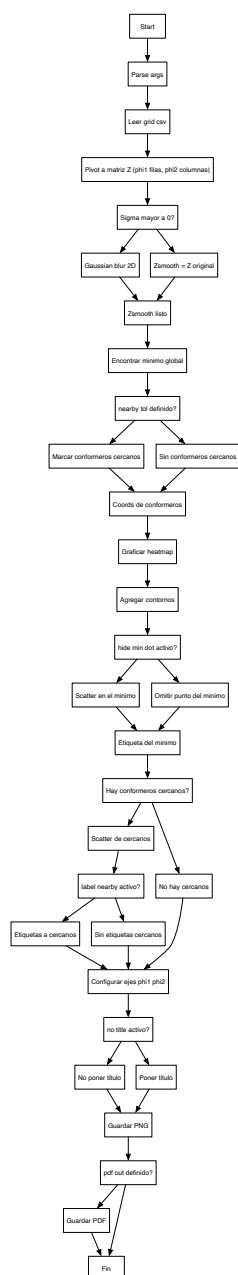
Figura A.14.: Diagrama de flujo del script rss.py para la generación de gráficas de Ramachandran.
