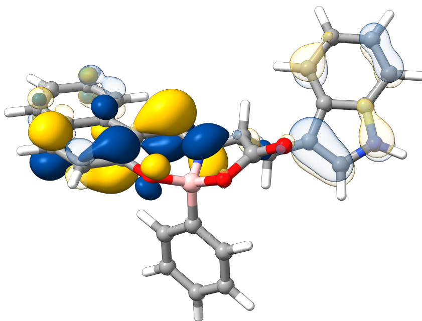
Figura 8.23.: NTO correspondientes a las transiciones más significativas en la excitación al estado S_3 de BO(W) 1c elongado en DMSO. 115a \rightarrow 116a : n = 97.61\% . Isovalor de 0.045. Se muestra la partícula como una isosuperficie sólida y el hueco como una isosuperficie semitransparente.
