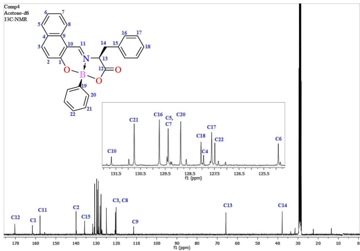
Figura A.5.: Espectro de 13 C-NMR de 11-bencilo-8-fenil-8H-8λ 4 ,12λ 4 -nafto[1,2-e][1,3,2]oxazaborolo[2,3-b][1,3,2]oxazaborinin-10(11H)-ona (BO(F) 1b) en Acetona-d 6 .
