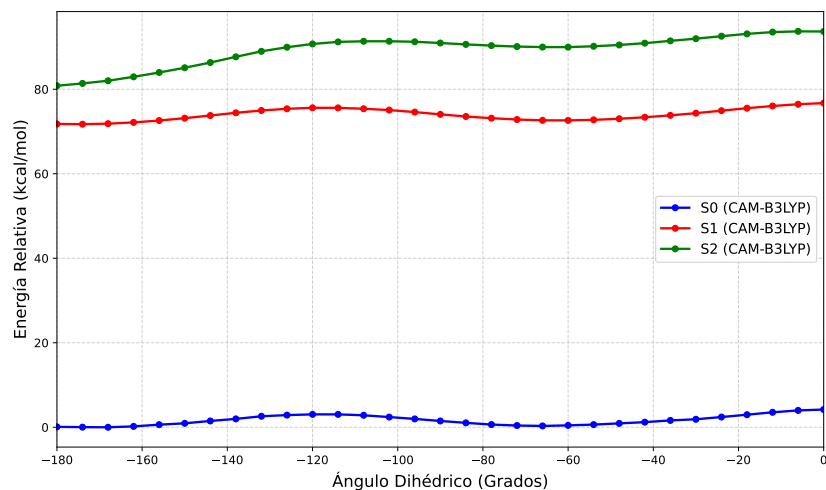
Figura 8.29.: Comparación en energía de las diferentes conformaciones de la molécula de 11-((1 H -indol-3-il)metil)-8-fenil-8 H -8 \lambda^4 ,12 \lambda^4 -nafto[1,2- e ]-[1,3,2]oxazaborolo[2,3- b ][1,3,2]oxazaborinin-10(11 H )-ona 1c en DMSO al rotar el motivo de Trp.
