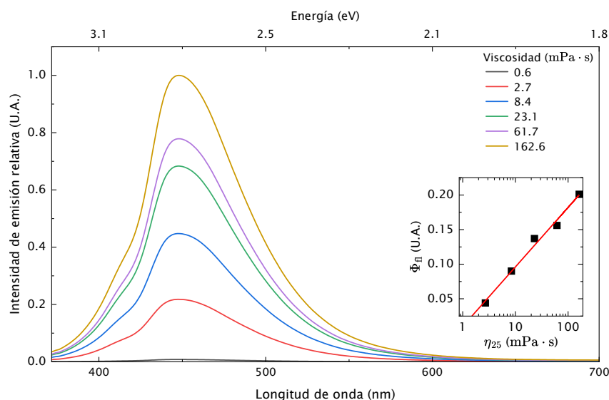
Figura 8.6.: Efecto del aumento de la viscosidad en \Phi_f en BO(W) 1c . Se aprecia un incremento en el rendimiento cuántico de fluorescencia, \Phi_f relativo al incrementar la fracción volumétrica de glicerol en la mezcla. La respuesta en el incremento de \Phi_f tiene un comportamiento logarítmico con la viscosidad del medio.
