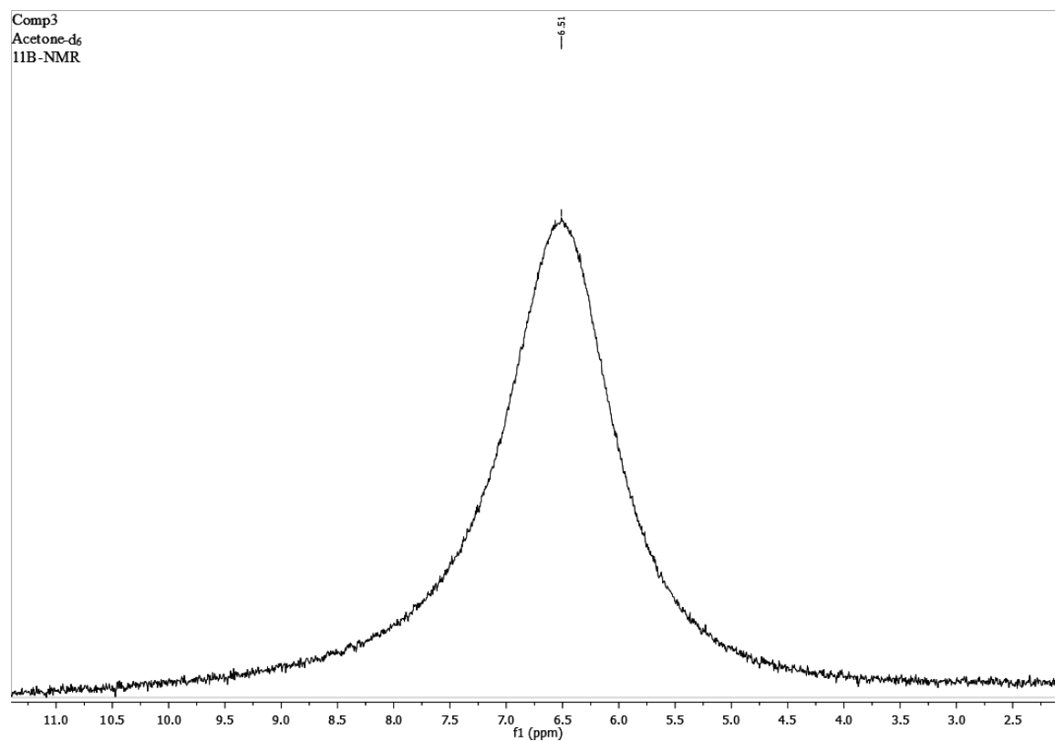
Figura A.12.: Espectro de ^{11}\text{B} -NMR de 11-(4-hidroxibencilo)-8-fenil-8 \lambda^4 ,12 \lambda^4 -nafto[1,2- e ][1,3,2]oxazaborolo[2,3- b ][1,3,2]oxazaborinin-10(11 H )-ona (BO(Y) 1d) en DMSO- d_6 .
