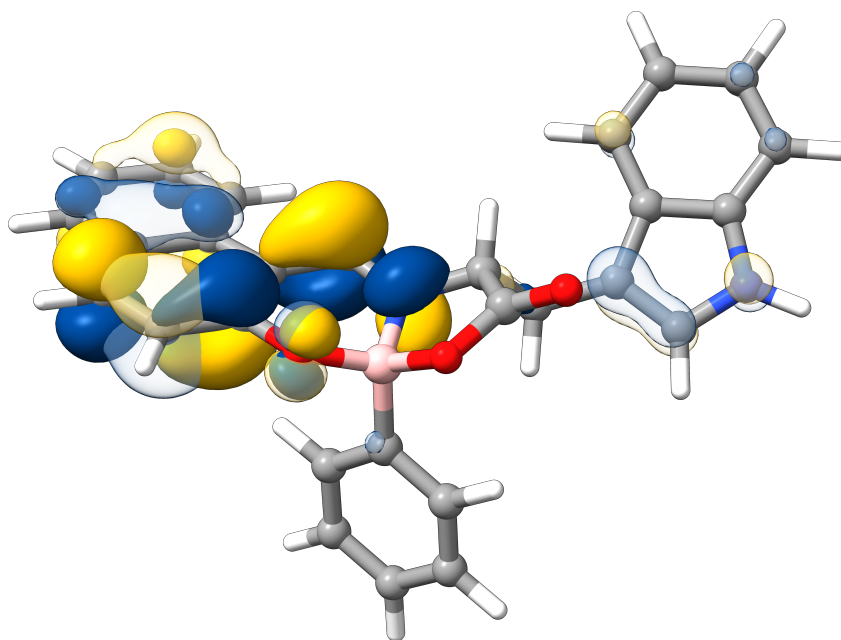
Figura 8.22.: NTO correspondientes a las transiciones más significativas en la excitación al estado S_2 de BO(W) 1c elongado en DMSO. 115a \rightarrow 116a : n = 94.39\% . Isovalor de 0.045. Se muestra la partícula como una isosuperficie sólida y el hueco como una isosuperficie semitransparente.
