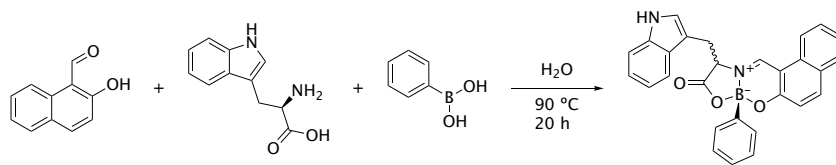
Esquema 7.4.: Síntesis de 11-((1 H -indol-3-il)metil)-8-fenil-8 H -8 \lambda^4 ,12 \lambda^4 -nafto[1,2- e ][1,3,2]oxazaborolo[2,3- b ][1,3,2]oxazaborinin-10(11 H )-ona, BO(W) 1c .
