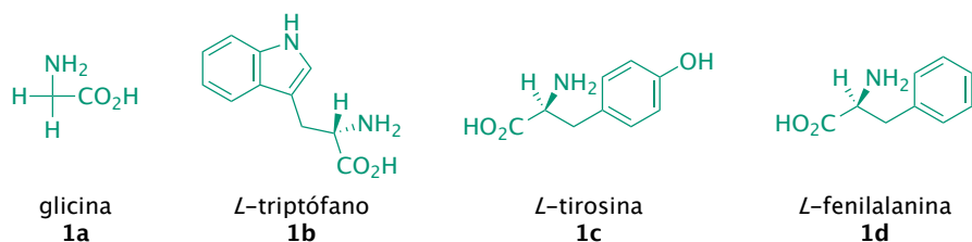
Esquema 7.2.: Estructuras de los \alpha -aminoácidos utilizados.
