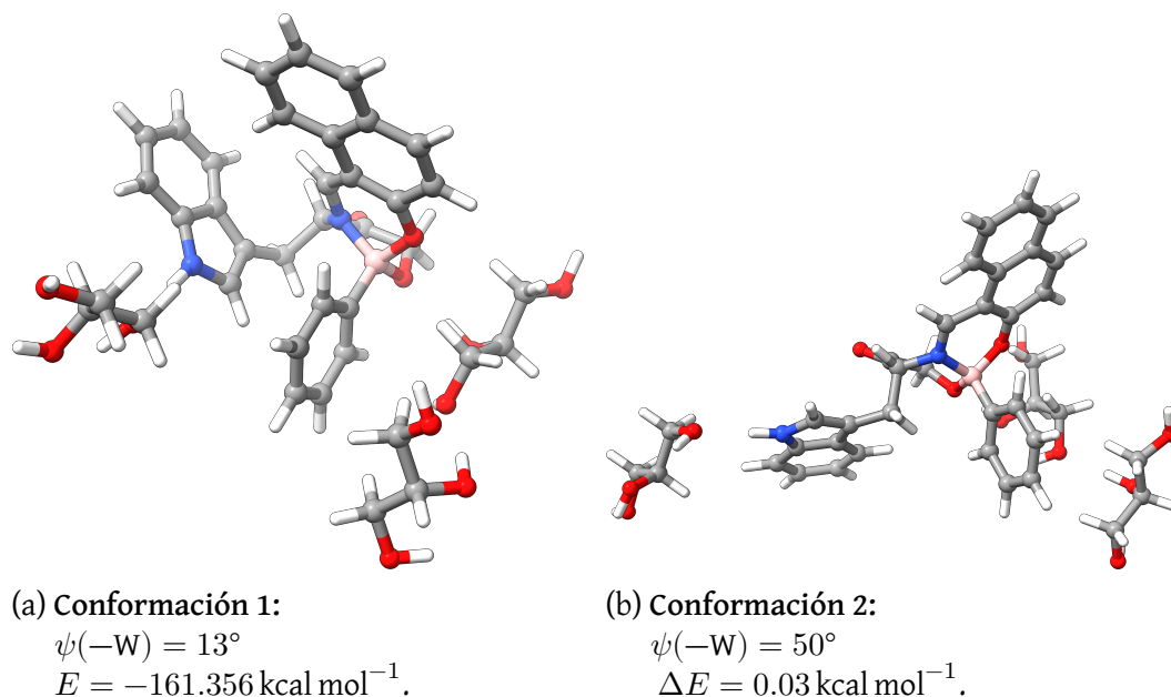
Figura 8.20.: Estructuras de BO(W) con glicerol explícito, optimizadas en GFN2-xTB con solvatación implícita de DMSO.
