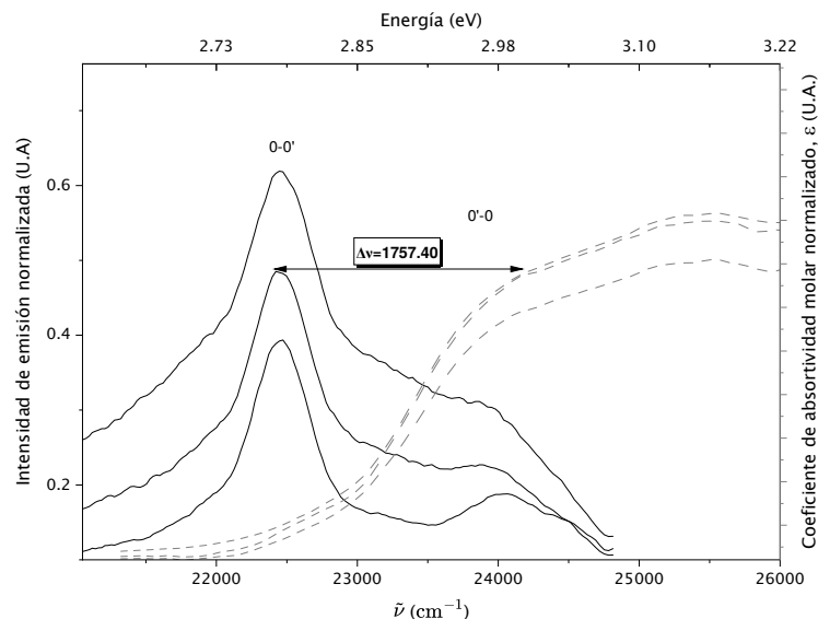
Figura 8.9.: Espectro de fluorescencia y de absorbancia molecular de BO(W) 1c en MeCl 3 . \lambda_{\text{EX}} = 411 \text{ nm} , \lambda_{\text{EM}} = 454 \text{ nm} , c_{\text{M}} = 1.5326 \times 10^{-5} \text{ nmol mL}^{-1} , anchura de ranura de entrada: 5.00 nm paso de banda; Anchura de ranura de salida: 5.00 nm; tiempo de integración: 0.1 s.
