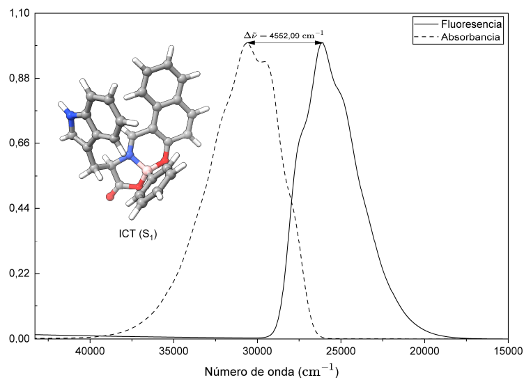
Figura 8.41.: Espectro de fluorescencia y de absorción para la conformación ICT de BO(W) 1c.
