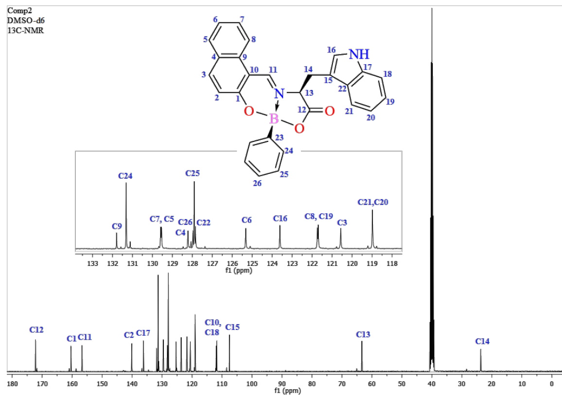
Figura A.8.: Espectro de 13 C-NMR de 11-((1H-indol-3-il)metil)-8-fenil-8H-8λ 4 ,12λ 4 -nafto[1,2-e][1,3,2]oxazaborolo[2,3-b][1,3,2]oxazaborin-10(11H)-ona (BO(W) 1c) en DMSO-d 6 .
