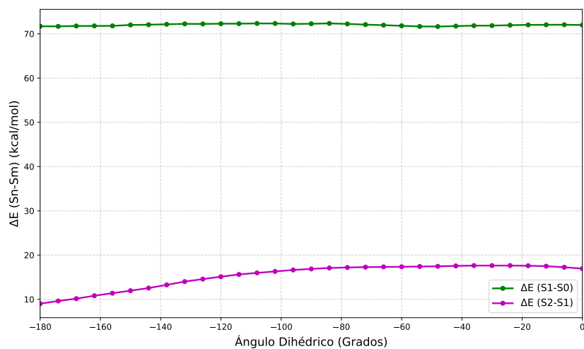
Figura 8.30.: Comparación en energía de los estados excitados de las diferentes conformaciones de la molécula de 11-((1 H -indol-3-il)metil)-8-fenil-8 H -8 \lambda^4 ,12 \lambda^4 -nafto[1,2- e ][1,3,2]oxazaborolo[2,3- b ][1,3,2]oxazaborinin-10(11 H )-ona 1c en DMSO al rotar el motivo de Trp.
