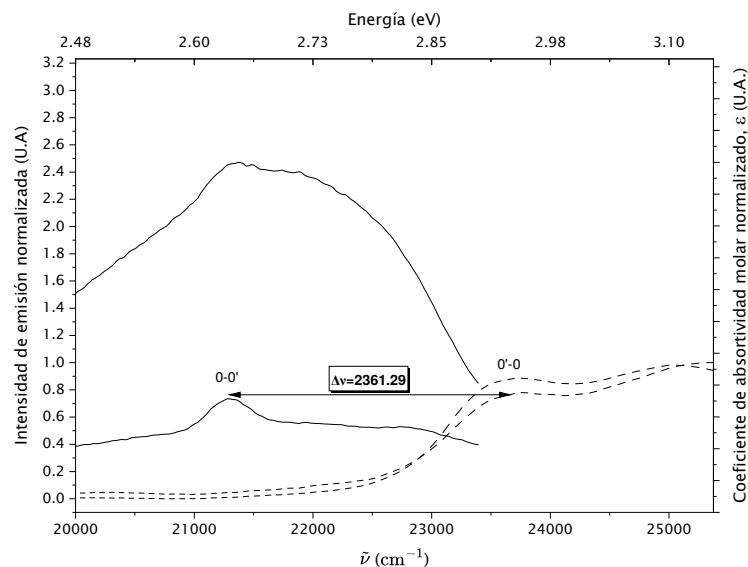
Figura 8.11.: Espectro de fluorescencia y de absorbancia molecular de BO(W) 1c en Dioxano. \lambda_{EX} = 413 nm, \lambda_{EM} = 470 nm, c_M = 1.66925 \times 10^{-5} nmol mL -1 , anchura de ranura de entrada: 5.00 nm paso de banda; Anchura de ranura de salida: 5.00 nm; tiempo de integración: 0.1 s.
