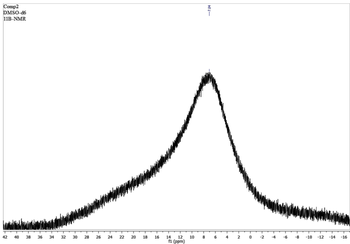
Figura A.9.: Espectro de ^{11}\text{B} -NMR de 11-((1 H -indol-3-il)metil)-8-fenil-8 H -8 \lambda^4 ,12 \lambda^4 -nafto[1,2- e ][1,3,2]oxazaborolo[2,3- b ][1,3,2]oxazabori- nin-10(11 H )-ona (BO(W) 1c) en DMSO- d 6 .
