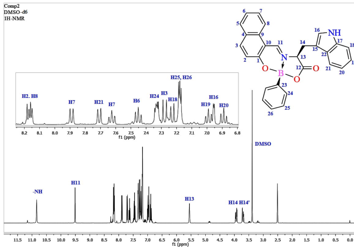
Figura A.7.: Espectro de 1 H-NMR de 11-((1H-indol-3-il)metil)-8-fenil-8H-8λ 4 ,12λ 4 -nafto[1,2-e][1,3,2]oxazaborolo[2,3-b][1,3,2]oxazaborin-10(11H)-ona (BO(W) 1c) en DMSO-d 6 .
