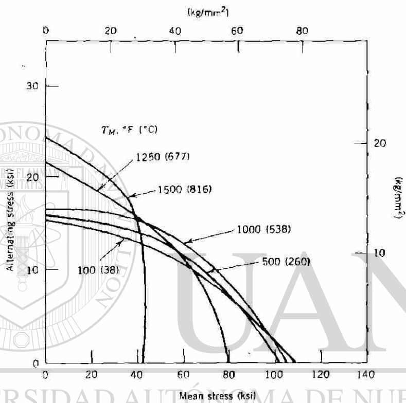
2.) Diagrama típico de Goodman, para un álabe de aleación base níquel con 10E9 ciclos.
