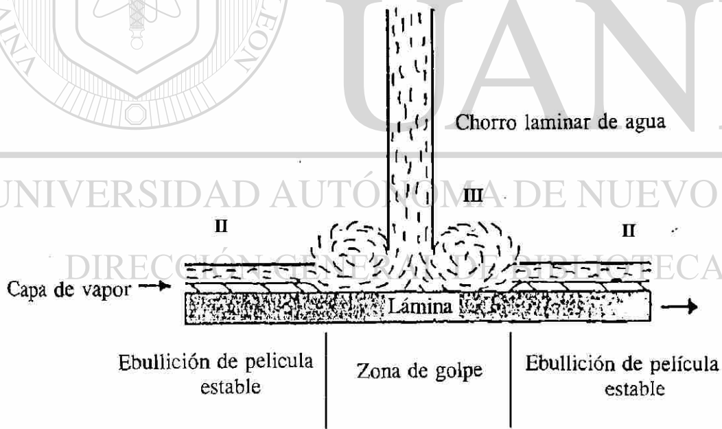
Fig. 4.2.- Zonas de enfriamiento producidas en la superficie superior de la lámina durante su enfriamiento. (R. Colás and C. M. Sellars: Accelerated Cooling of Rolled Steel, Winnipeg, Canadá, 1987)
