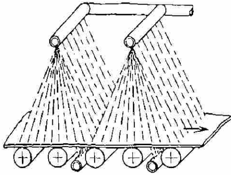
Fig. 2.5.- Sistema de enfriamiento que utiliza cabezales tipo espreas. [2.8]
