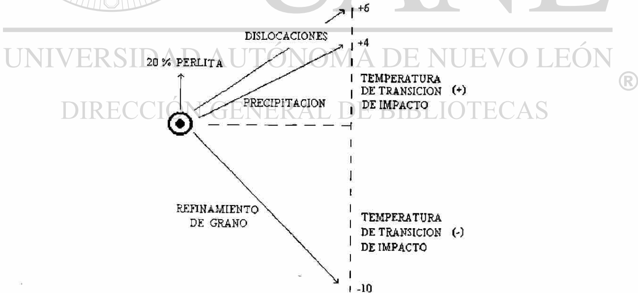
Fig. 3.10.- Factores estructurales que afectan la tensión de fluencia y la temperatura de transición de impacto en aceros ferríticos-perlíticos. [3.5]
