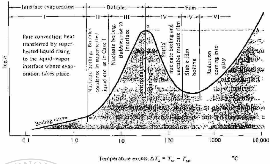
Fig. 4.1.- Flujo de calor en la superficie de un alambre de platino calentado eléctricamente. (Farber and Scoriah: Trans. ASME, vol. 70, p. 369, 1948)
