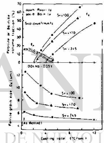
Fig. 3.4.- Cambios de la microestructura transformada con la velocidad de enfriamiento después del laminado controlado en un acero 0.10% C-1.50% Mn-0.04% Nb-0.09% V. [3.11]
