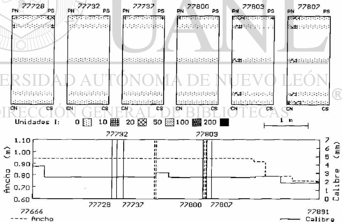
Fig. 5.1. Detalles de planeza en rollos laminados el 4 de mayo de de 1993.
