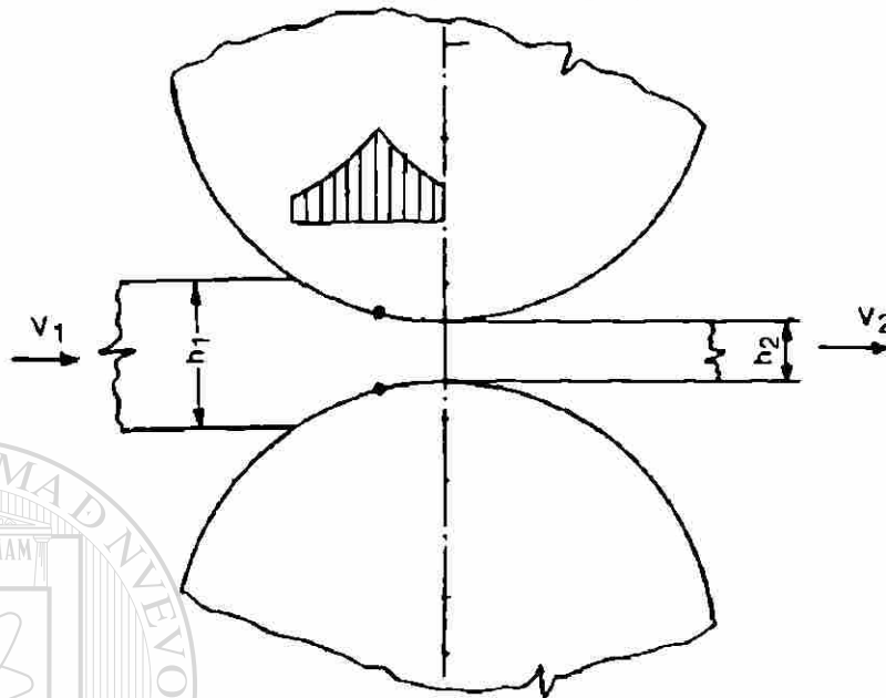
Fig. 2.5 Representación esquemática de la reducción en un pase.
