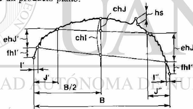
Fig. 2.1 Perfil de un producto plano.
