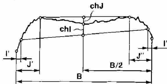
Fig. 2.2 Definición de perfil: a) Corona central y parcial con signos iguales y b) Corona central y parcial con signos opuestos.
