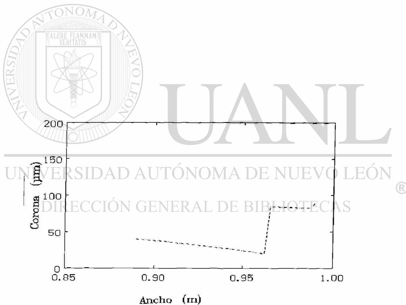
Fig. 5.27 Variación del coronamiento mecánico en una lámina de 93.98 centímetros según se descentre un máximo de cinco cm. a cada lado.
