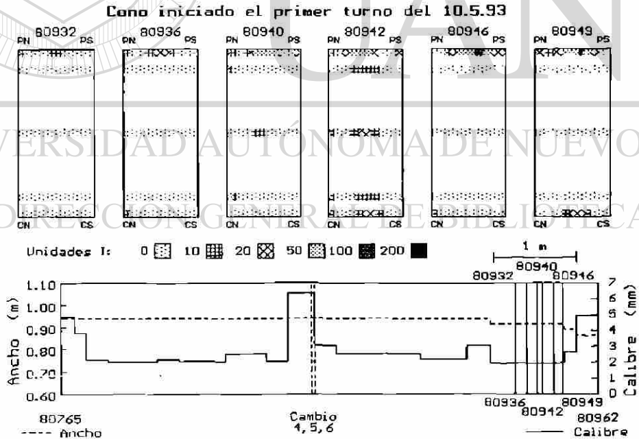
Figura 5.3. Posición de las secuencias a las que se les midió planeza a lo largo del cono laminado el primer turno del 10 de mayo de 1993.
