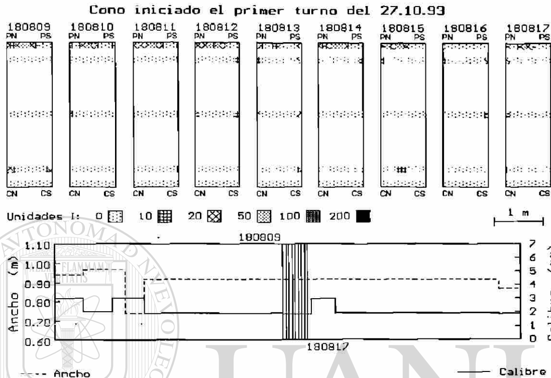
Figura 5.13 Posición de las secuencias a las que se les midió planeza a lo largo del cono de prueba.
