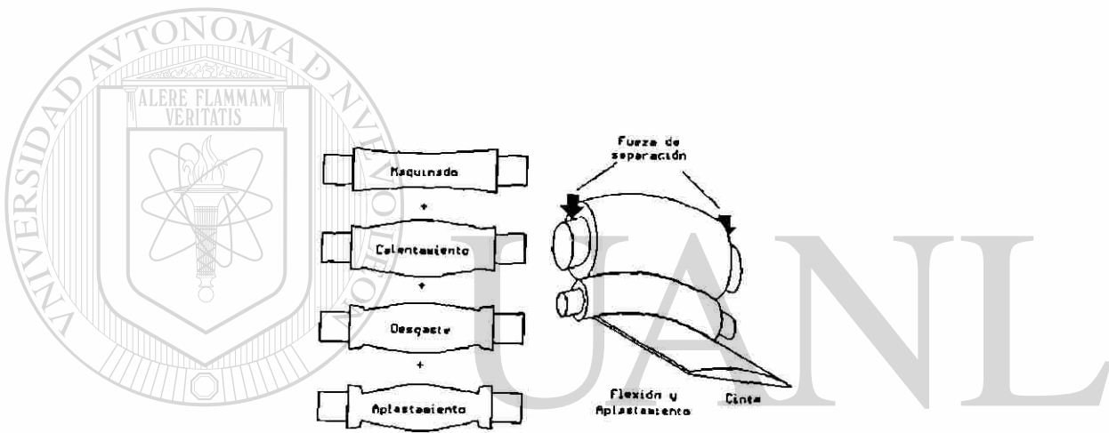
Fig. 3.1 Fenómenos que afectan el perfil de los rodillos de trabajo.
