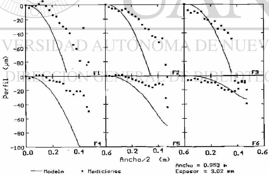
Figura 5.8 Comparación entre los perfiles medidos y predichos para la secuencia 83127.
