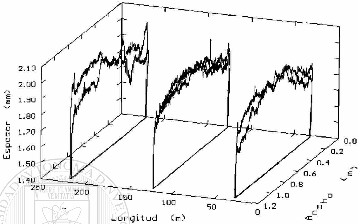
Fig. 5.17 Variación del perfil de la lámina a lo largo de la secuencia 180814.
