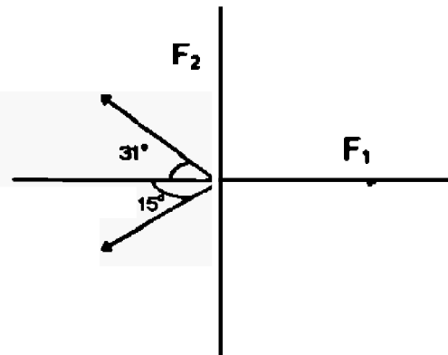
FIGURA 3.8 DIAGRAMA DE FUERZAS CASO 3
