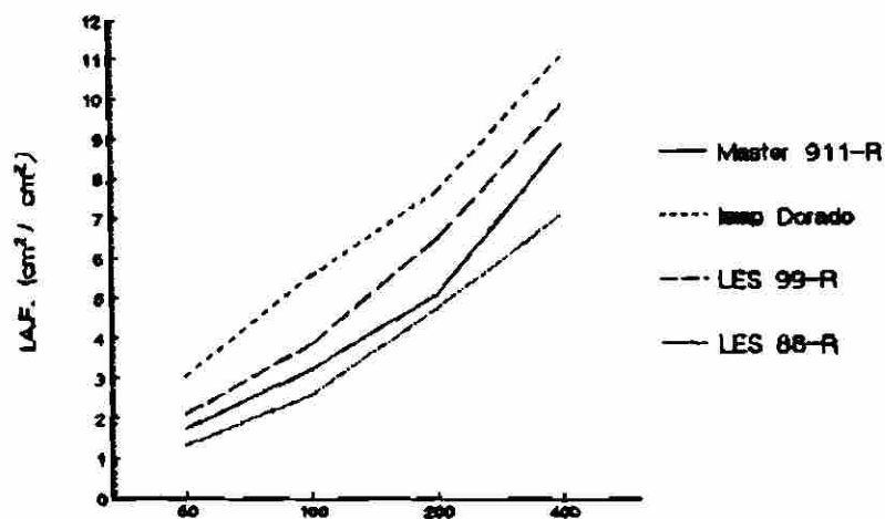
Densidades de población (miles pl/ha) Figura 53. LAF. en cuatro genotipos de sorgo a cuatro densidades de población M.V. 87.
