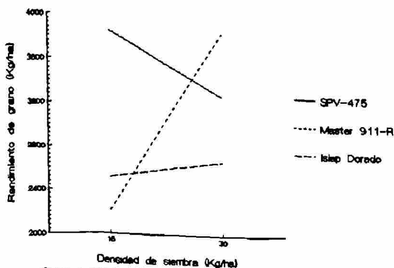
Figura 4. Rendimiento de grano en tres genotipos de sorgo a dos densidades de siembra S.N.P. 88.
