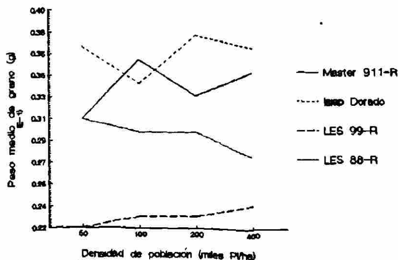
Figura 8. Peso medio de grano en cuatro genotipos de sorgo a cuatro densidades de población M.V. 87.
