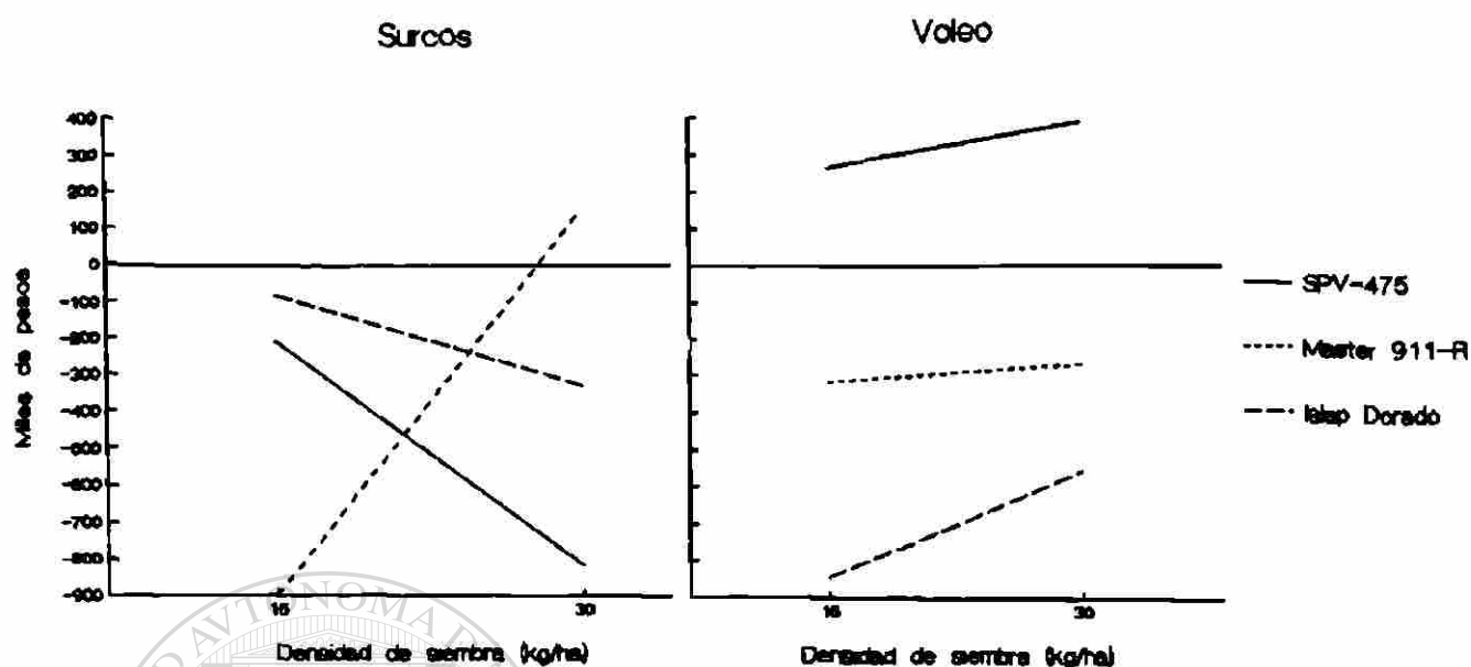
Figura 68. Rend. Econ. neto/ha/ciclo, por venta de grano para tres genotipos de sorgo a dos Dens. de siembra en cada método de siembra SNP. 88
