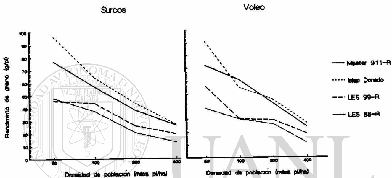
Figura 58. Rendimiento de grano / pl en cuatro genotipos de sorgo a cuatro densidades de población en cada método de siembra M.V. 87.
