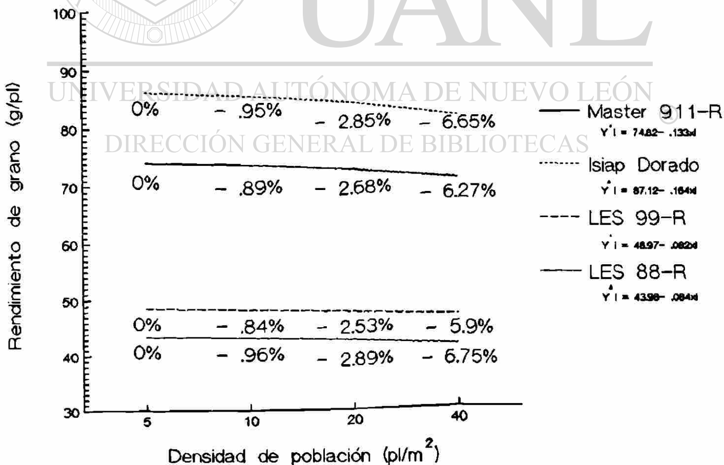
Figura 63. Rend. de grano por pl y su % de reducción en cuatro genotipos de sorgo a cuatro densidades de población M.V. 87.
