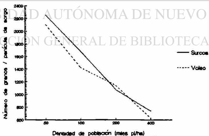
Figura 10. Número de granos por panícula de sorgo en dos métodos de siembra a cuatro densidades de población M.V. 87.
