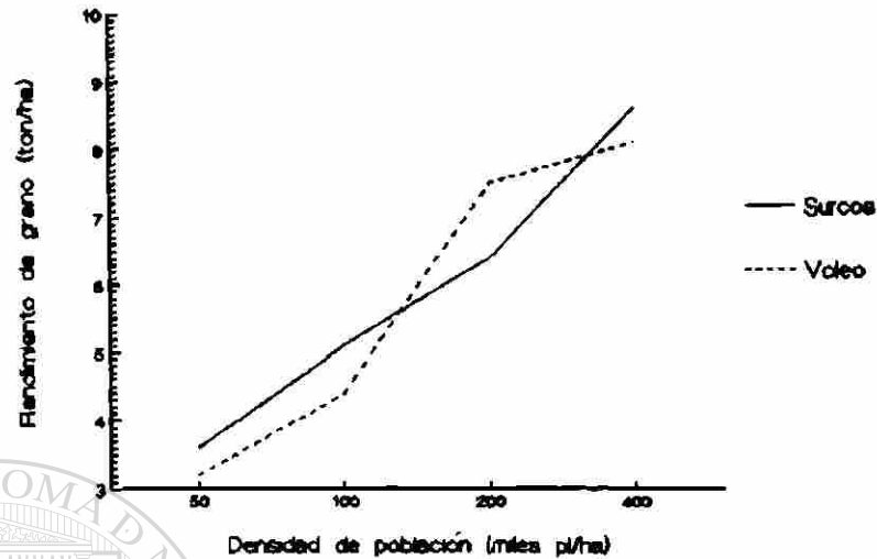
Figura 1. Rendimiento de grano en dos métodos de siembra a cuatro densidades de población M.V. 87.
