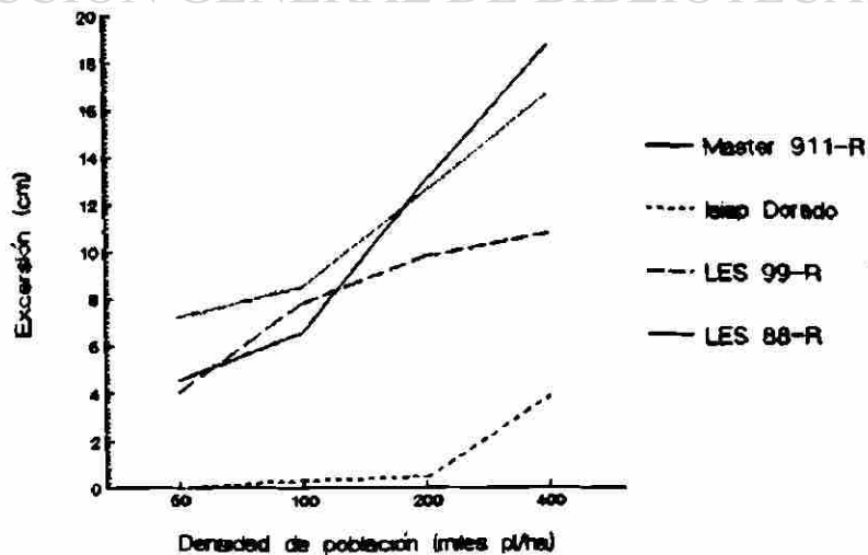
Figura 30. Excersión en cuatro genotipos de sorgo a cuatro densidades de población M.V. 87.
