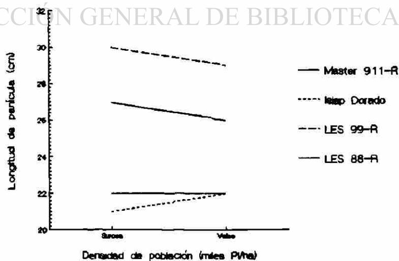
Figura 21. Longitud de panícula en cuatro genotipos de sorgo en dos métodos de siembra M.V. 87.
