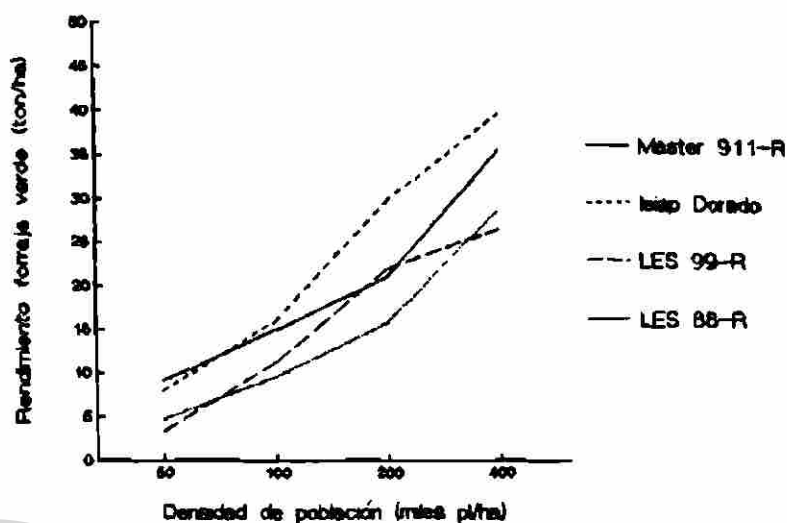
Figura 71. Rendimiento de forraje verde por ha en cuatro genotipos de sorgo a cuatro densidades de población M.V. 87.
