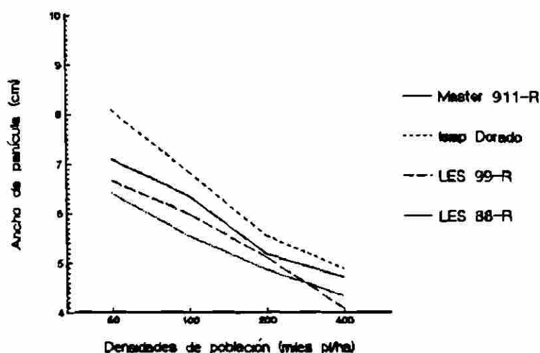
Figura 26. Ancho de panícula en cuatro genotipos de sorgo a cuatro densidades de población M.V. 87.
