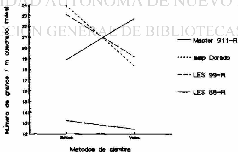
Figura 15. Número de granos / m cuadrado en cuatro genotipos de sorgo en dos métodos de siembra M.V. 87.
