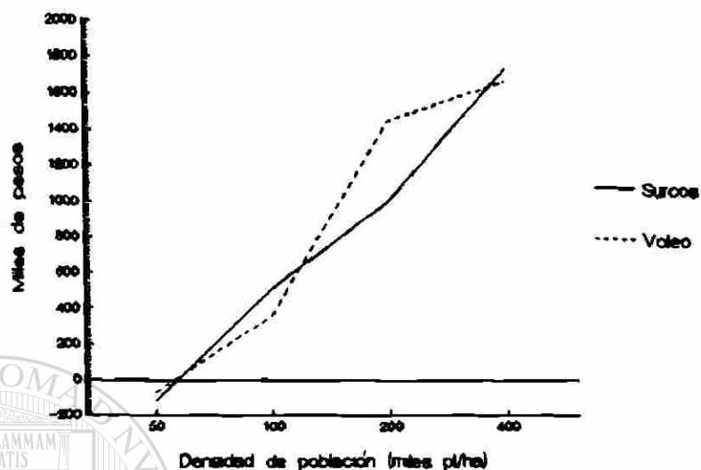
Figura 64. Rend Econ. neto/ha/ciclo, por venta de grano en dos métodos de siembra a cuatro densidades de población MV. 87.
