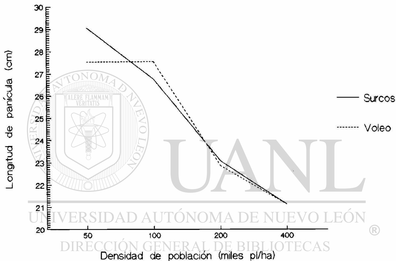
Figura 20. Longitud de panícula en dos métodos de siembra a cuatro densidades de población M.V. 87.
