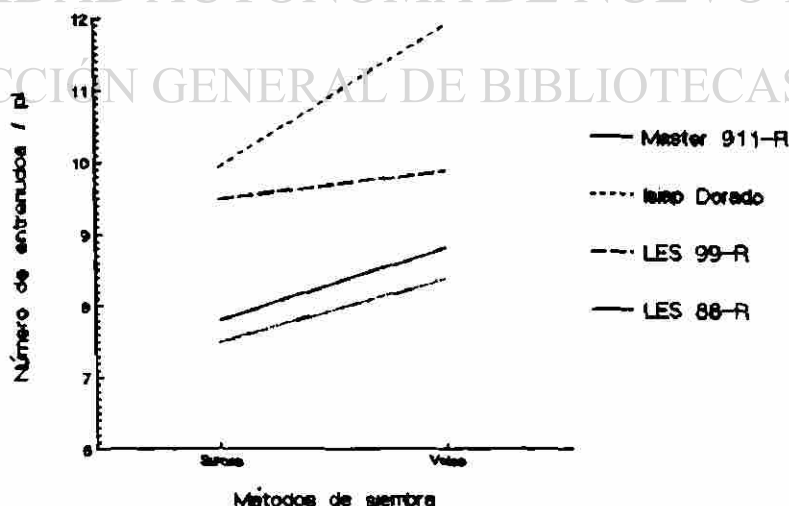
Figura 33. Número de entrenudos / pl en cuatro genotipos de sorgo en dos métodos de siembra M.V. 87.
