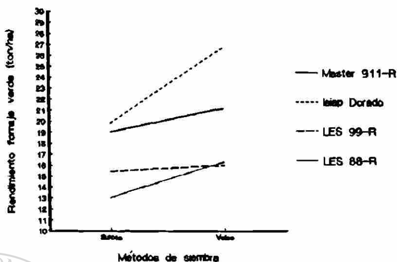
Figura 70. Rendimiento de forraje verde por ha para cuatro genotipos de sorgo en dos métodos de siembra M.V. 87.
