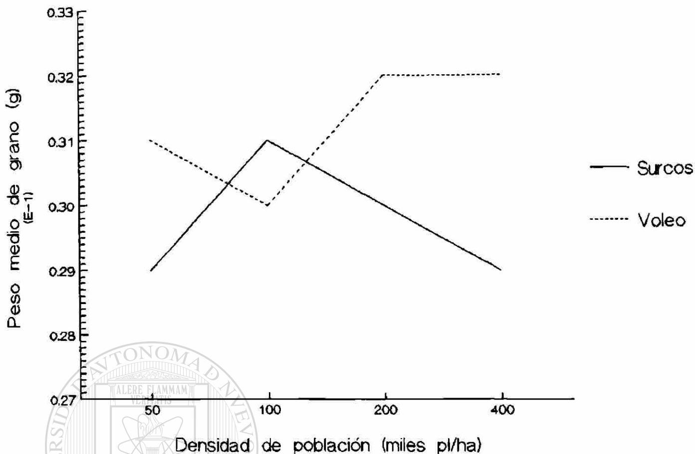
Figura 6. Peso medio de grano en dos métodos de siembra a cuatro densidades de población M.V. 87.
