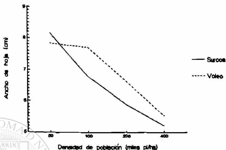
Figura 46. Ancho de hoja en dos métodos de siembra a cuatro densidades de población M.V. 87.
