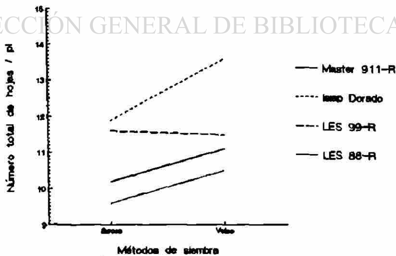
Figura 50. Número total de hojas / pl en cuatro genotipos de sorgo en dos métodos de siembra M.V. 87.
