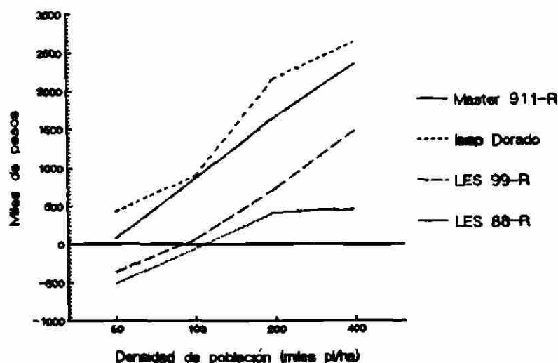
Figura 56. Rend. económico neto/ha/ciclo, por venta de grano para cuatro genotipos de sorgo a cuatro densidades de población M.V. 87.
