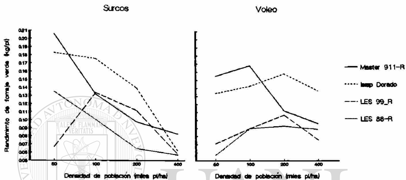
Figura 62. Rend. individual de forraje verde en cuatro genotipos de sorgo a cuatro densidades de población en cada método de siembra M.V. 87.
