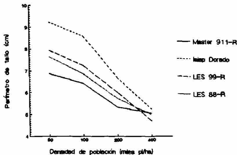
Figura 41. Perímetro de tallo de cuatro genotipos de sorgo a cuatro densidades de población M.V. 87
