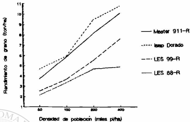
Figura 2. Rendimiento de grano en cuatro genotipos de sorgo a cuatro densidades de población M.V. 87.
