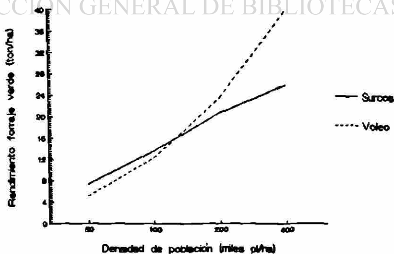
figura 69. Rendimiento de forraje verde por ha en dos métodos de siembra a cuatro densidades de población M.V. 87.
