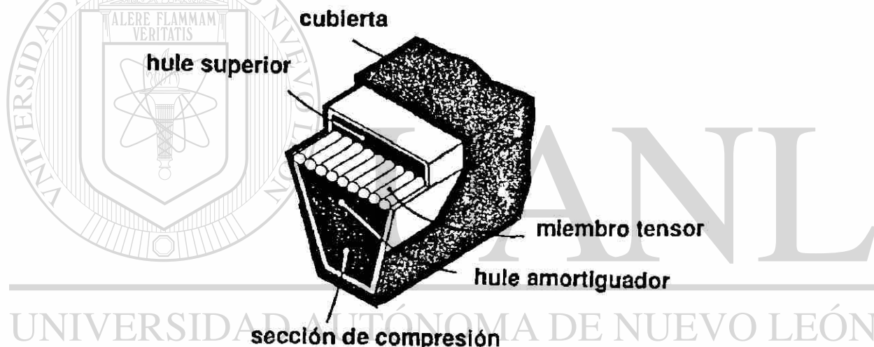
Fig. 4.14 Corte transversal que ilustra la construcción de una banda en V
