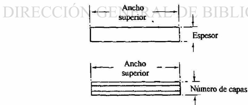
Fig. 4.10 Designación del tamaño de una banda plana.
