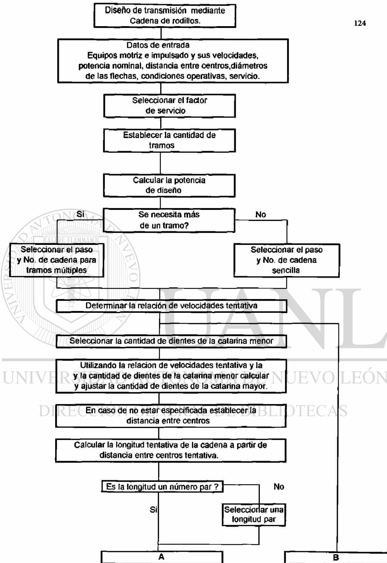
Fig. 5.7(a) Diagrama de flujo para la selección de cadenas de rodillos.
