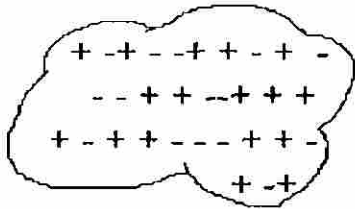
FIG 3.1.7.1 Nube de tormenta con distribución irregular de las cargas eléctricas.
