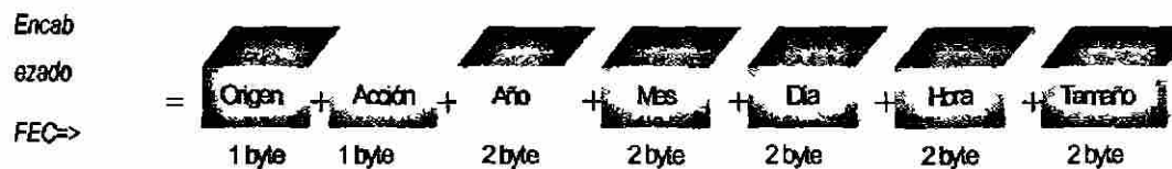
Figura 5. Encabezado de un mensaje FEC => Servidor
