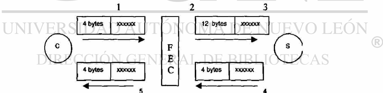
Figura 8. Secuencia de transmisión y recepción de Mensajes en el FEC
