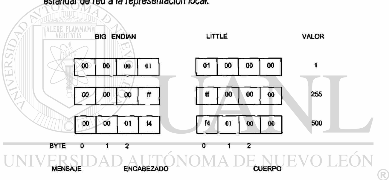
Figura 6. Diferentes Representaciones de Datos
