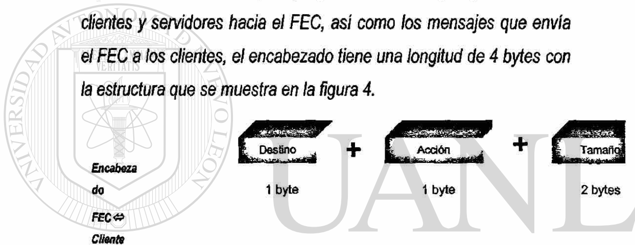
Figura 4. Encabezado de un mensaje FEC Cliente
