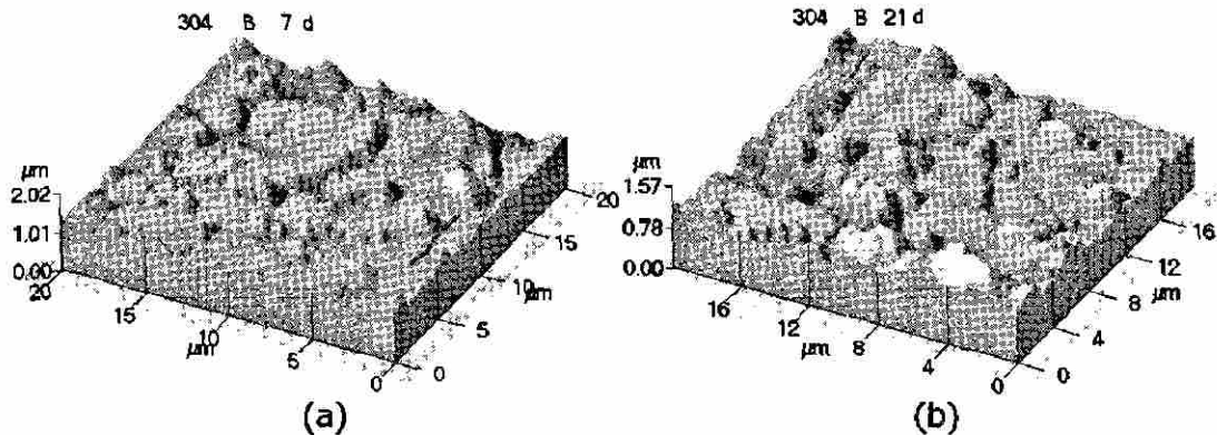
Figura 40. Imágenes AFM ( 20 \times 20 \mu\text{m}^2 ) de las películas pasivas formadas sobre el acero AISI 304 al ser expuesto en la solución de extracto de cemento en presencia de cloruro (10 g/l NaCl), durante 7 días (a) y 21 días (b).
