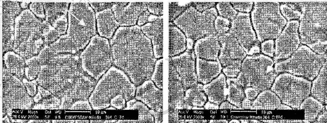
Figura 29. Imágenes SEM (X 2,000) de las películas pasivas del acero AISI 304 formadas naturalmente (a) y después de su exposición en la solución saturada de \text{Ca}(\text{OH})_2 a 7 días (b) y 21 días (c).
