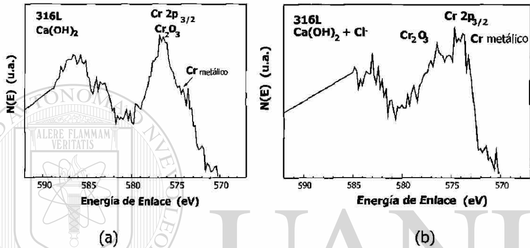
Figura 45. Espectros XPS del Cr de las películas pasivas del acero AISI 316L formadas (a) en la solución saturada de \text{Ca(OH)}_2 y (b) en la solución saturada de \text{Ca(OH)}_2 con cloruro (10 g/l NaCl) (6 días de exposición).
