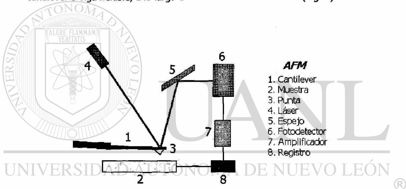
Figura 6. Esquema del microscopio AFM .
