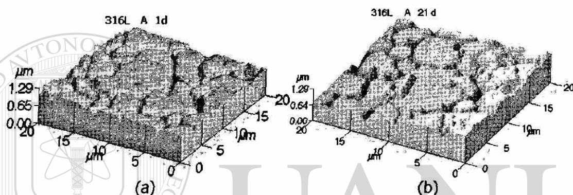
Figura 39. Imágenes AFM ( 20 \times 20 \mu\text{m}^2 ) de la topografía de la capa pasiva del acero AISI 316L expuesto en la solución de extracto de cemento durante 1 día (a) y 21 días (b).
