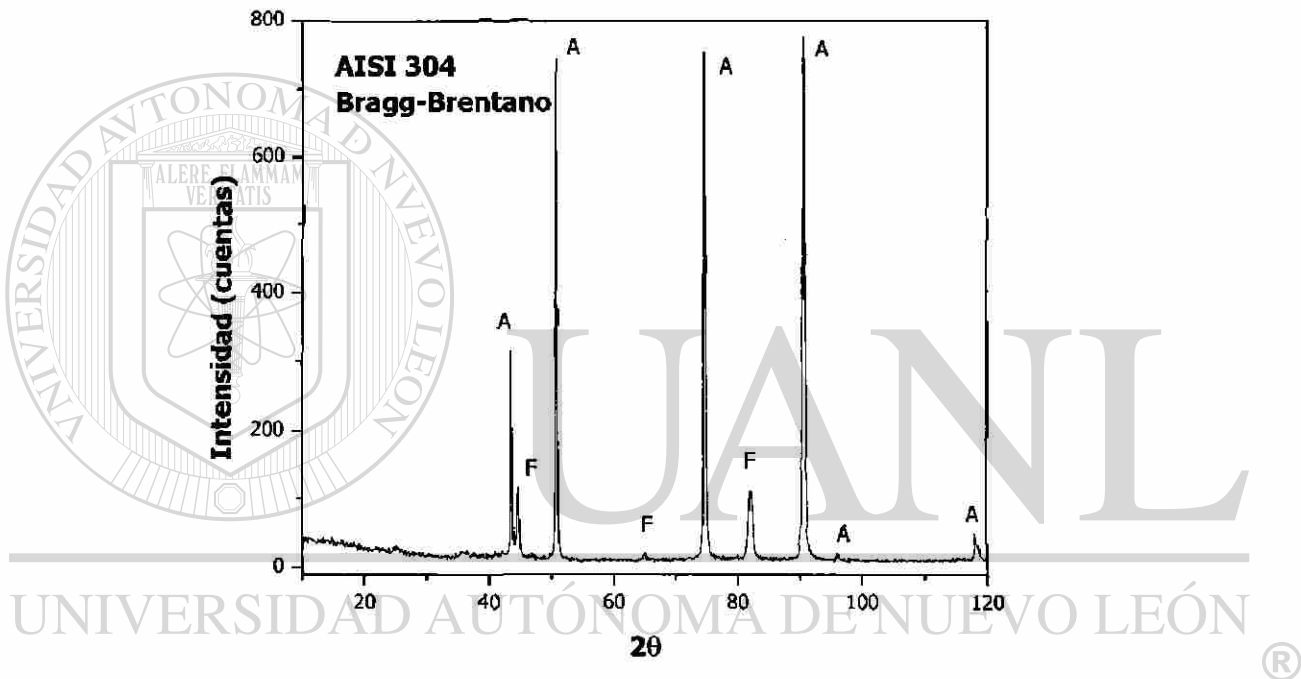
Figura 9. Difractograma del acero AISI 304 por geometría de Bragg-Brentano. La fase austenítica está marcada con A y la ferrítica con F.
