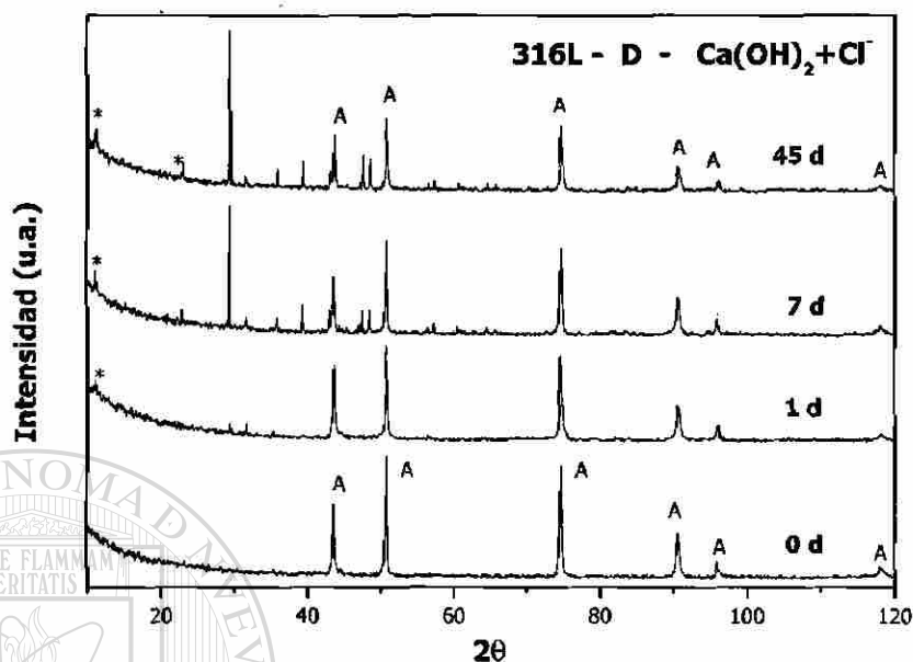
Figura 18. Difractograma del acero AISI 316L (técnica de haz rasante, 2^\circ ) expuesto en la solución saturada de \text{Ca(OH)}_2 con cloruro (10 g/l NaCl), a diferentes tiempos de inmersión. Las reflexiones de los productos de corrosión se indican con asteriscos.
