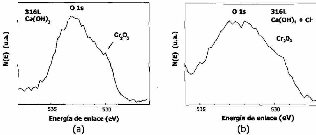
Figura 47. Espectros XPS del O de las películas pasivas del acero AISI 316L formadas (a) en la solución saturada de \text{Ca(OH)}_2 y (b) en la solución saturada de \text{Ca(OH)}_2 con cloruro (10 g/l NaCl) (6 días de exposición).
