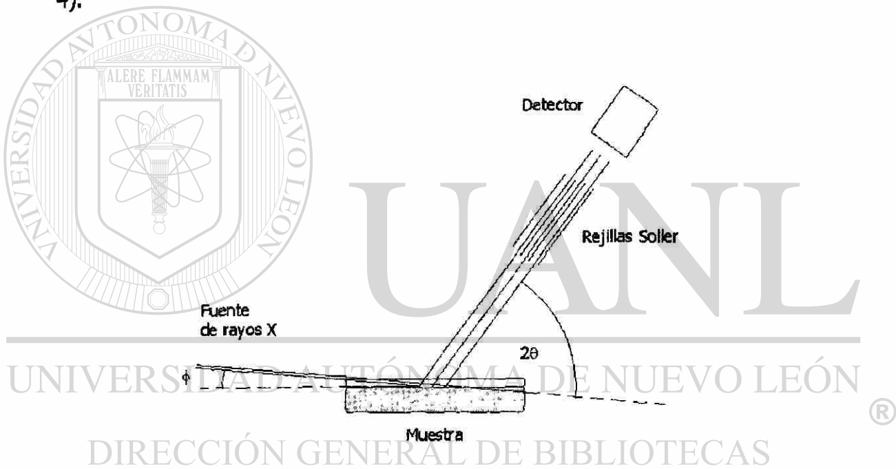
Figura 4. Geometría de haz rasante ( GID ) de la difracción de rayos X ( XRD ).
