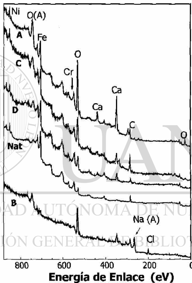
Figura 43. Identificación elemental por XPS de las capas pasivas formadas en el acero AISI 316L expuesto en las soluciones modelos: Nat-formada naturalmente, A-extracto de cemento, B-extracto de cemento con cloruro (10 g/l NaCl), C-solución saturada de \text{Ca}(\text{OH})_2 , y D-solución saturada de \text{Ca}(\text{OH})_2 con cloruro (10 g/l NaCl).
