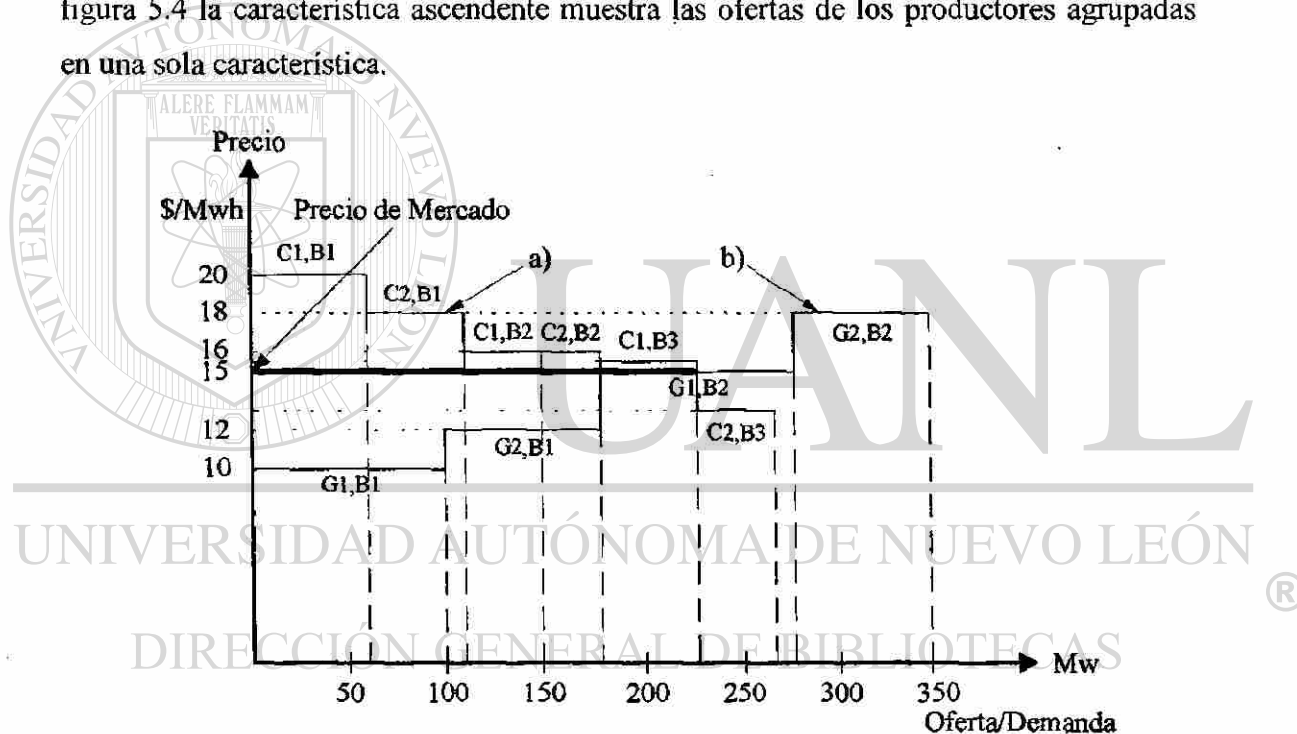
Fig. 5.4. Características del consumo y venta de energía en función del precio. a) Ofertas de compradores. b) Ofertas de productores.
