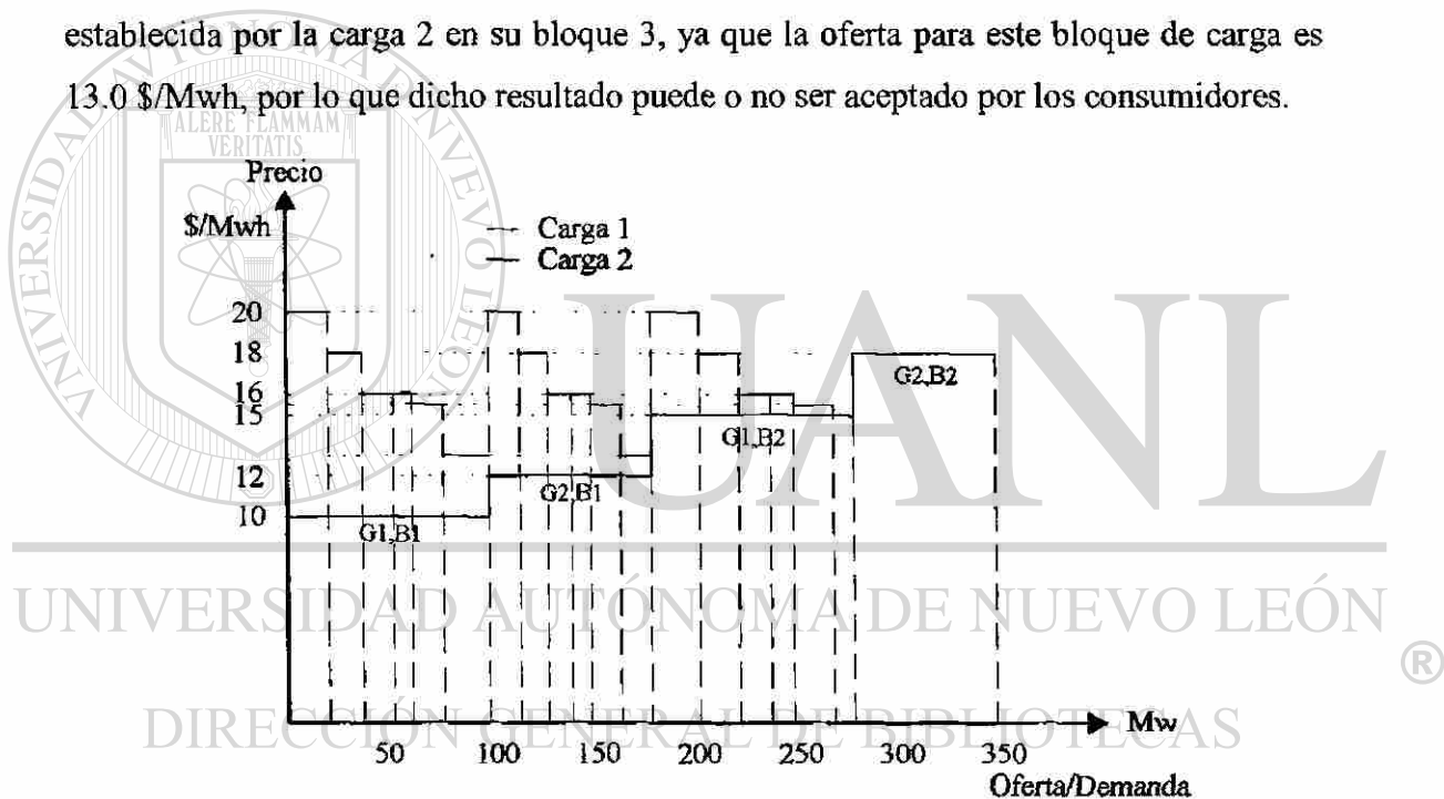
Fig. 5.5. Características del consumo y venta de energía maximizando el beneficio.
