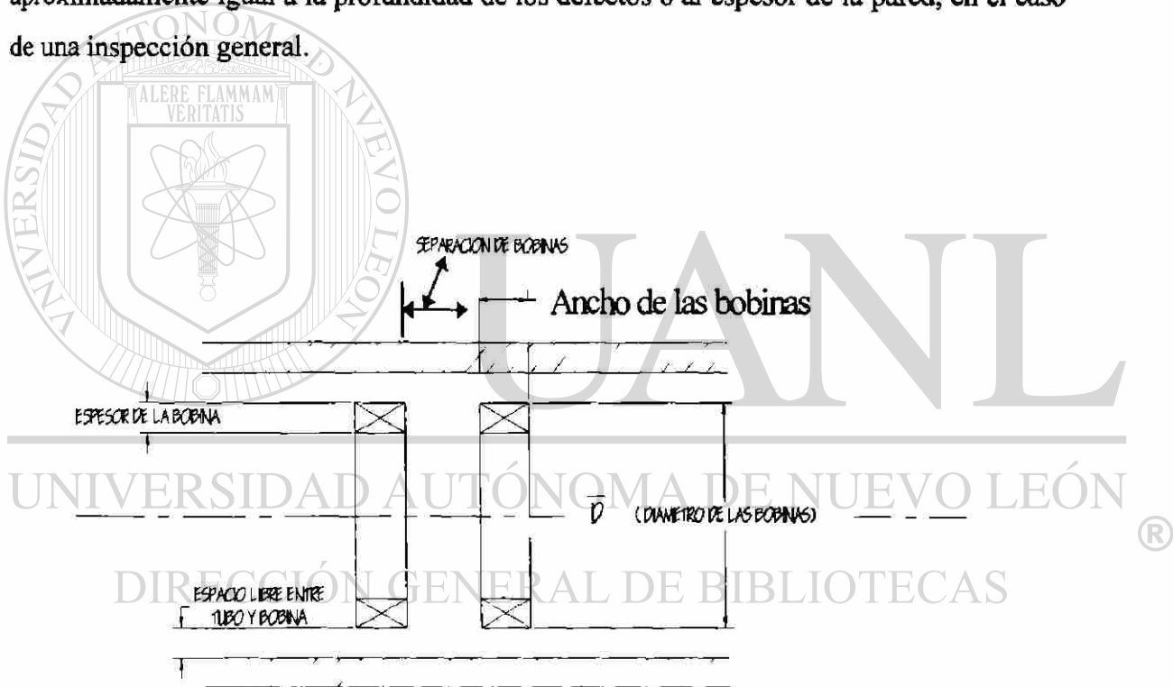
FIGURA 6.2 Nomenclatura de las bobinas de sonda
