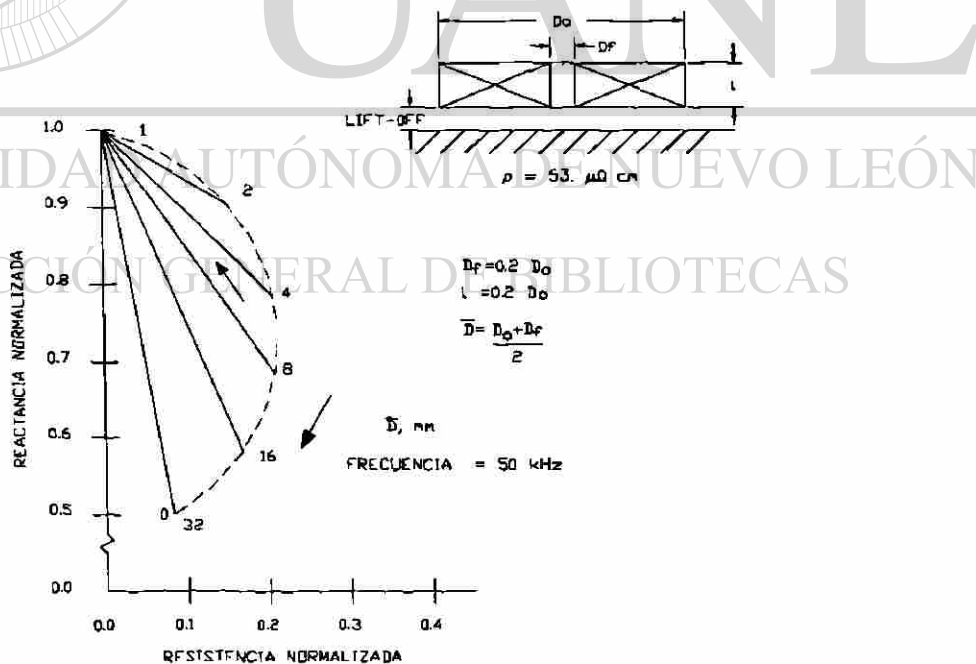
FIGURA 5.8 Gráfica de impedancia-efecto de diámetro de la bobina de superficie
