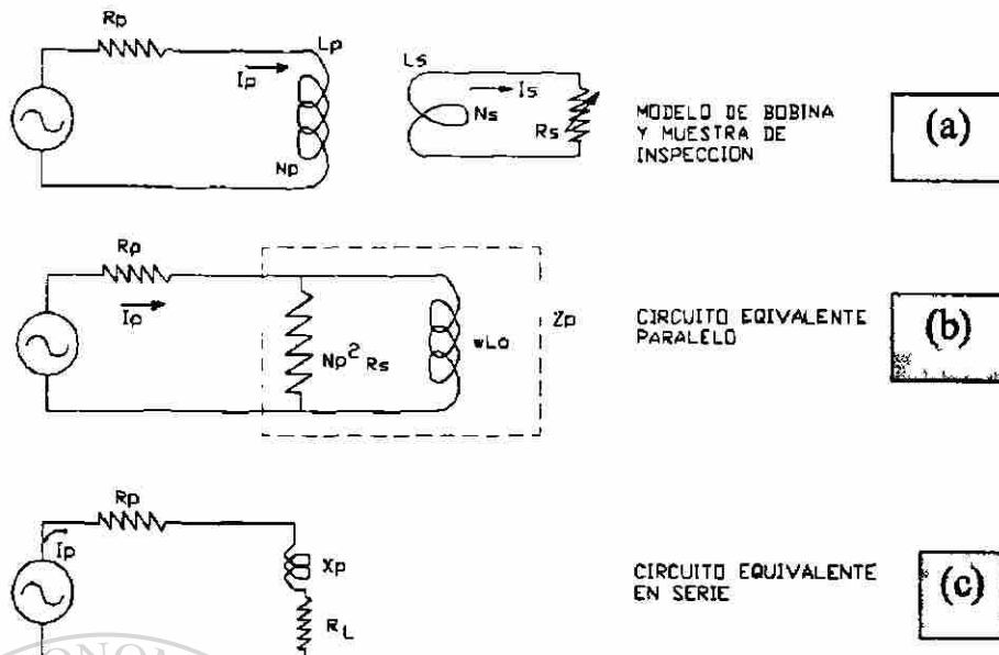
FIGURA 4.6 Circuitos equivalentes
