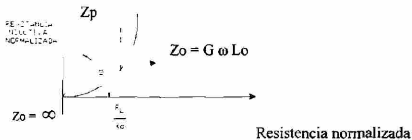
FIGURA 4.7 Representación gráfica de la impedancia
