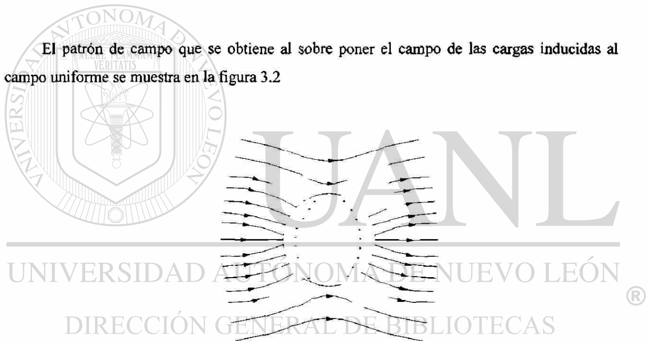
FIGURA 3.2 Patrón de campo de una esfera conductora en un campo eléctrico uniforme.
