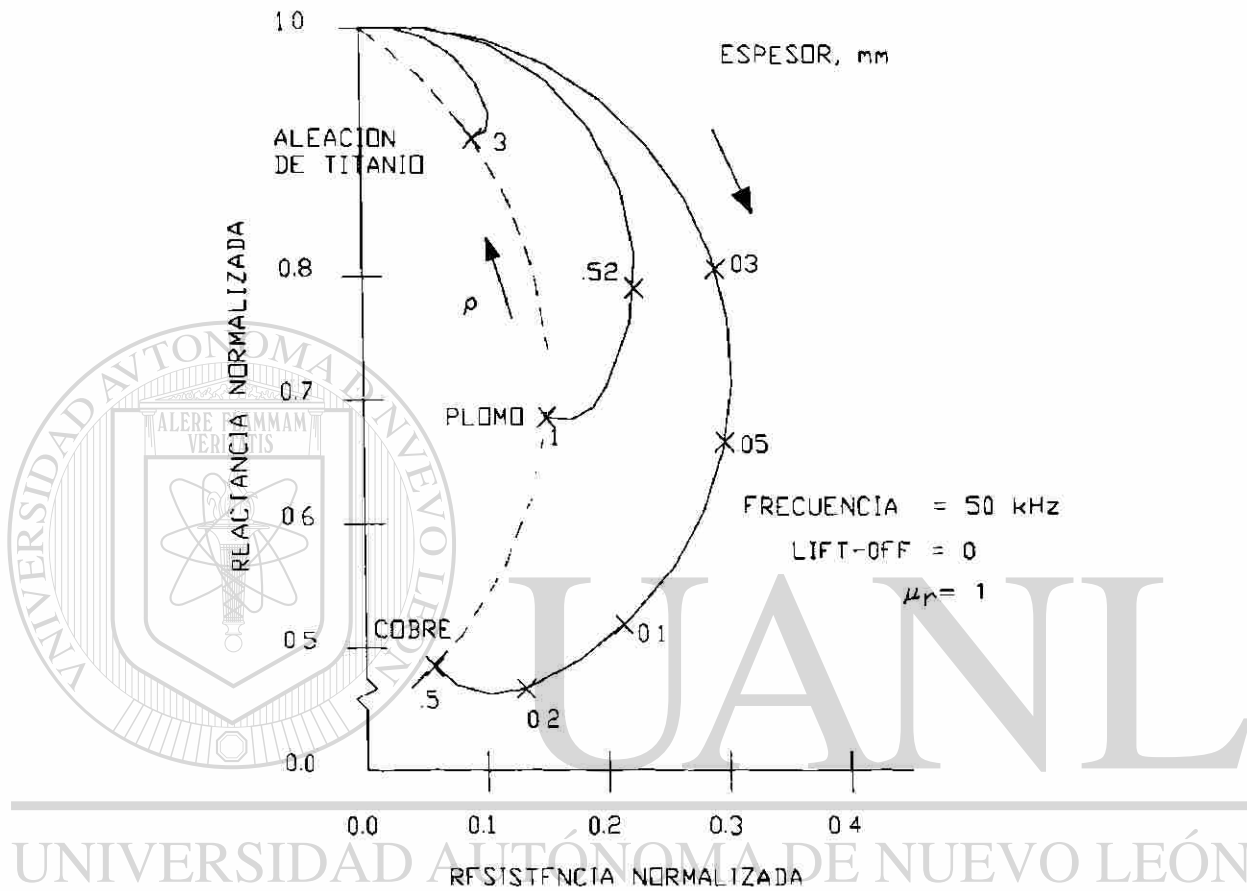
FIGURA 5.6 Gráfica de impedancia-efecto de espesor
