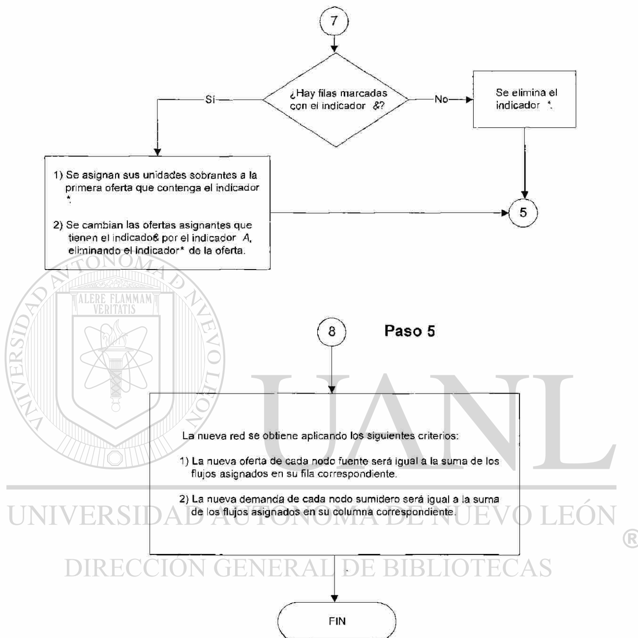
Figura 4.7. Diagrama del algoritmo heurístico De la Cruz entre los pasos 4 y 5.
