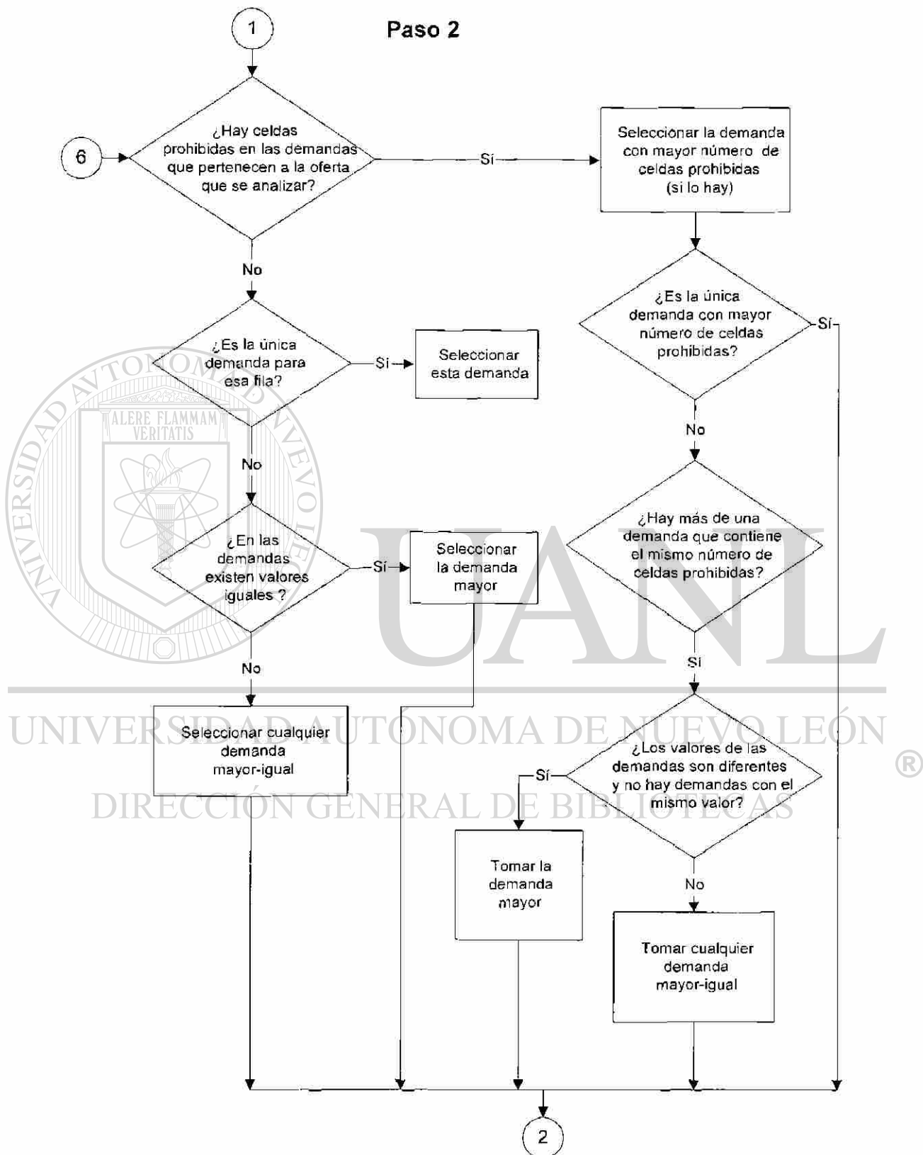
Figura 4.4. Diagrama del algoritmo heurístico De la Cruz en el paso 2.
