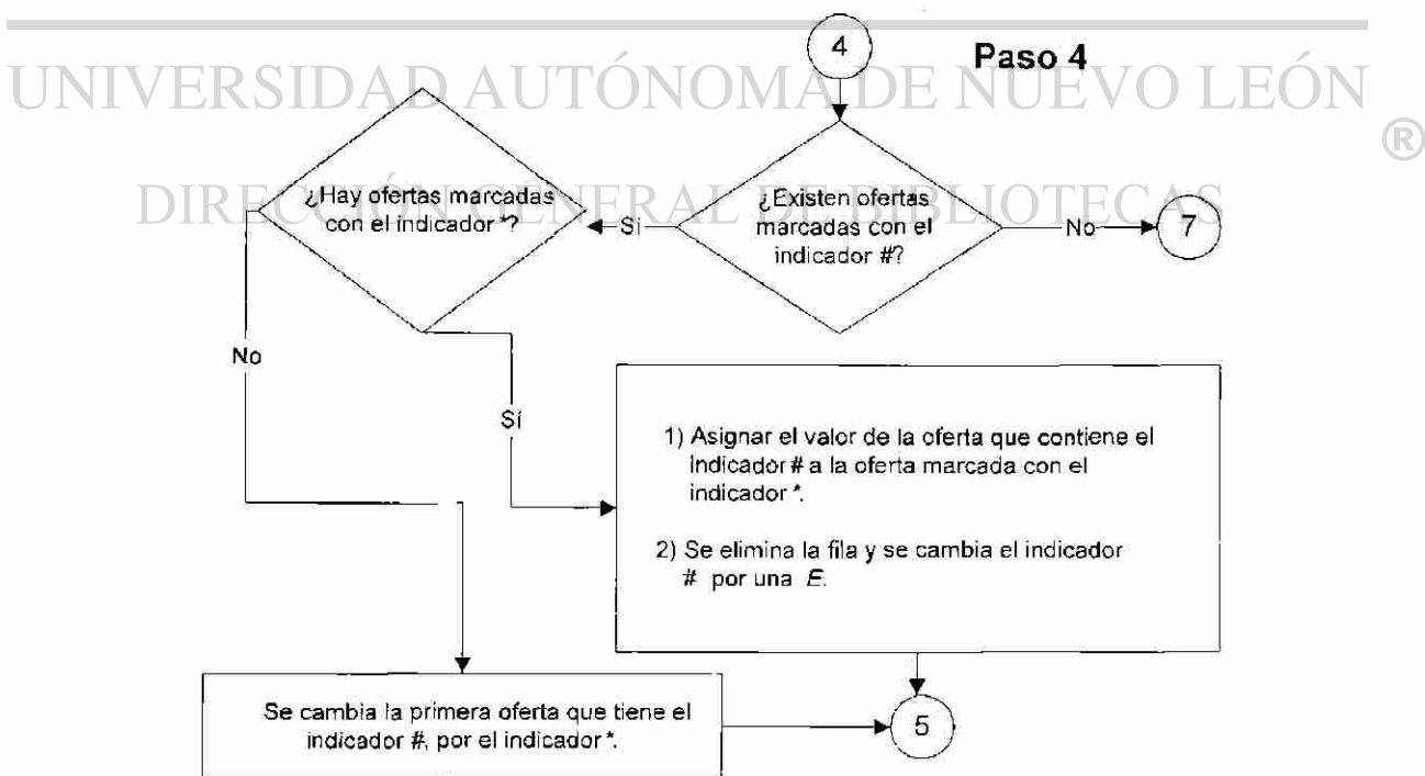
Figura 4.6. Diagrama del algoritmo heurístico De la Cruz entre los pasos 3 y 4.
