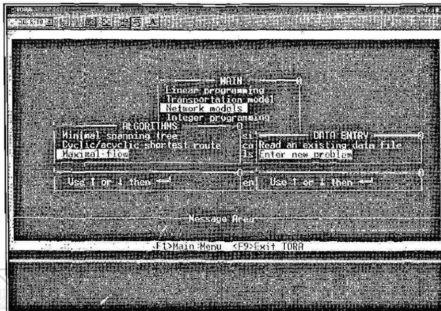
Figura 5.6. Submenú del algoritmo de "Flujo Máximo".
