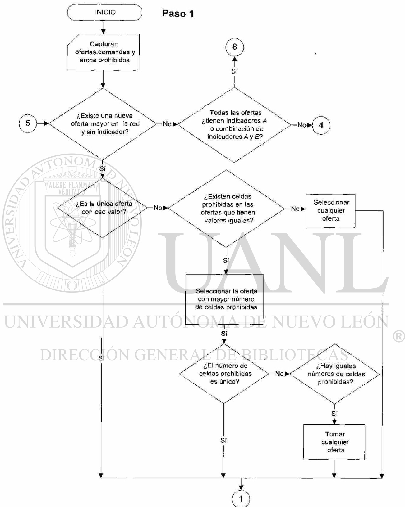
Figura 4.3. Diagrama del algoritmo heurístico De la Cruz en el paso 1.
