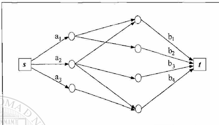
Figura 3.2. Red bipartita incompleta aumentada.
