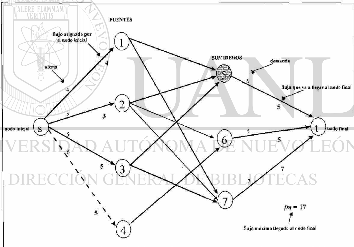
Figura 4.2. Aplicación del algoritmo de Flujo Máximo.
