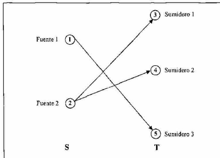
Figura 2.5. Red bipartita incompleta.
