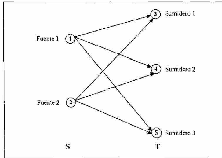
Figura 2.3. Red bipartita completa.
