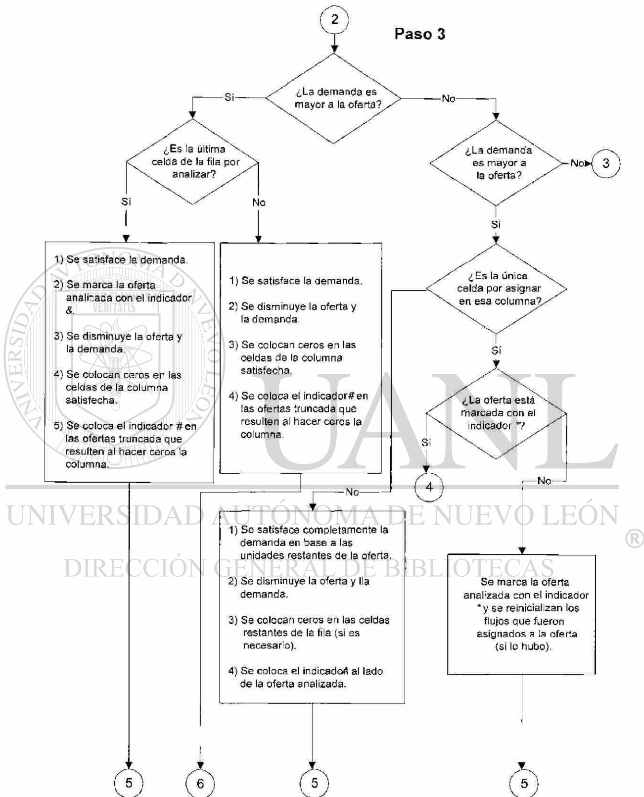
Figura 4.5. Diagrama del algoritmo heurístico De la Cruz en el paso 3.
