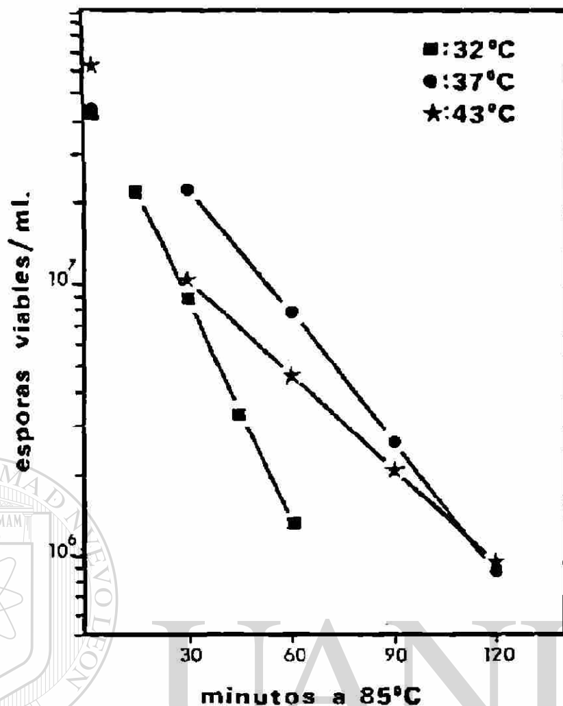
Fig. 25. Curvas de muerte térmica de esporas de C. perfringens cepa FD-1, producidas a 32, 37 y 43°C. y sometidas a 85°C.
