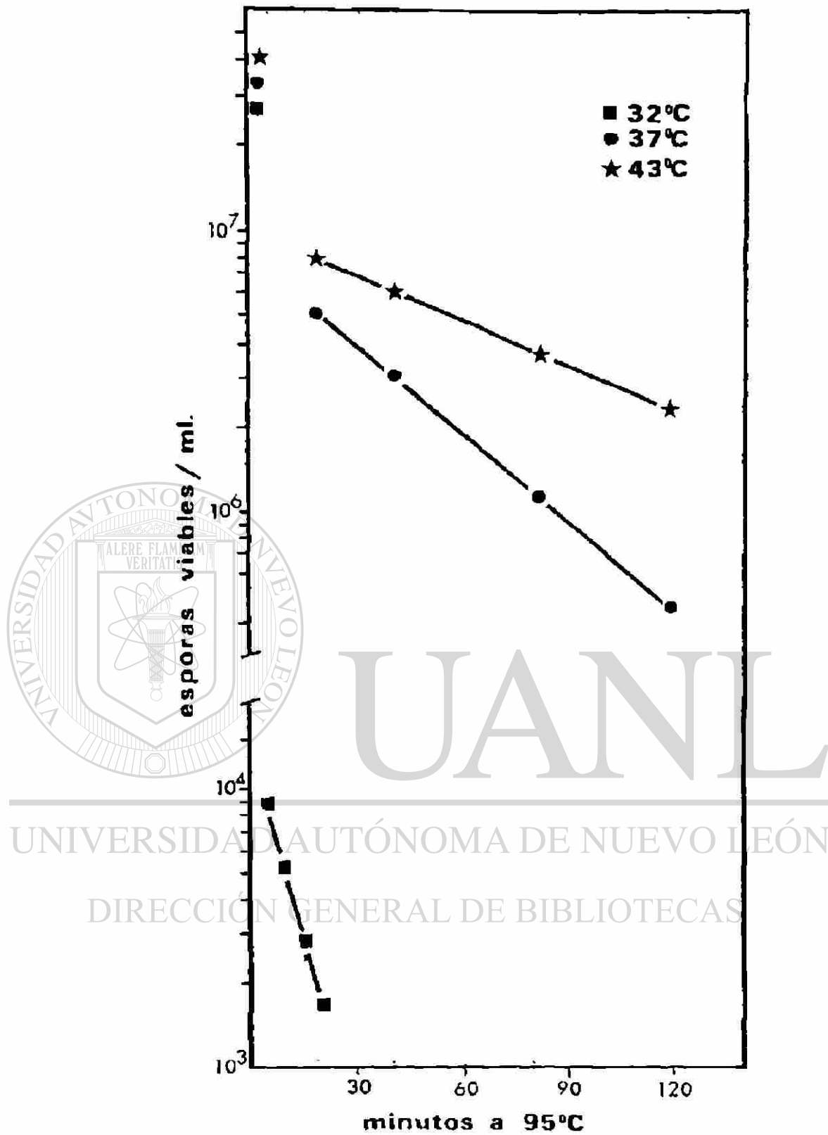
Fig. 24. Curvas de muerte térmica de esporas de C. perfringens cepa FD-1041, producidas a 32, 37 y 43°C, y sometidas a 95°C.
