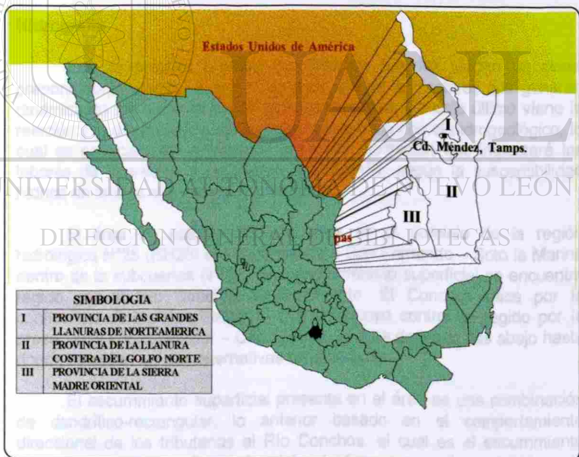
Figura N°4.- Provincias Fisiográficas de Tamaulipas (modificado de INEGI).
