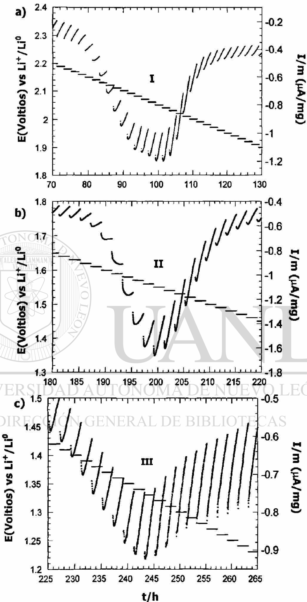
Figura 13. Curvas de relajación I vs t para la composición Nb_7W_{10}O_{47} . La velocidad de barrido utilizada fue de \pm 10 mV/2 h. a) Mximo I, b) Mximo II y c) Mximo III.
