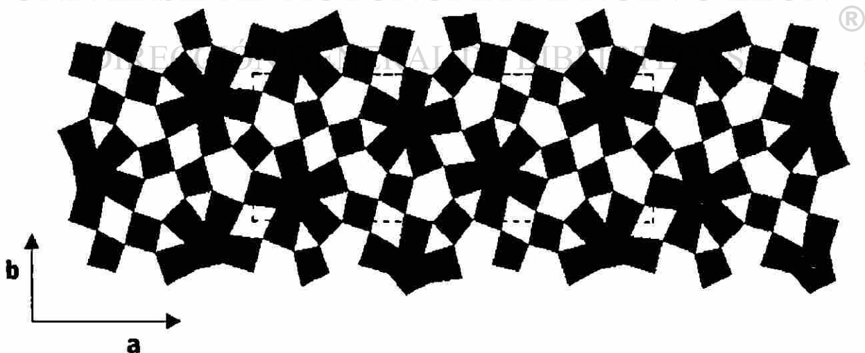
Figura 2. Enrejado Cristalino de Nb_8W_9O_{47}
