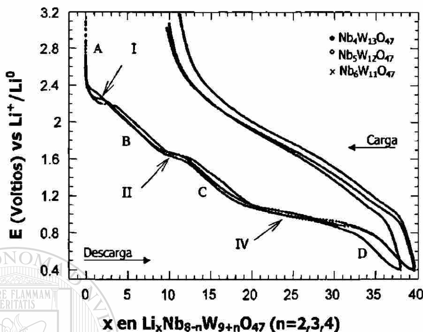
Figura 14.- Diagrama E vs x de las celdas con configuración \text{Li}/\text{Nb}_4\text{W}_{13}\text{O}_{47} , \text{Li}/\text{Nb}_5\text{W}_{12}\text{O}_{47} y \text{Li}/\text{Nb}_6\text{W}_{11}\text{O}_{47} , durante 1 ciclo completo carga-descarga. La intensidad de corriente aplicada fue de \pm 60 \mu\text{A} / 0.5 \text{ h} .
