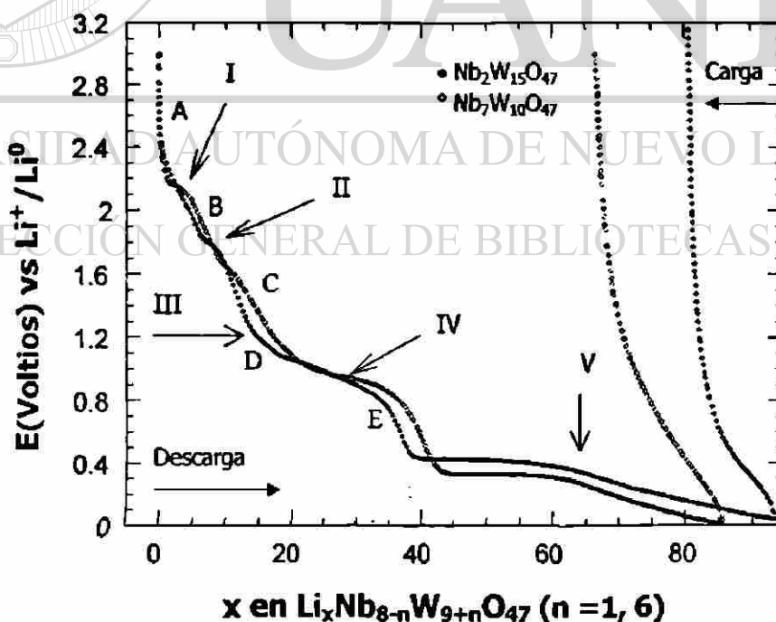
Figura 17. Diagrama E vs x para las celdas con configuración Li//Nb_2W_{15}O_{47} y Li//Nb_7W_{10}O_{47} en un intervalo de potencial de 3.0-0.01 Voltios vs Li^+/Li^0 . La intensidad de corriente aplicada fue de \pm 60 \mu A / 0.5 h .
