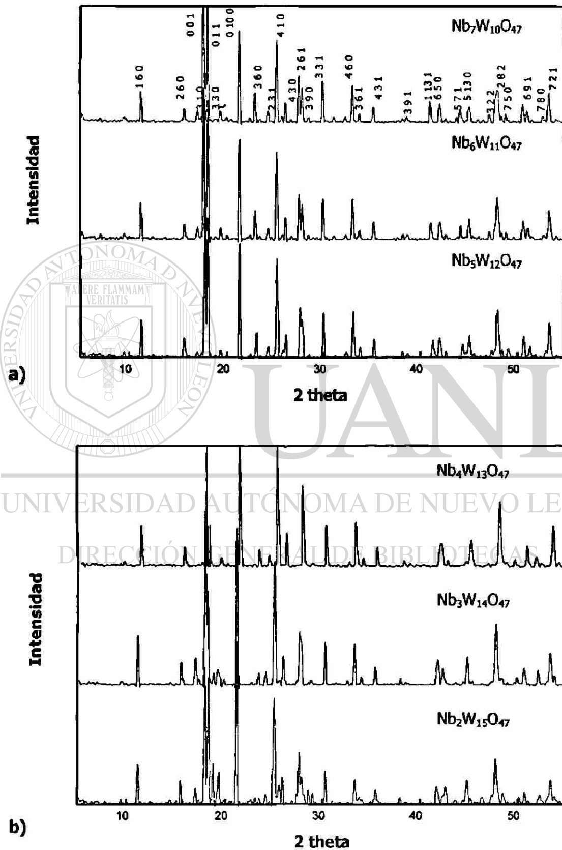
Figura 6.- Diagramas de difracción de rayos-X de las diferentes composiciones pertenecientes a la solución sólida Nb_{8-n}W_{9+n}O_{47} ( 1 \leq n \leq 6 ).
