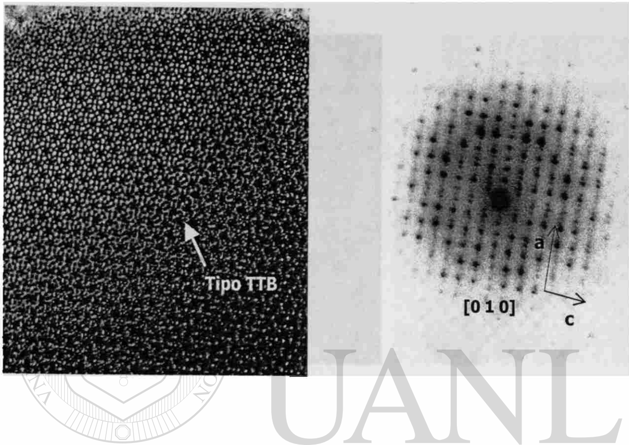
Figura 7.- Diagrama de difracción de electrones e imagen de la composición \text{Nb}_2\text{W}_{15}\text{O}_{47} en el eje de zona [0\ 1\ 0] .
