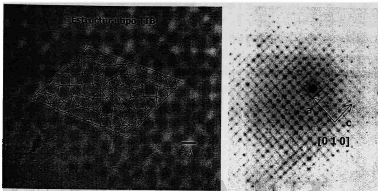
Figura 8.- Diagrama de difracción de electrones e imagen de la composición Nb_4W_{13}O_{47} en el eje de zona [0\ 1\ 0] .
