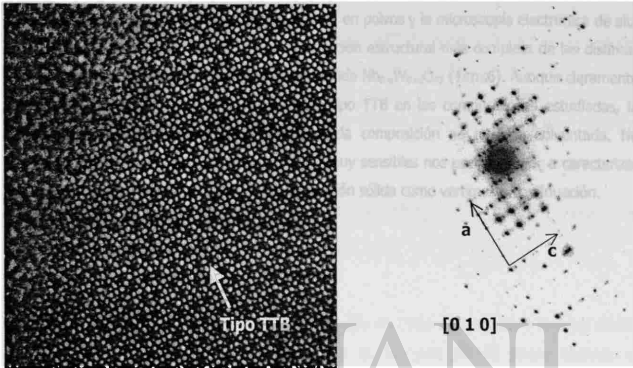
Figura 9.- Diagrama de difracción de electrones e imagen a lo largo del eje [0\ 1\ 0] , para la composición Nb_7W_{10}O_{47} .
