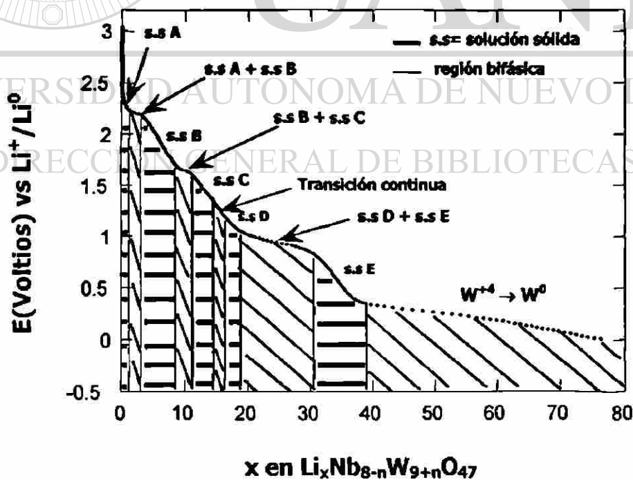
Figura 24. Diagrama de fases para el sistema \text{Li}/\text{Nb}_{8-n}\text{W}_{9+n}\text{O}_{47}(1 \leq n \leq 6) .
