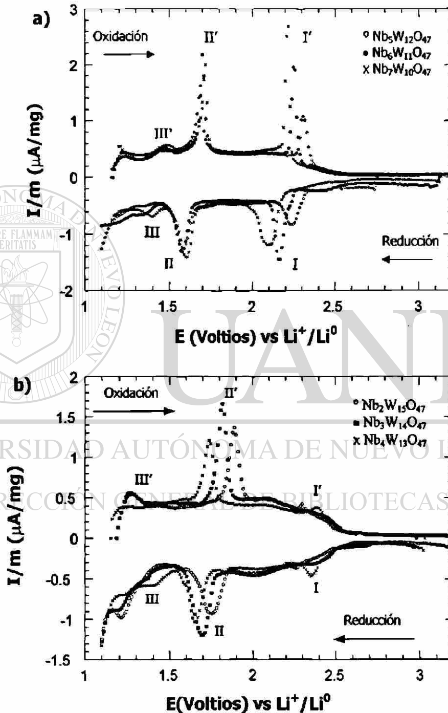
Figura 11.- Diagrama I vs E de un conjunto de celdas con configuración \text{Li}/\text{Nb}_{8-n}\text{W}_{9+n}\text{O}_{47} ( 1 \leq n \leq 6 ) que muestran 1 ciclo completo de carga-descarga. La velocidad de barrido utilizada fue de \pm 10 \text{ mV}/2 \text{ h} .
