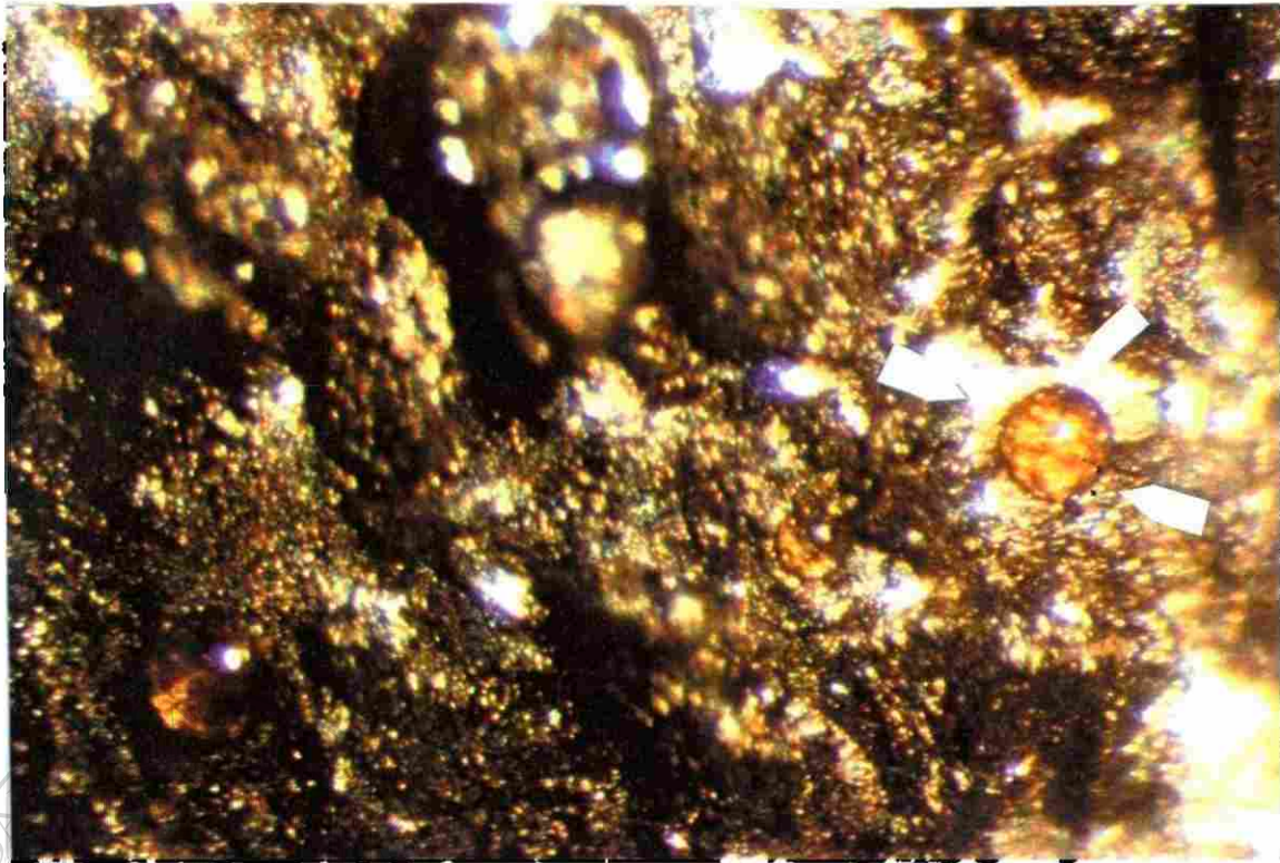
Fig. 5.4.1 Fotografía donde se muestra una gota de \text{SiO}_2 , la cual posteriormente se unirá a la wustita para formar la fayalita.
