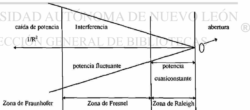
Fig 4.3.1 Zonas de radiación de una abertura [21]
