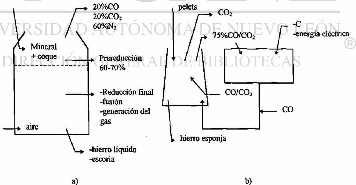
Fig. 2.6.1 Presentación esquemática de los procesos de reducción de mineral de hierro, a) alto horno, b) Wüster.
