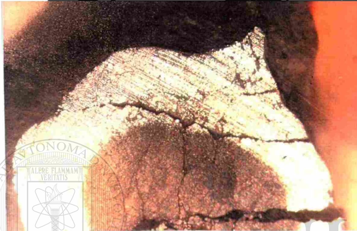
fig. 5.2.2 Fotografía donde se muestra la reducción topoquímica en un pelet de mineral de hierro a una temperatura de 950^{\circ}\text{C} en 55\%\text{H}_2 21\%\text{CO} 14\%\text{CO}_2 y 10\%\text{N}_2 , donde la fase amarilla es hierro metálico y la fase gris es wustita.
