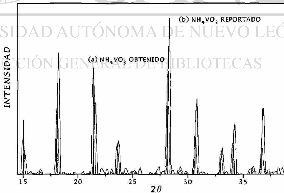
Difractograma 3.13 Comparación del metavanadato obtenido por la filtración en caliente vs el metavanadato comercial de la marca ALFA
