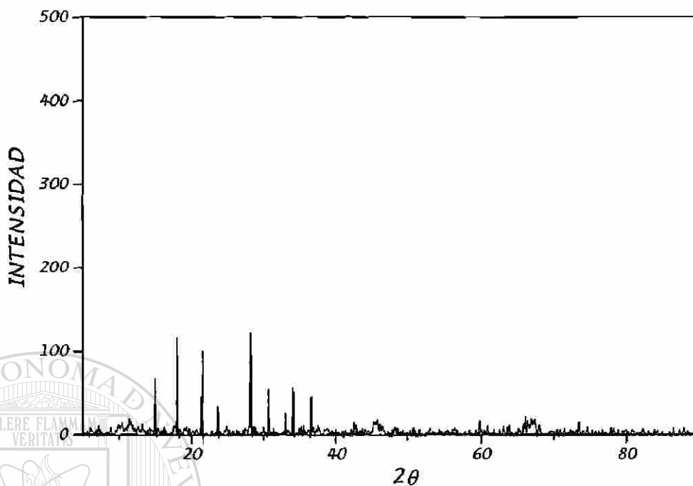
Difractograma 3.12 Metavanadato obtenido de la filtración en frío
