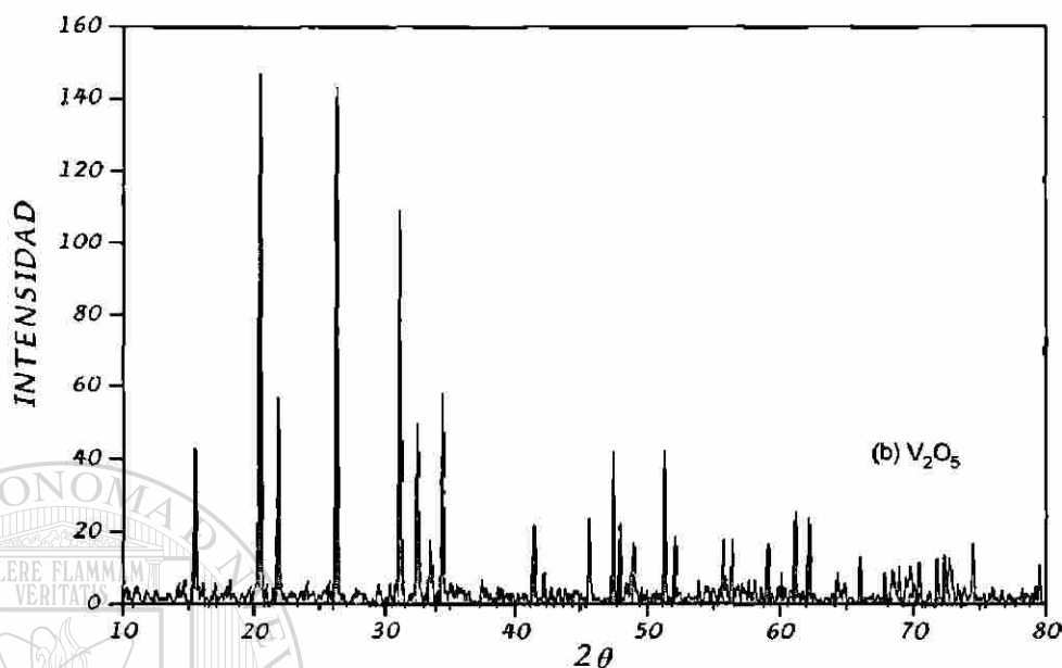
Difractograma 3.14b Pentóxido de vanadio obtenido de la descomposición del NH_4VO_3 (ec. 13) de la filtración en frío
