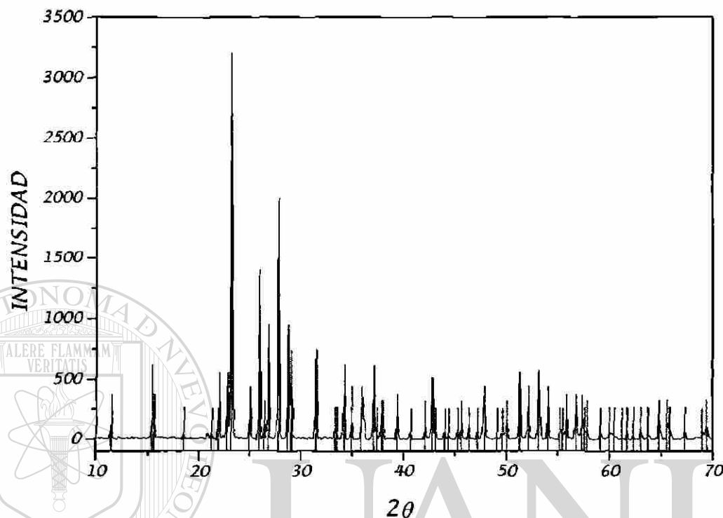
Diffractograma 3.3 Señales de Azufre en el residuo del catalizador después de ser tratado con bisulfuro de carbono
