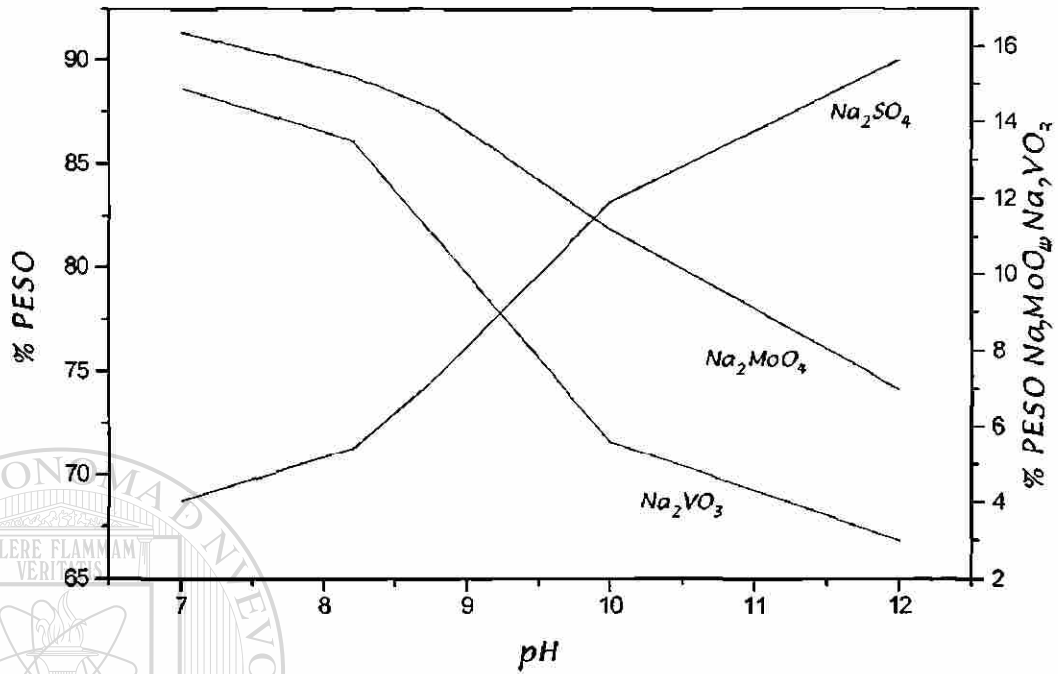
Figura 3.4 Variación del porcentaje en peso de los compuestos con respecto al pH de la solución alcalina
