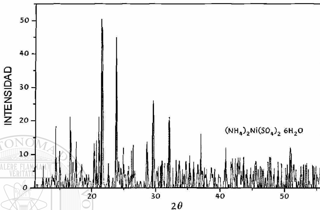
Difractograma 3.5 Señales de el compuesto nickelboussingaultite y su patrón reportado
