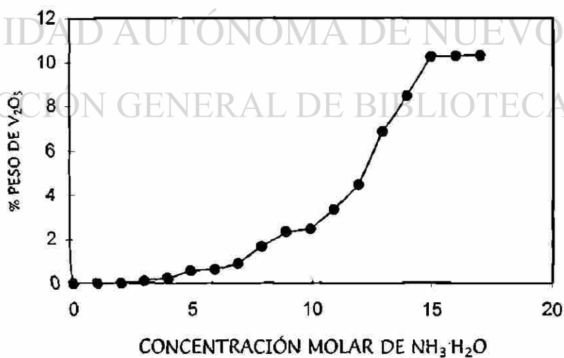
Figura 3.6 Porcentaje en peso de V_2O_5 vs Concentración molar de NH_3 \cdot H_2O
