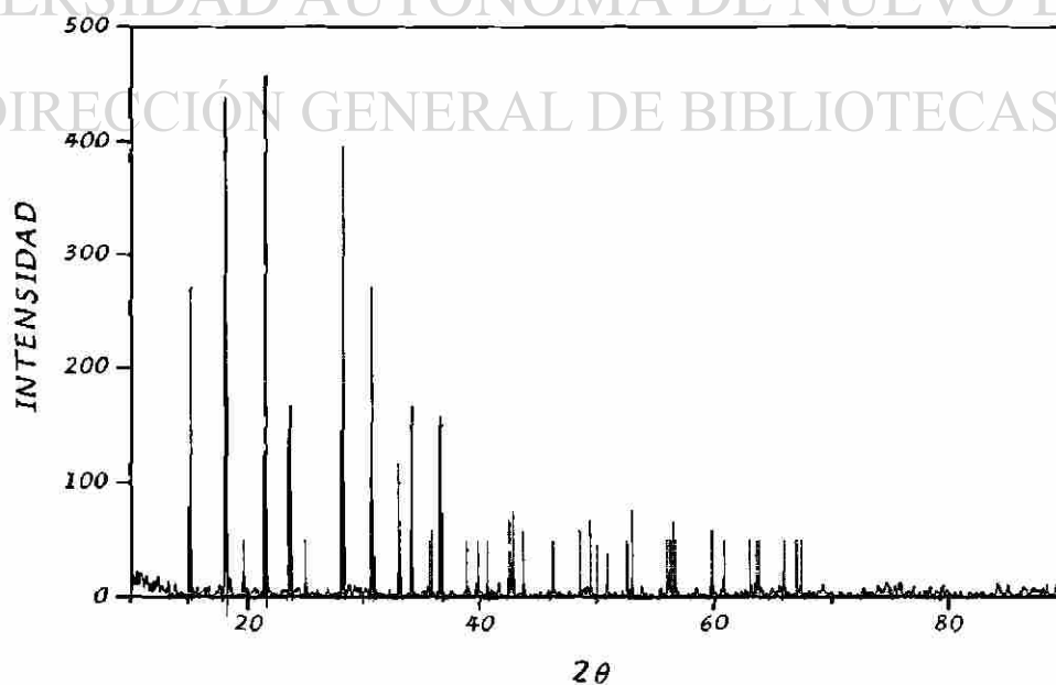
Diffractograma 3.11 Metavanadato obtenido de la filtración en caliente
