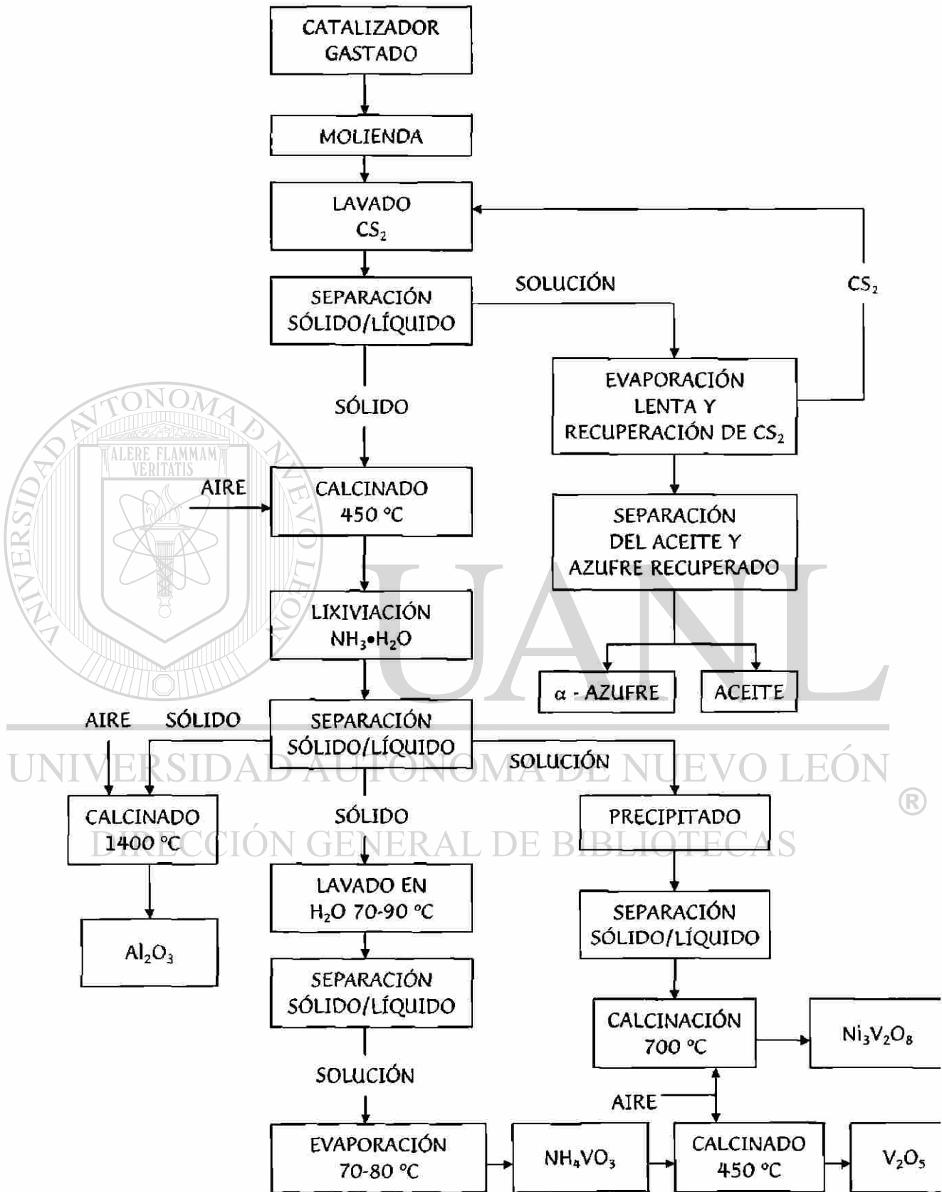
Figura 2.5 Diagrama de flujo para la lixiviación con \text{NH}_3 \cdot \text{H}_2\text{O}
