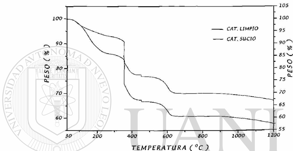
Figura 3.3 Pérdida de peso por la técnica de TGA
