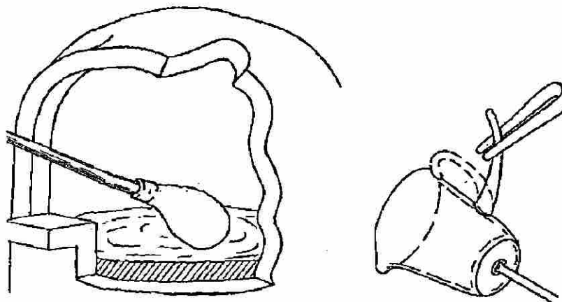
Fig. 2.5 Esquema de la fabricación de vidrio soplado
