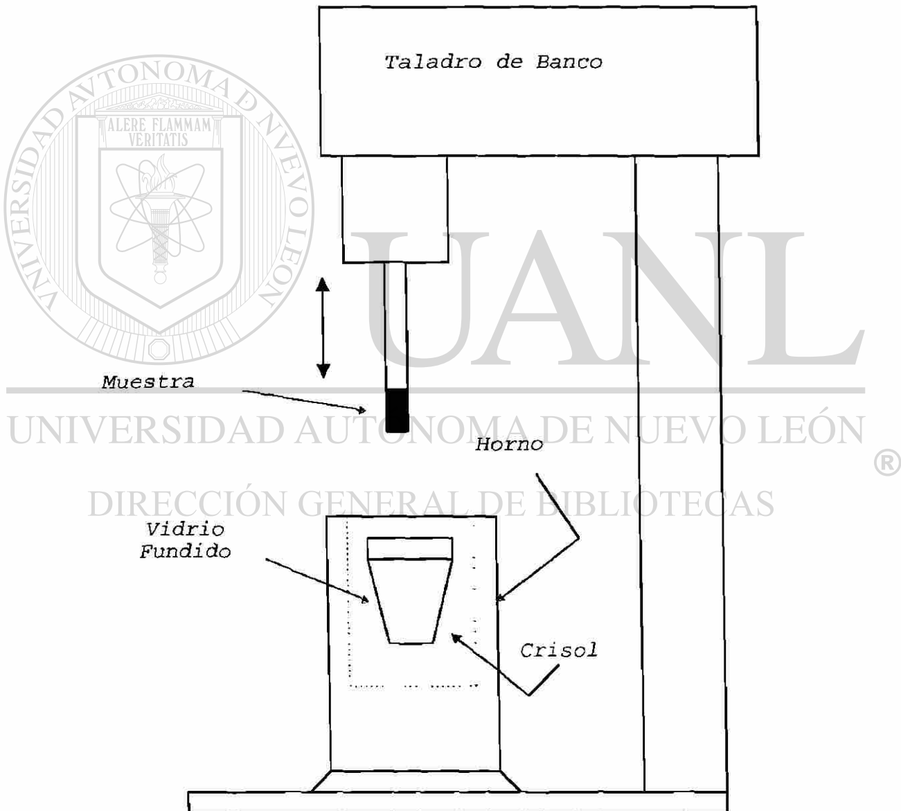
Fig. 5.1 Representación Esquemática del sistema de pruebas de desgaste para material cerámico
