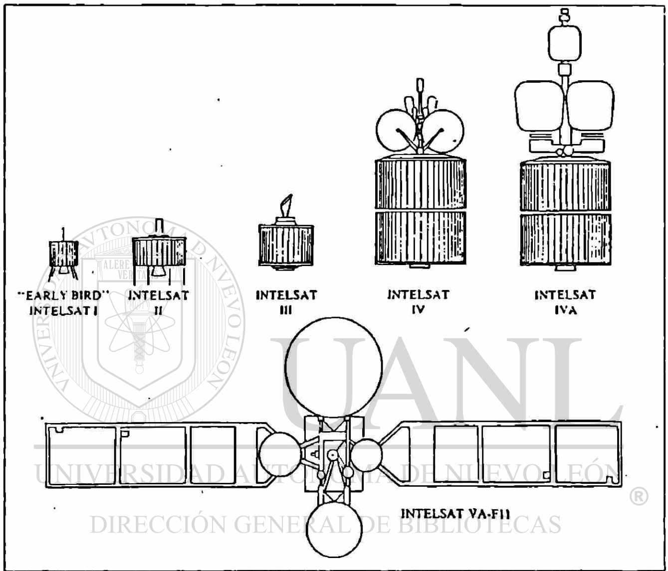
Representación a escala de las series INTELSAT
