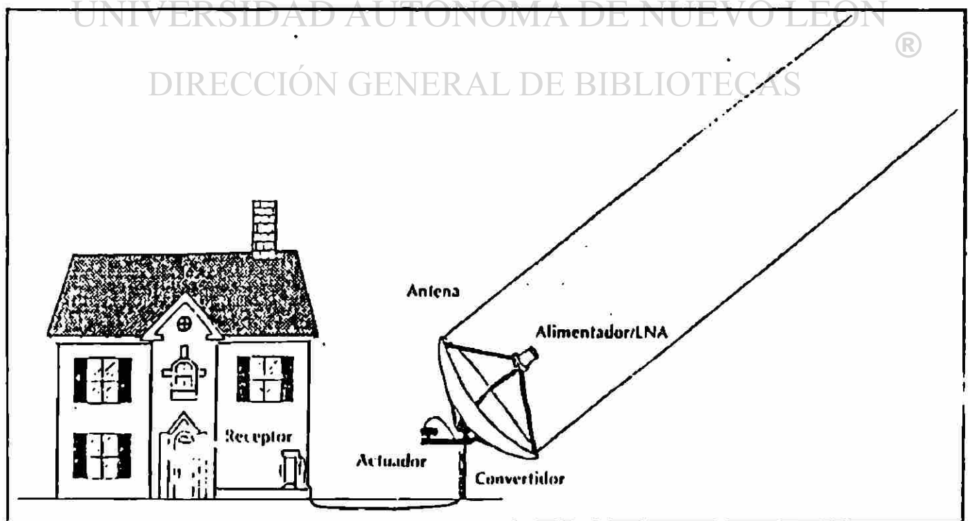
Estación Terrestre Típica. Las señales captadas por la antena son enfocadas hacia el alimentador y el amplificador de ondas bajas. Luego son transmitidas por cable hacia el convertidor, y de ahí a un receptor de satélite modificador. El sistema puede alimentar cualquier número de equipos de televisión.
