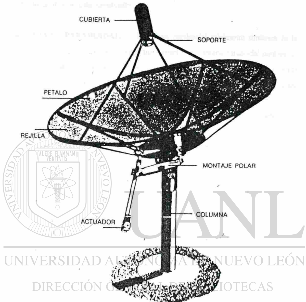
Esquema antena con paraboloides por sectores de rejilla adecuada para satélites de 4 GHz
