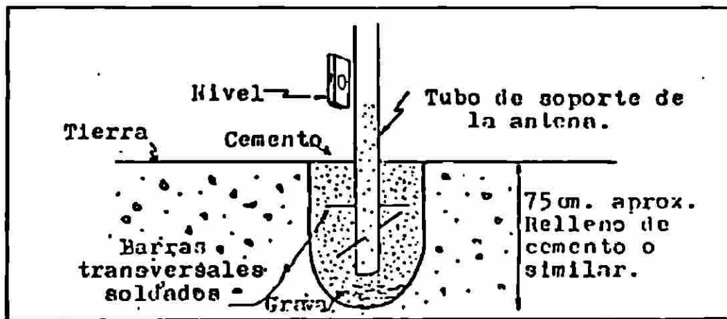
TIPOICO SOPORTE DE POSTE DE ANTENA
