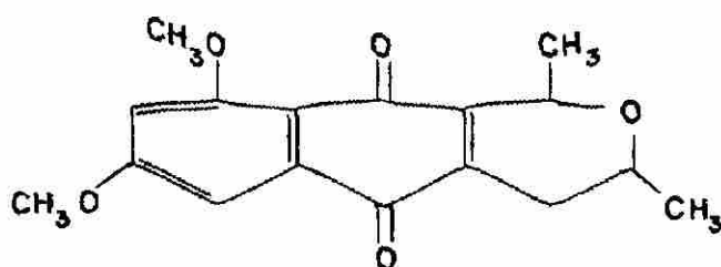
7-METOXIELEUTERINA
