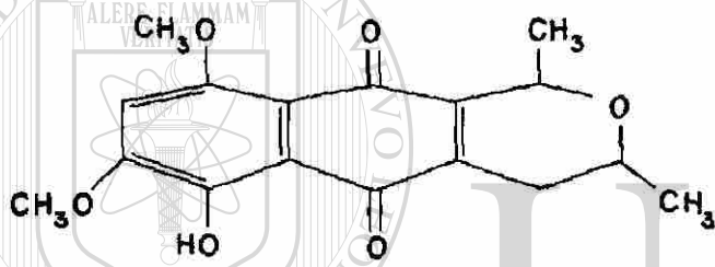
6-OH-7-METOXIELEUTERINA
