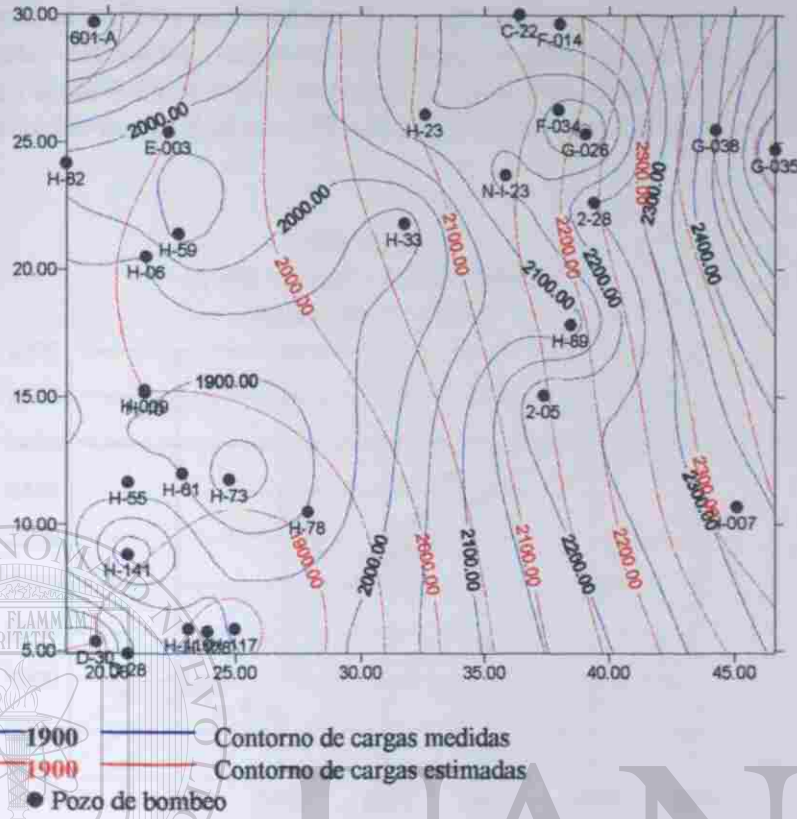
Figura 4.14. Representación de contornos medidos y estimados de cargas piezométricas para 1996.
