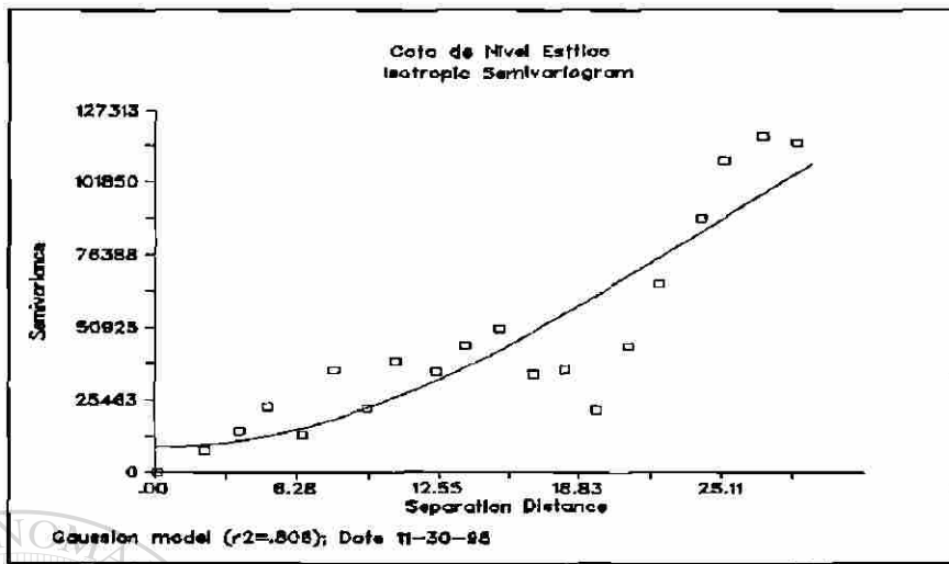
Figura 4.9. Modelo isotrópico gaussiano para la cota de nivel estático.
