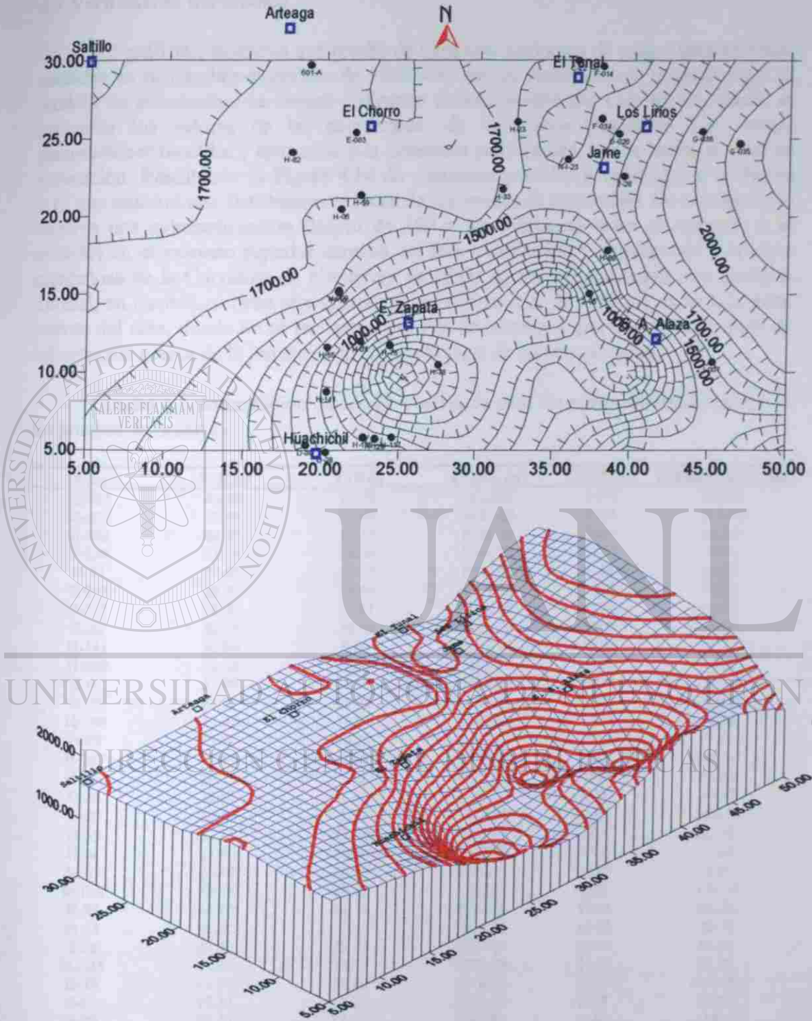
Figura 4.13. Carta y Perfil Piezométrico en bloque simulado para el año 2020 del área de estudio.
