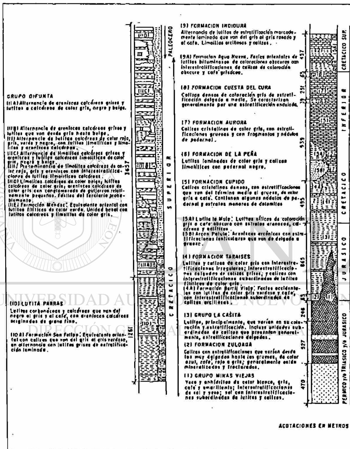
Figura 3.3. Secuencia estratigráfica de la Provincia Plegada de Coahuila (Adaptada de Wall et al. 1961).
