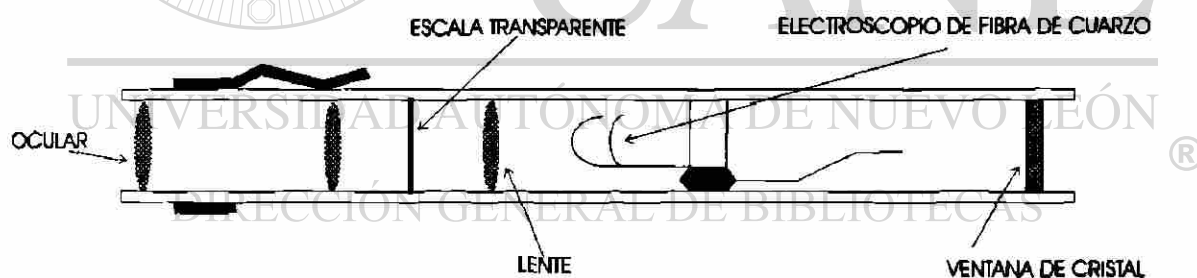
DOSIMETRO TÍPICO DE BOLSILLO DE LECTURA DIRECTA
