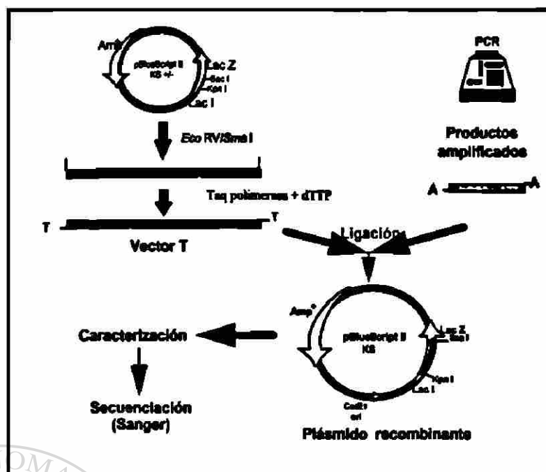
Fig. 8. Estrategia de clonación. Los productos de PCR obtenidos fueron ligados al vector pBS-KS II, formando así lo que es el plásmido recombinante el cual posteriormente fue transformado en células Ca^{++} competentes; luego las clonas recombinantes obtenidas fueron caracterizadas utilizando diferentes enzimas de restricción; finalmente las clonas recombinantes que tuvieran el inserto deseado fueron secuenciadas.
