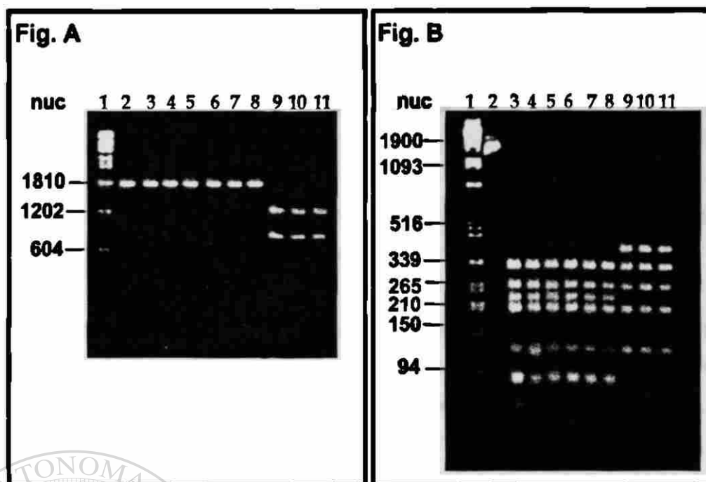
Fig. 14. Diferenciación del inserto de las clonas recombinantes. Se muestran las clonas que fueron amplificadas y caracterizadas por digestión con las enzimas Eco RI (Fig. A) y Alu I (Fig. B). Los productos generados fueron resueltos en geles de agarosa al 1.0% y 2.5%, respectivamente. Carril 2 producto sin digerir; carriles 3 al 11, digestión de las clonas; carril 1 marcador \lambda cortado con Pst I para la fig A y para la fig B un cósmido recombinado cortado con Bam HI y Eco RI.
