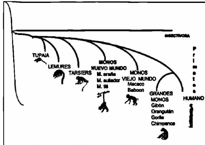
Fig 3. Evolución paleontológica de los primates. Se muestra la evolución de los primates según los datos paleontológicos. A partir de un orden ancestral cercano a los tarsiers, divergieron los monos del nuevo mundo, los monos del viejo mundo y finalmente los grandes monos y el humano (Alvarez, 1977).
