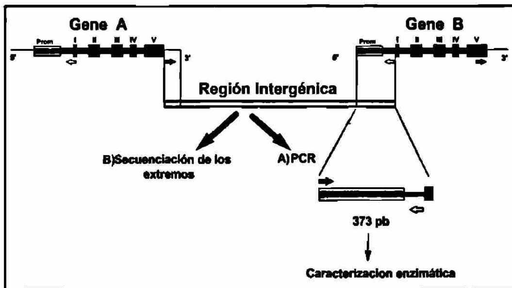
Fig.11. Estrategia para obtener la organización del locus. Se muestra el traslape de la región intergénica con los genes para así lograr la organización del locus del complejo multigénico GH-PL del mono araña.
