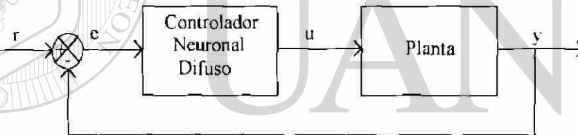
Fig. 4.1.- Diagrama de bloques de un Sistema de Control Neuronal Difuso
