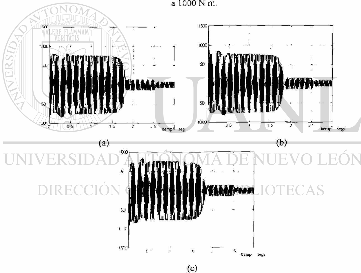
Fig. 5.42.- Corrientes en las fases a, b y c del motor con un cambio del par mecánico a 1000 N m
