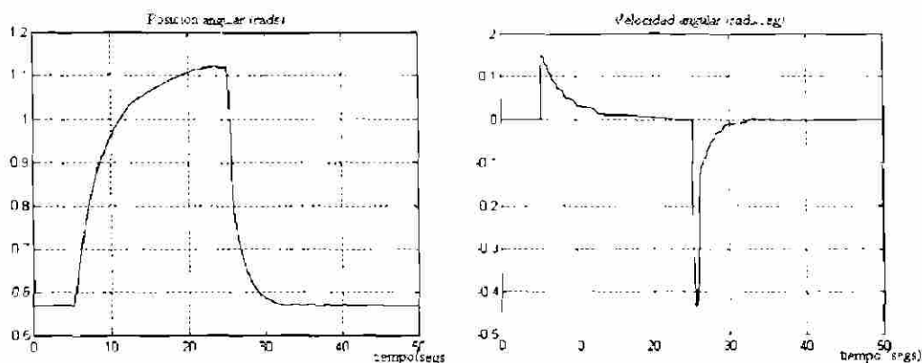
Fig. 5.8.- Falla tipo a (0.6) sin integrador y sin ruido
