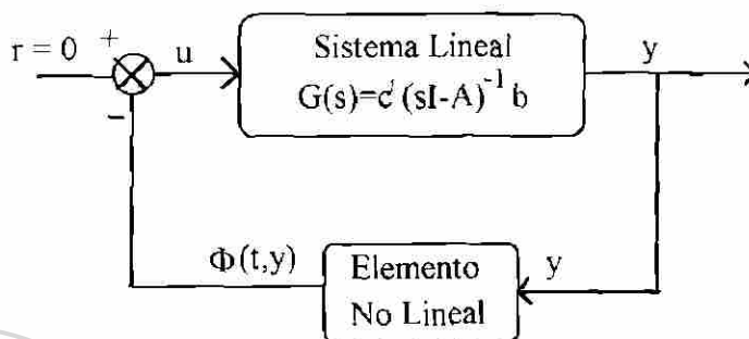
Fig. 4.5.- Sistema retroalimentado
