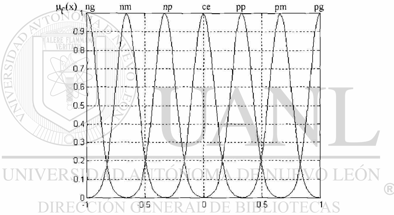
Fig 2.5.- Definición funcional con funciones tipo gaussianas
