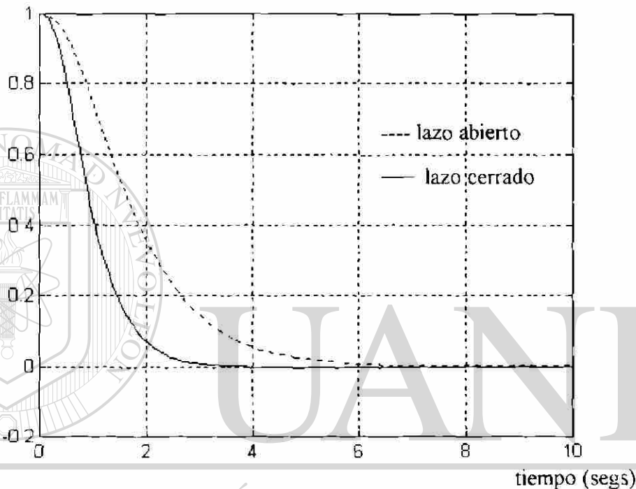
Fig.4.7.- Sistema de Tercer Orden en lazo abierto y lazo cerrado
