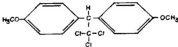
2,2-bis-(P-METOXIFENIL)-1,1,1-TRICLOROETANO.
