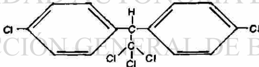
2,2-bis-(P-clorofenil)-1,1,1-tricloroetano
