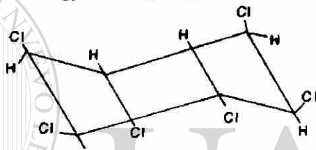
1 \alpha ,2 \beta ,3 \beta ,4 \alpha ,5 \beta ,6 \beta -HEXACLORO-CICLOHEXANO
