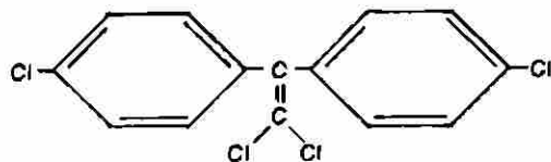
2,2-bis-(P-CLOROFENIL)-1,1-DICLORO-ETILENO.
