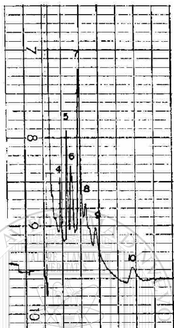
CROMATOGRAMA DE LA SOLUCION ESTANDAR B.
