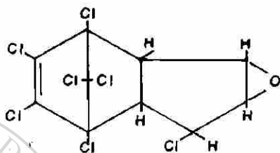
1,4,5,6,7,8,8-HEPTACLORO-2,3-EPOXI-2,3,3 \alpha ,4,7,7 \alpha -HEXAHIDRO-4,7-METANOINDENO.
