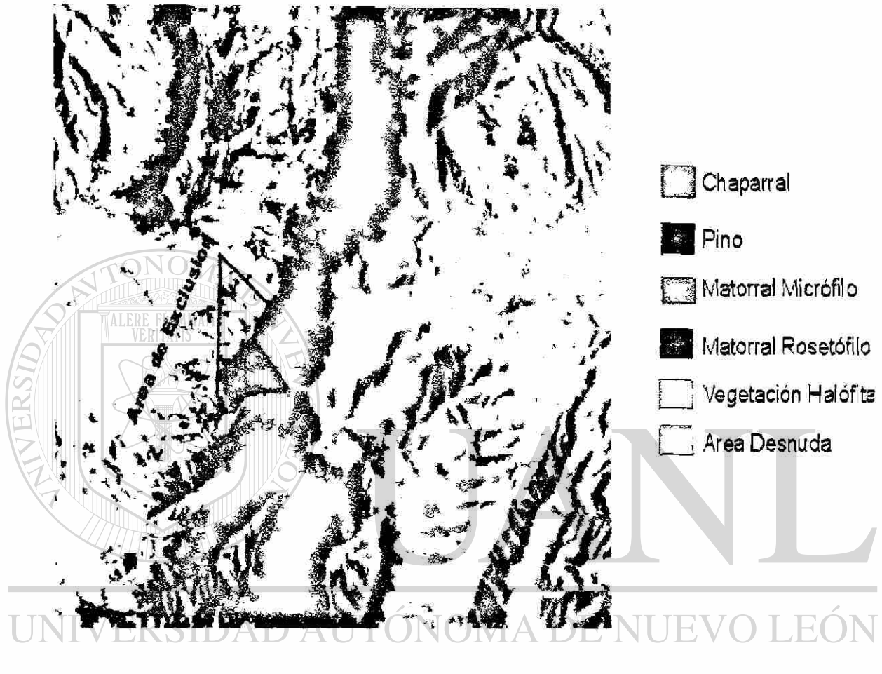
Figura 11. Mapa clasificado con seis tipos de cubierta en la exclusión del rancho "El Tigre".
