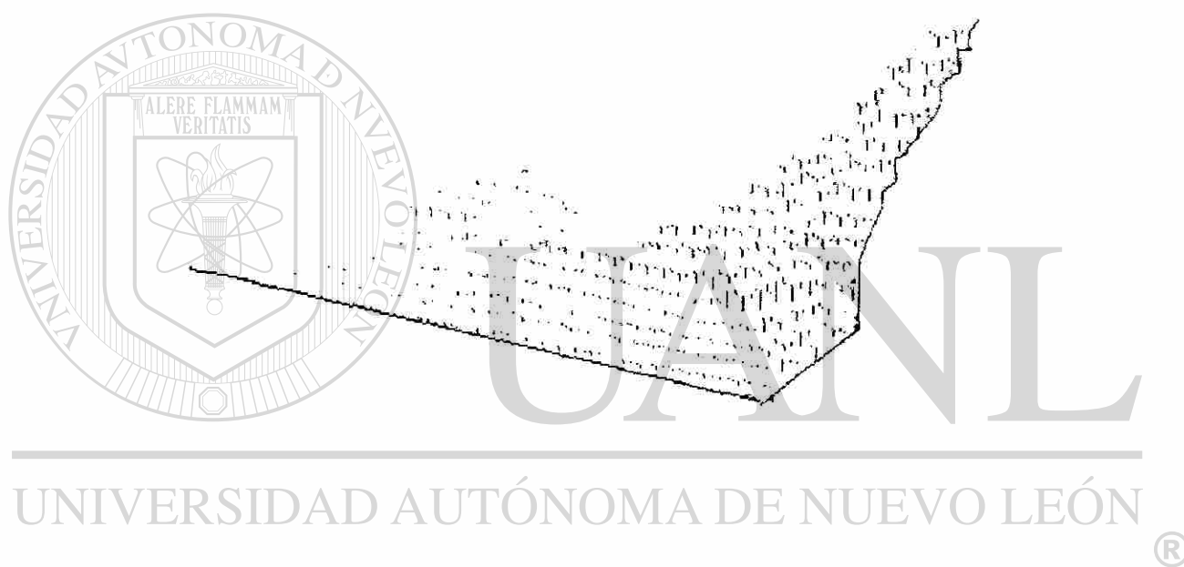
DIRECCIÓN GENERAL DE BIBLIOTECAS Figura 14. Caracterización de los rasgos topográficos del área de estudio mediante un modelo digital de elevación
