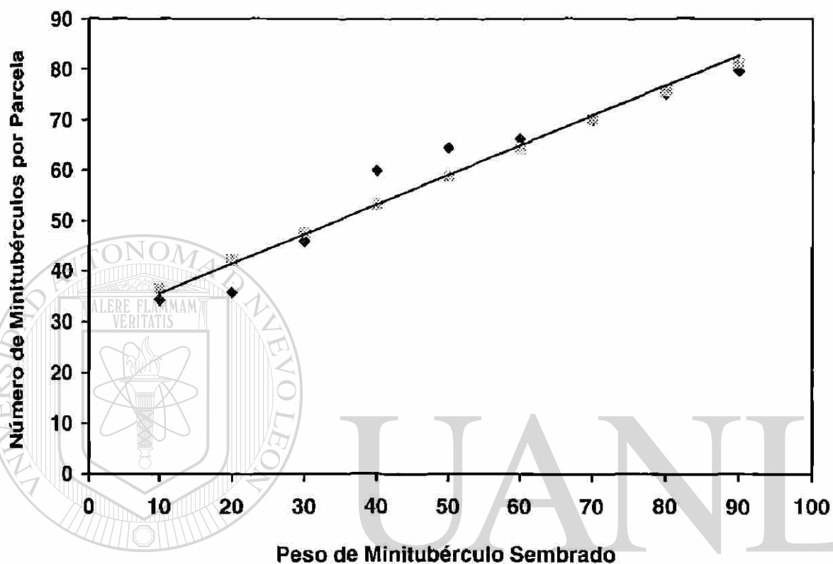
Figura 1. Relación lineal entre el peso de los minitubérculos de segunda generación sembrados (X) y la producción de minitubérculos de tercera generación por parcela (Y), var. Atlantic, O-I 98/99, FAUANL-HBR, Marín N.L.
