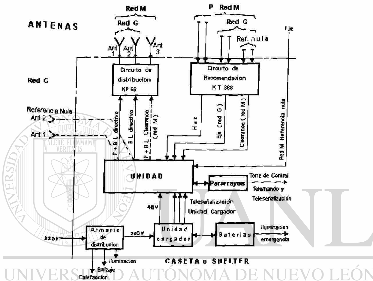
Fig 8.22 Uniones Eléctricas
