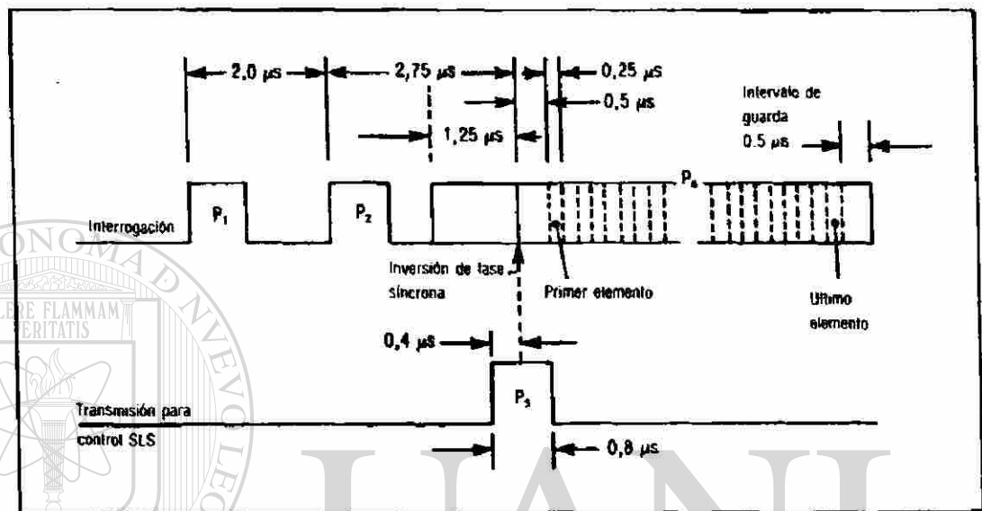
Fig. A.3 Secuencia de pulsos de interrogación en modo S
