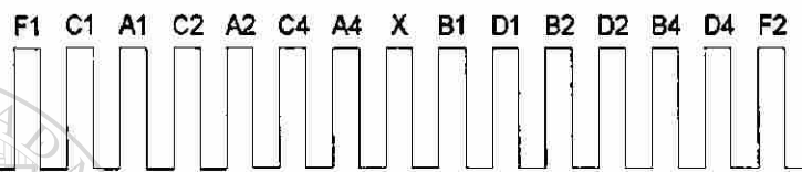
Fig. 4.4 Respuesta del transponder
