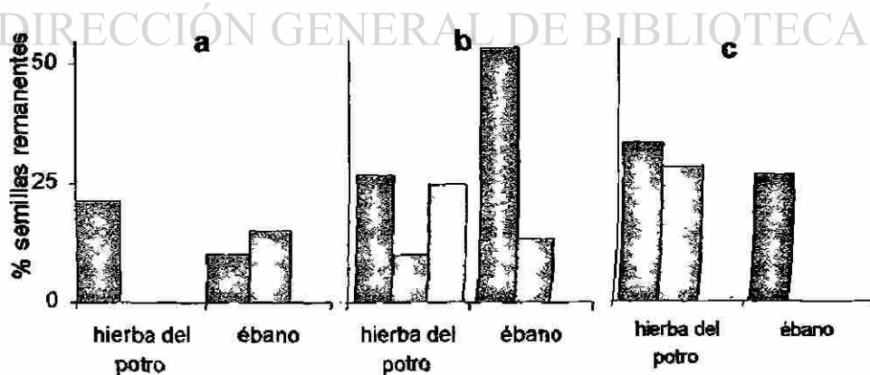
Fig. 3.13. Porcentaje de semillas remanentes, dispersión explosiva a) junio, b) noviembre, c) abril ■ aislado ■ borde □ inmerso
