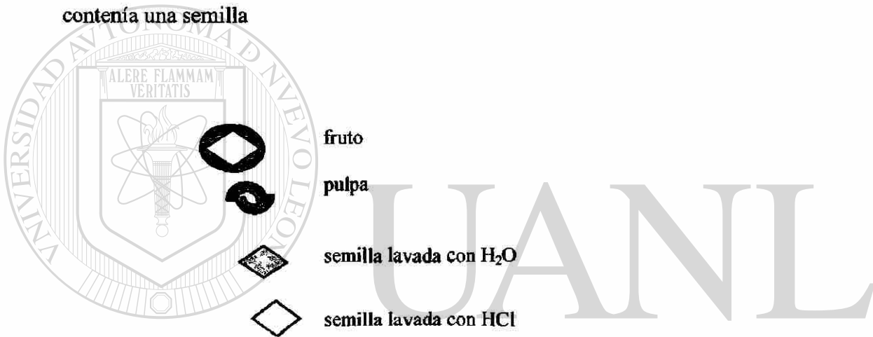
Fig. 3.1 Tratamiento a las especies dispersadas por vertebrados.
