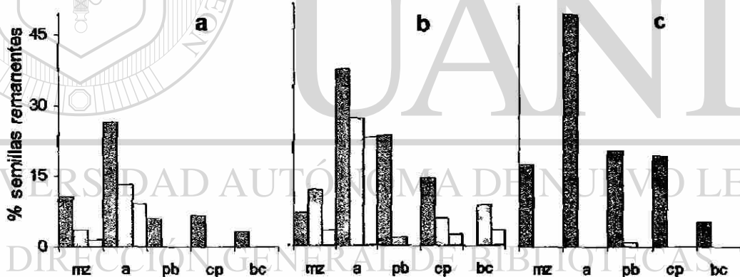
Fig. 3.11. Porcentaje de semillas remanentes, dispersión por vertebrados a) junio, b) noviembre; c) abril. mz= mezquite; a= anacahuita, pb= palo blanco; cp= chapote prieto; bc= barreta china. ■ aislado ■ borde □ inmerso
