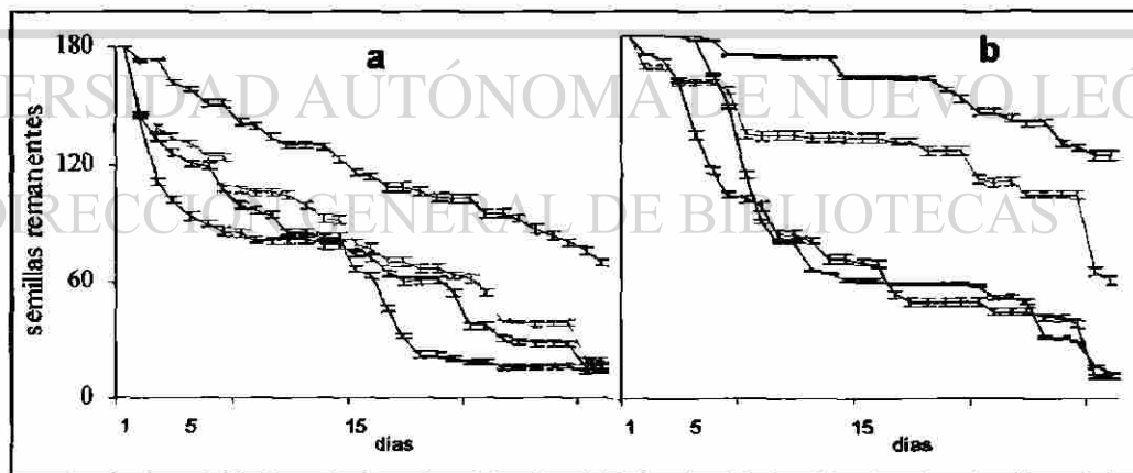
Fig. 3.3 Partes remanentes de fruto de anacahuita (promedio \pm intervalo de confianza \alpha=0.05 ; n=18 ), a) junio 98, b) noviembre 98.
