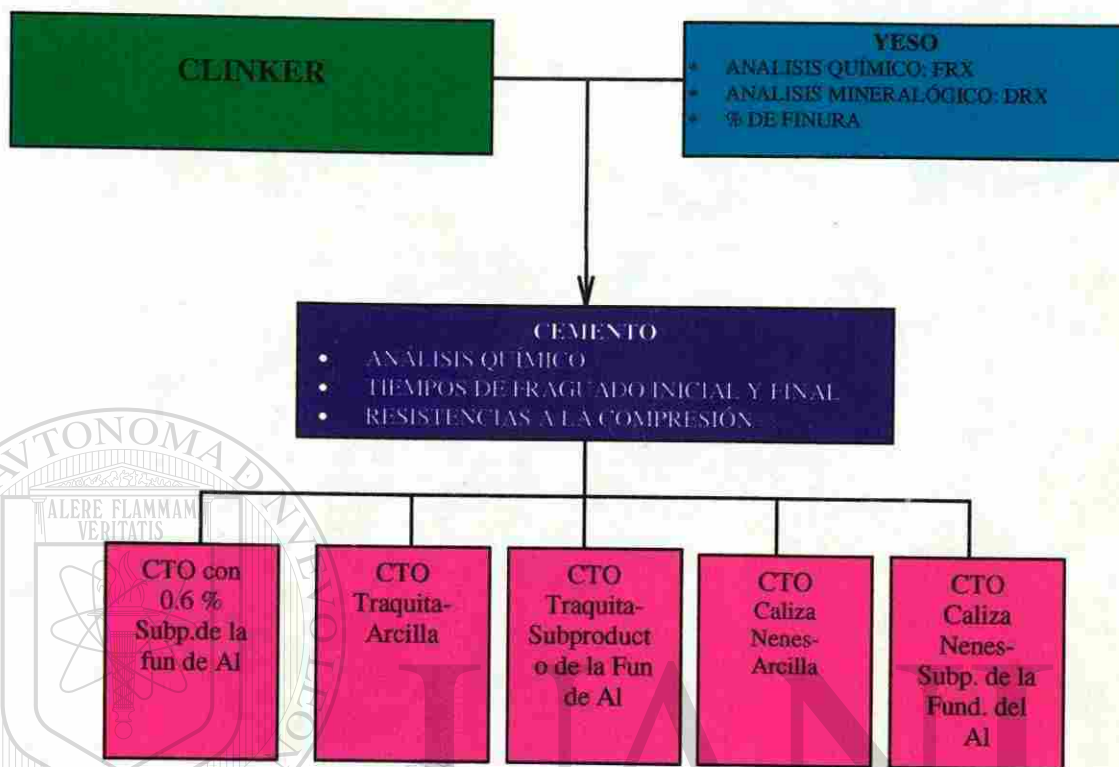
Figura III.9 Esquema de la preparación del cemento
