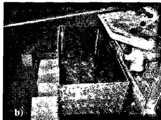
Figura III.8 a) Horno Semi-industrial, b) Clinker sinterizado a 1450 C y enfriado rápidamente
