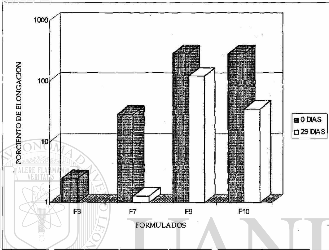
FIG. 11- PORCIENTO DE ELONGACION PROMEDIO PARA LOS DISTINTOS FORMULADOS ANTES Y DESPUES DEL TRATAMIENTO EN COMPOSTA.
