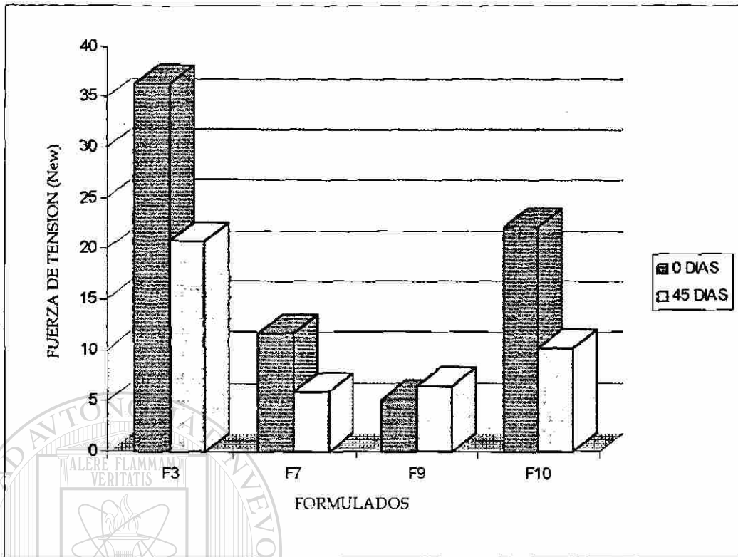
FIG. 9.- FUERZA DE TENSION PROMEDIO PARA EL TOTAL DE FORMULADOS ANTES Y DESPUES DEL TRATAMIENTO EN AGUA.
