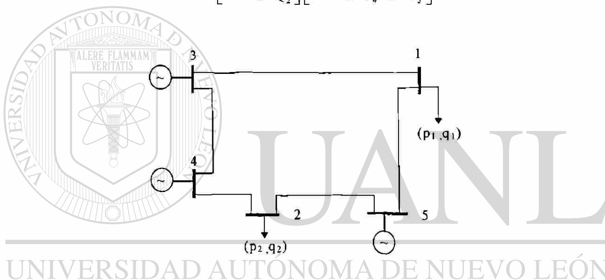
Fig. 2.7. Sistema de potencia de cinco nodos.
