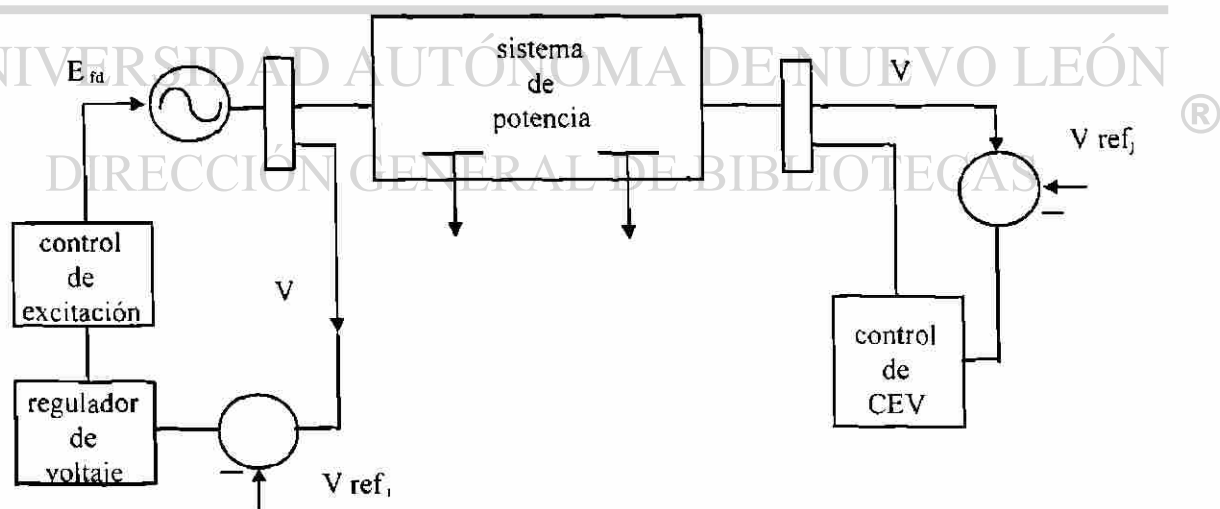
Fig. 2.4. Control de voltaje primario.
